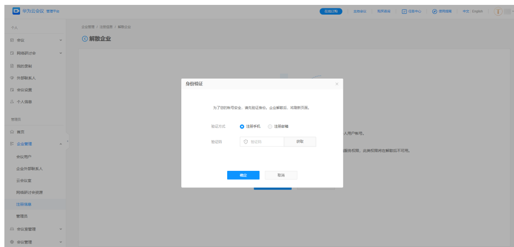
图 8-3 填写验证码
