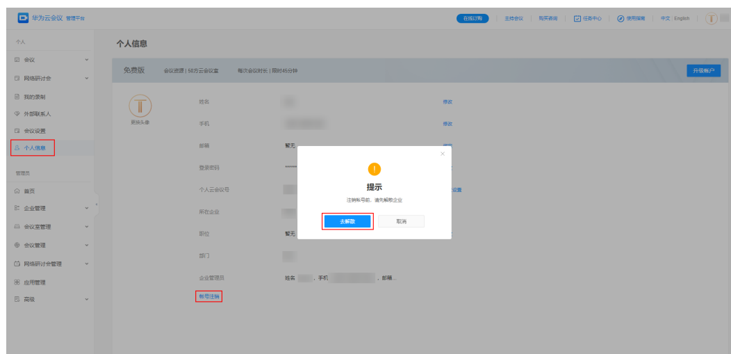
图 8-2 解散企业
