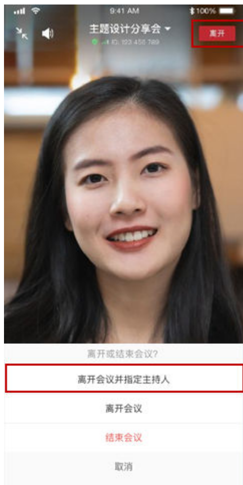
图 5-10 退出会议
