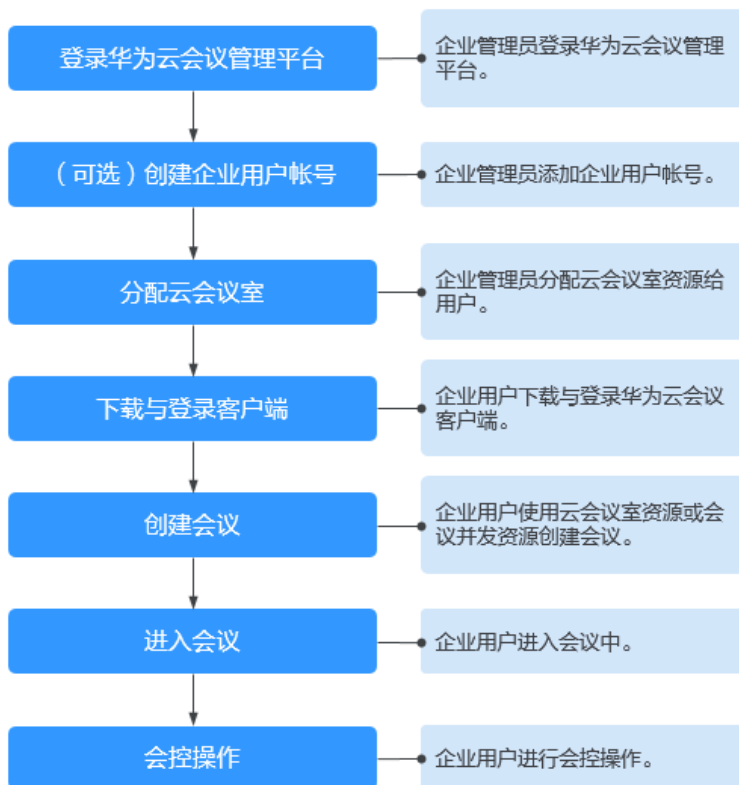
图 7-1 使用流程
