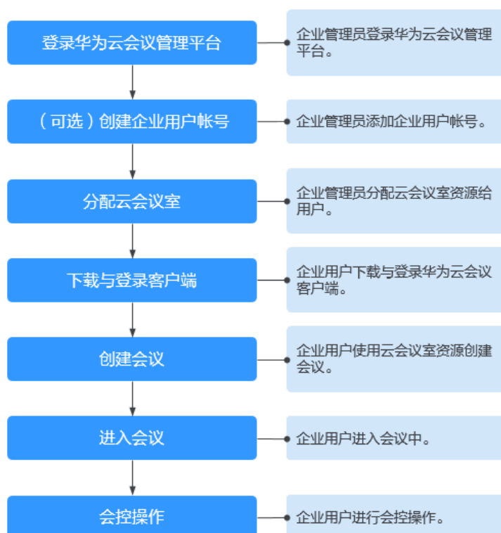
图 7-19 使用流程
