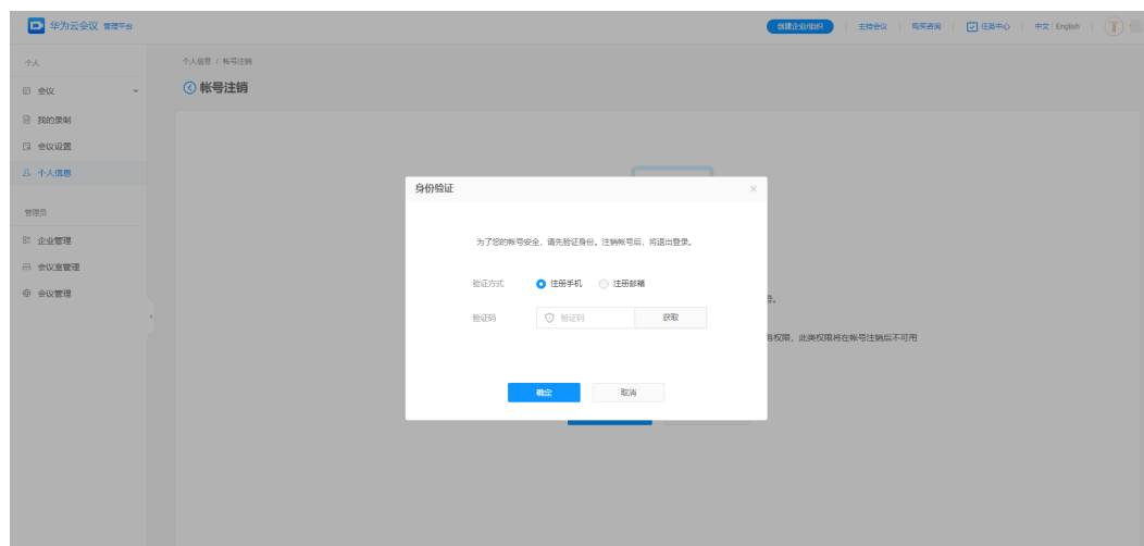
图 8-9 填写验证码
