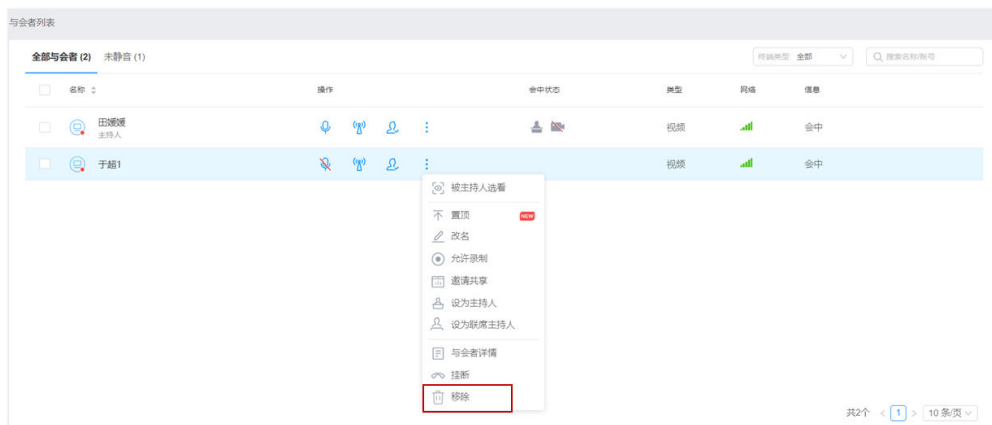
图 7-16 删除与会者
