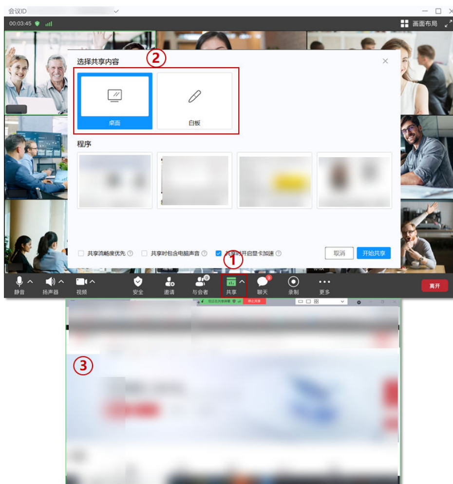
图 7-33 会议共享
