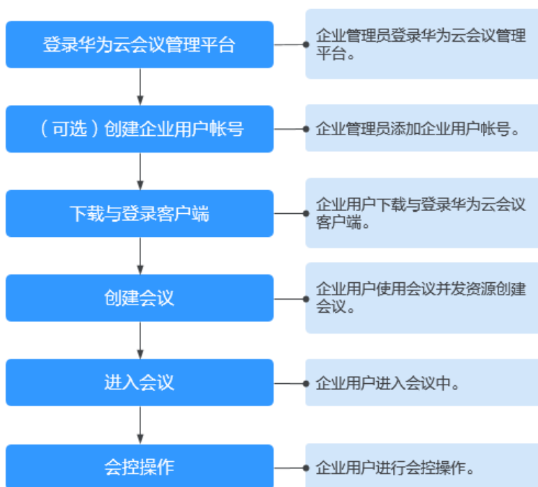
图 7-34 使用流程
