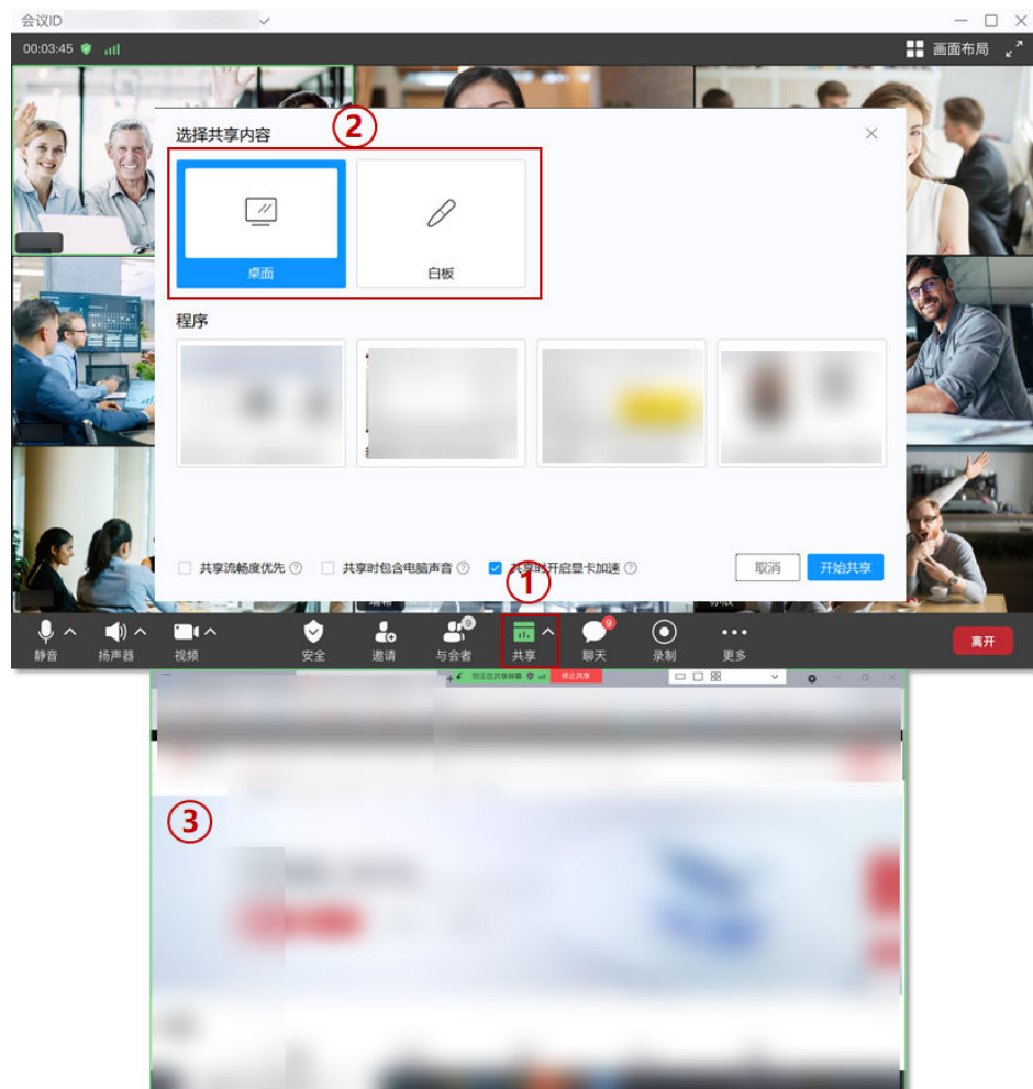
图 7-45 会议共享
