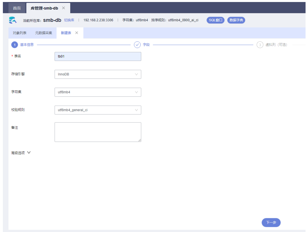
图 1-12 新建表
