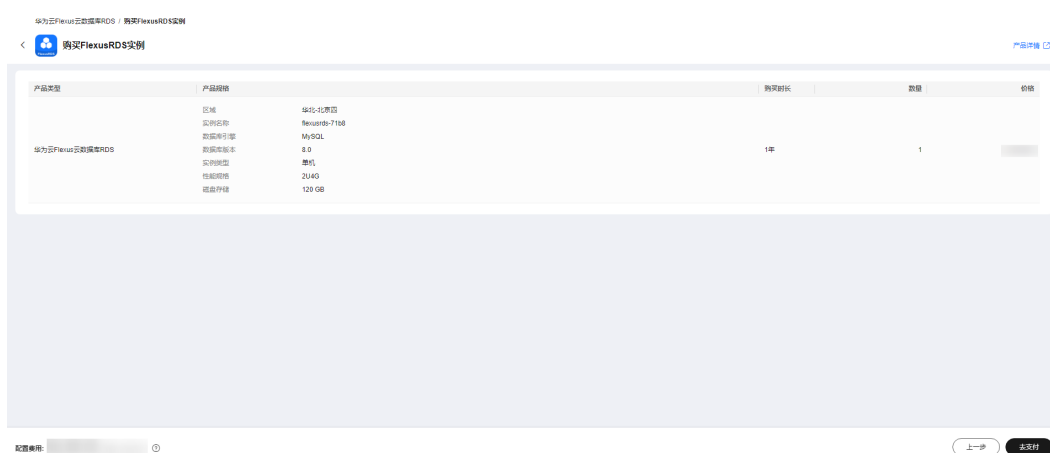
图 1-3 订单确认
