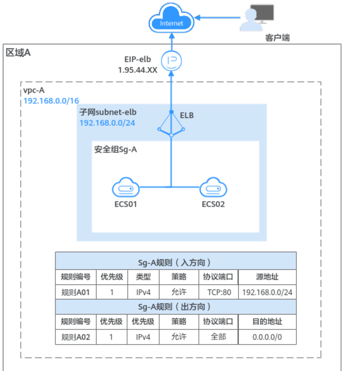
图 1-1 单个应用负载分发架构图
