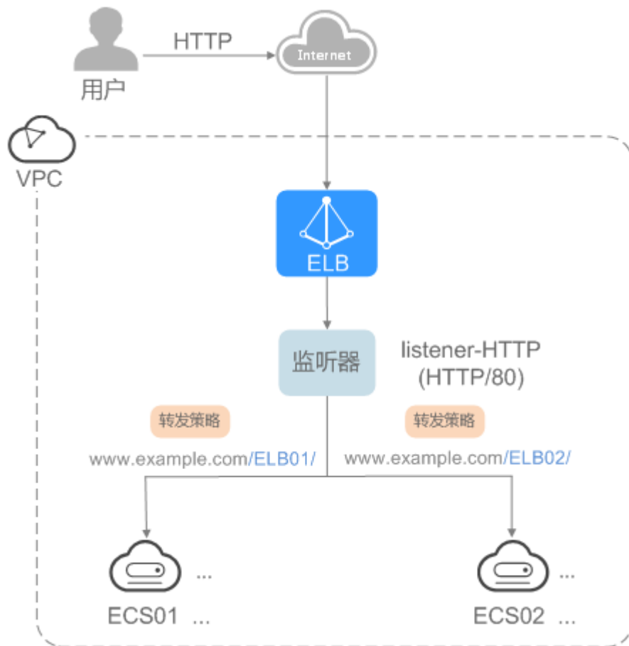
图 2-10 数据转发示意图
