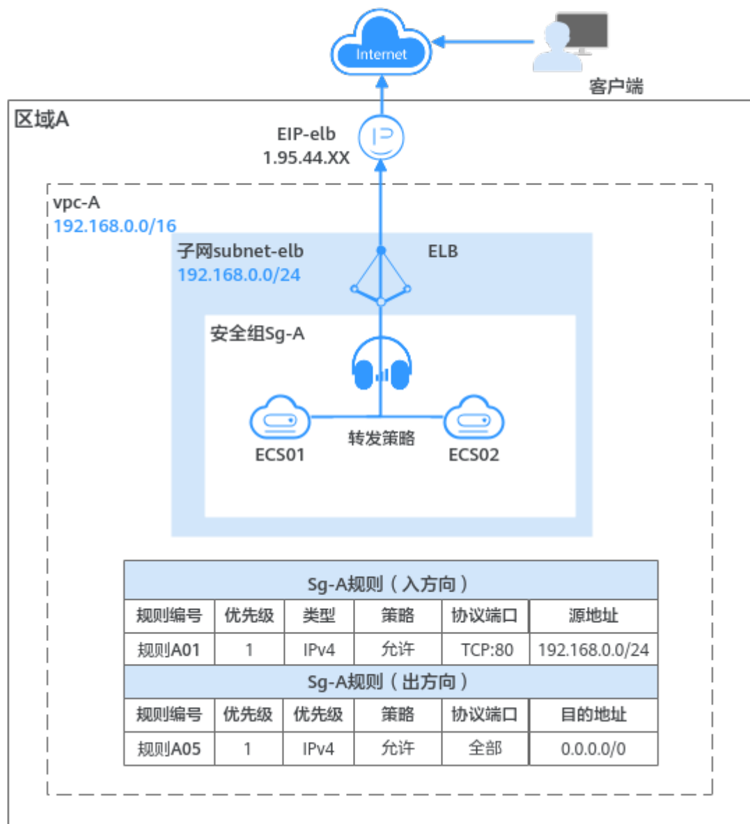
图 2-1 两个应用负载分发架构图
