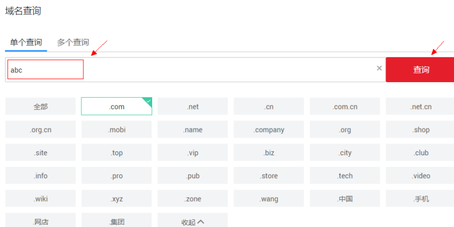
图 3-1 域名查询
