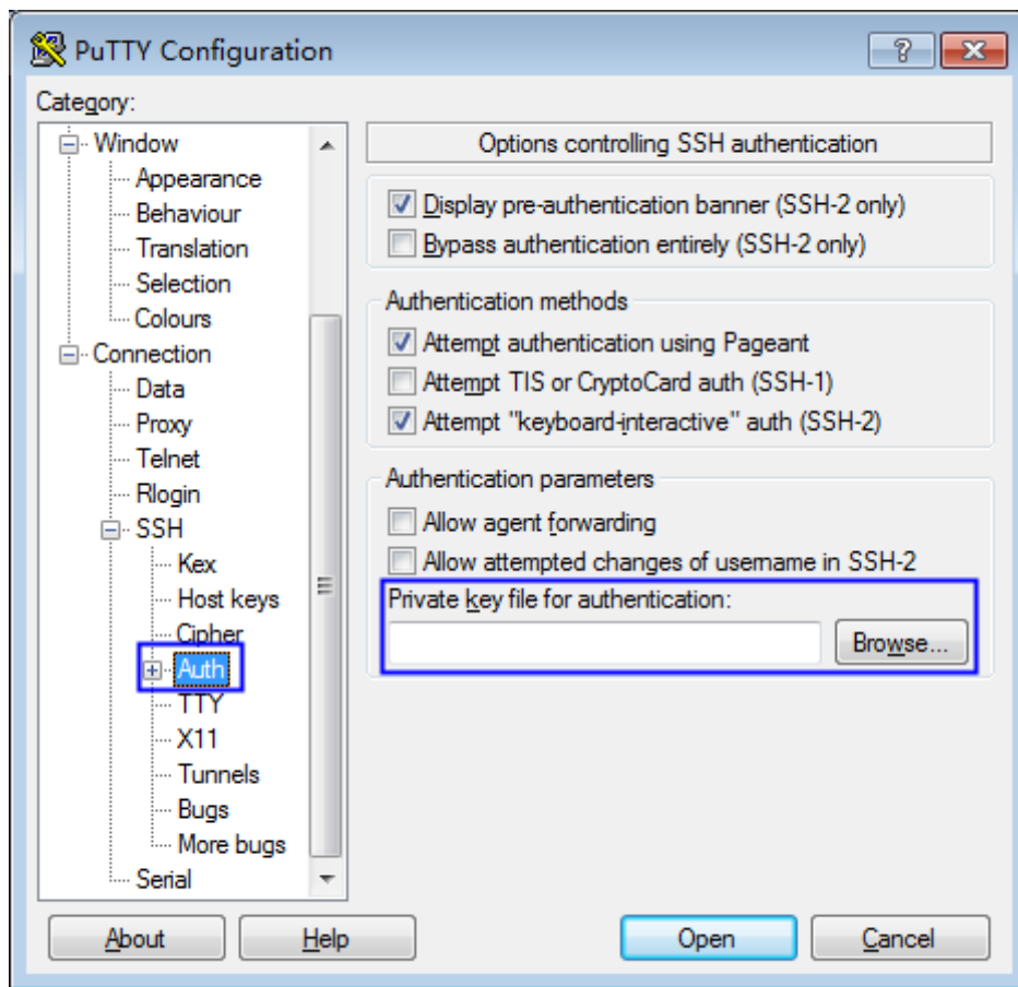
图 3-5 上传私钥文件
