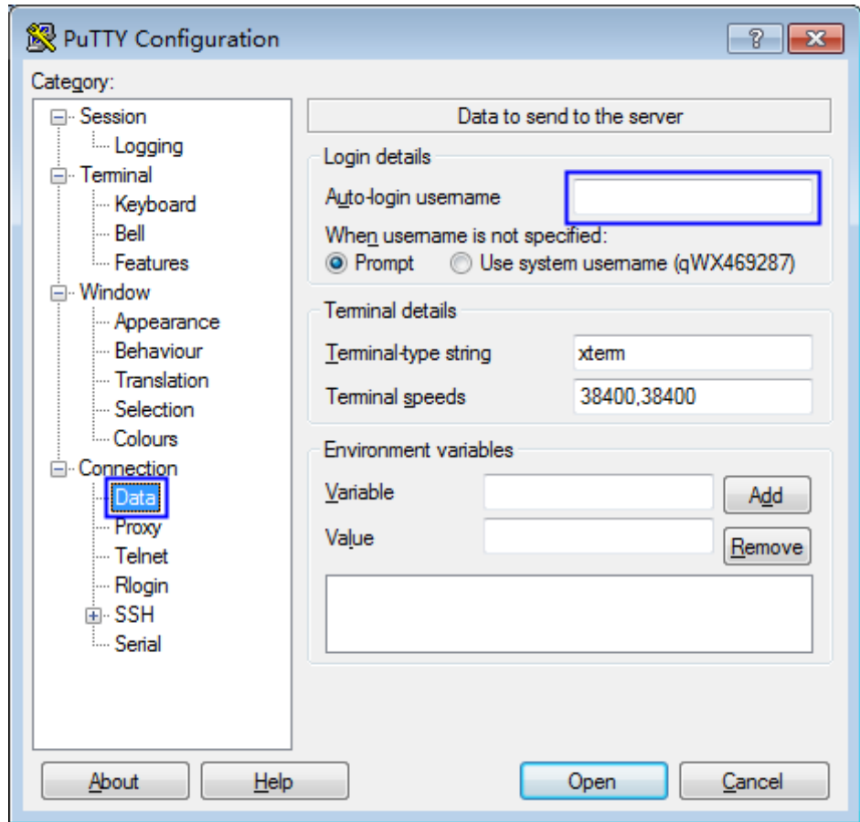
图 3-4 镜像用户名
