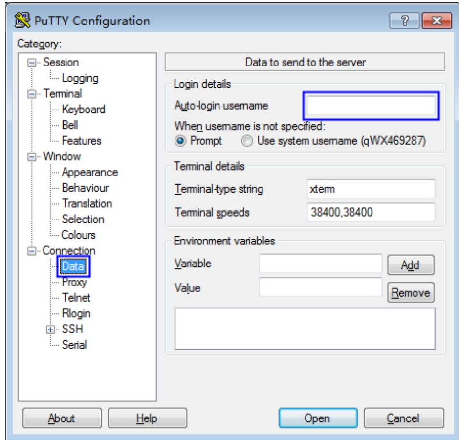
图 5-2 镜像用户名
