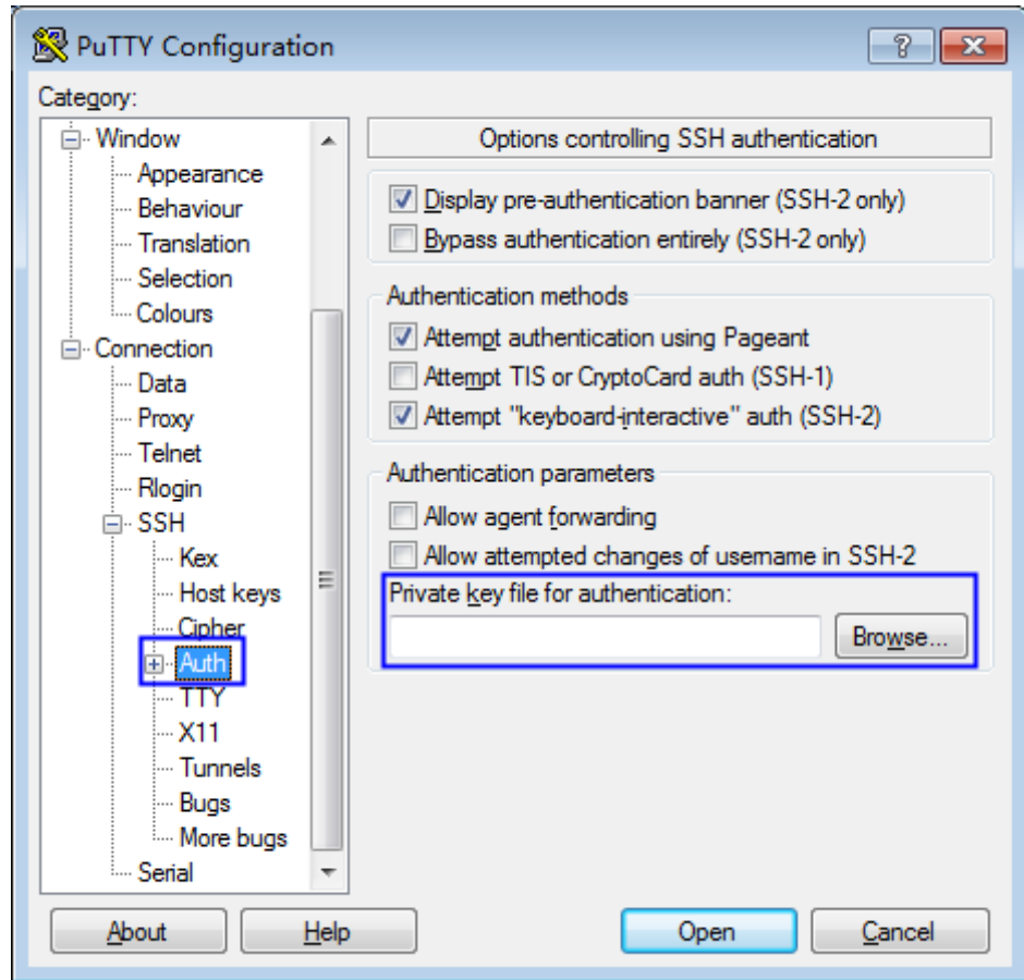
图 5-4 上传私钥文件
