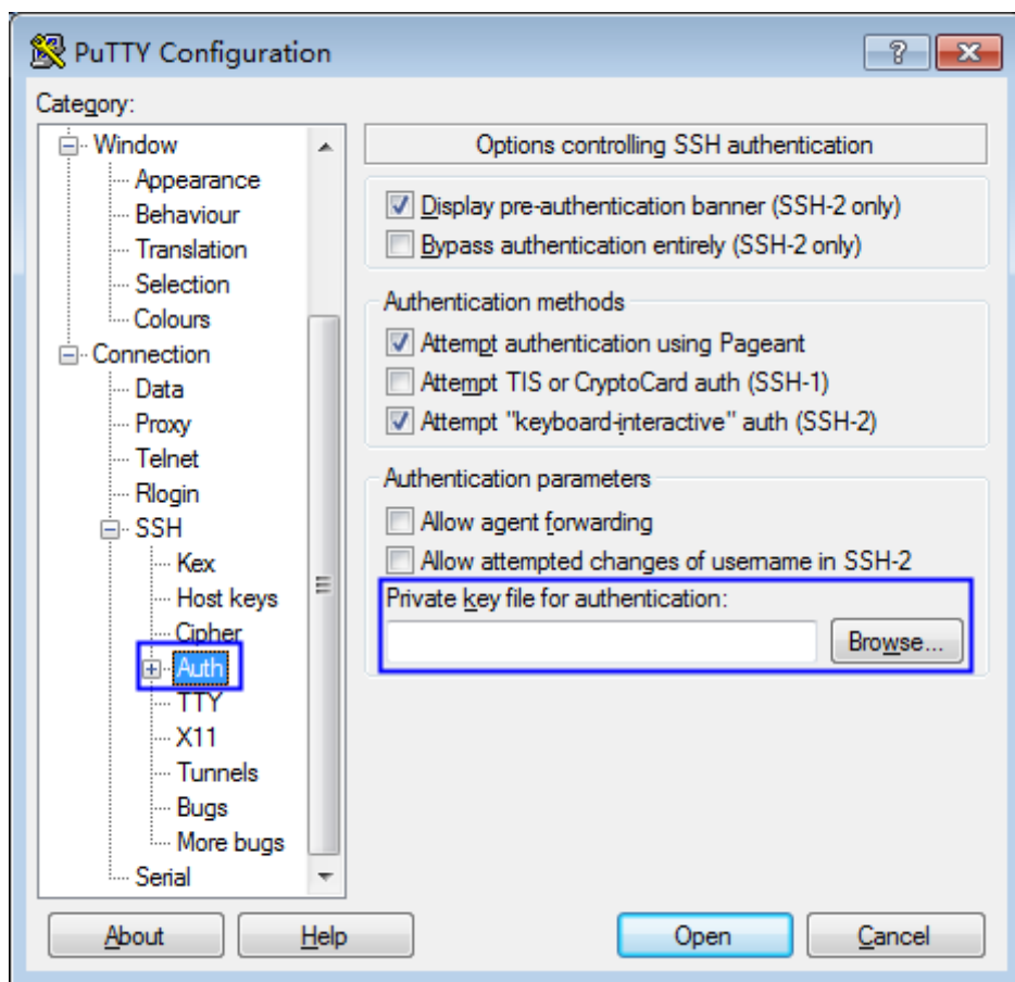
图 5-3 上传私钥文件
