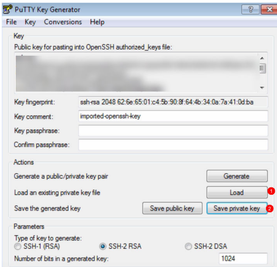
图 3-2 私钥文件格式转换
