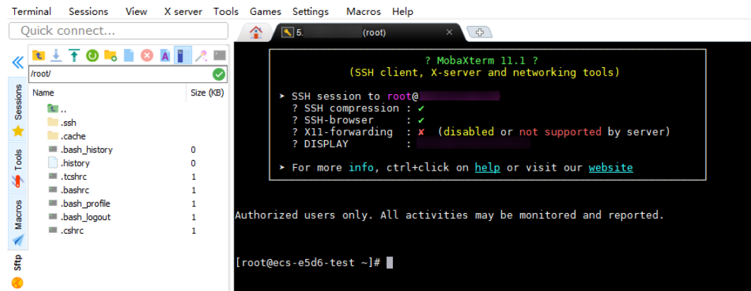
图 2-17 登录成功
