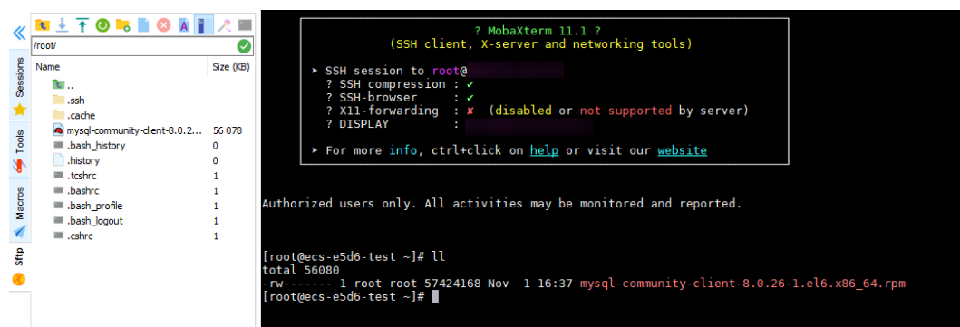
图 2-21 上传成功
