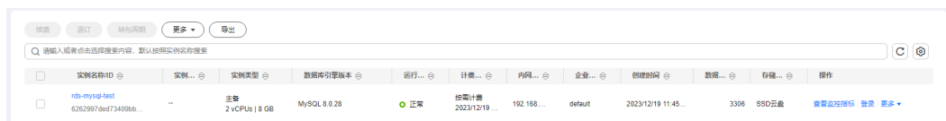
图 2-6 购买成功
