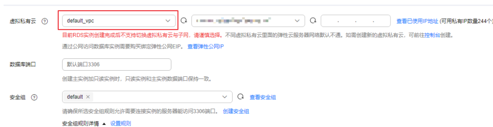
图 3-5 选择网络
