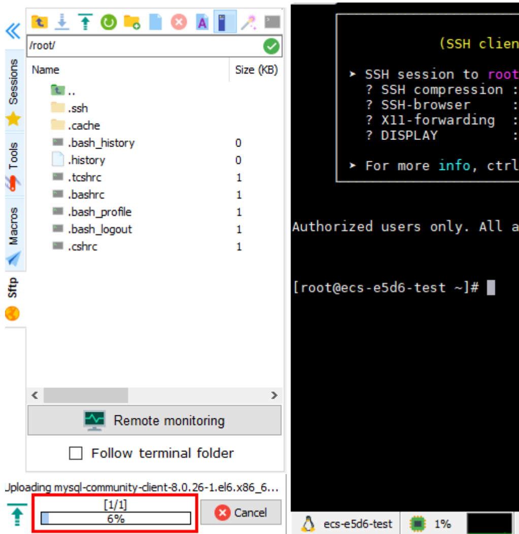
图 2-20 上传客户端
