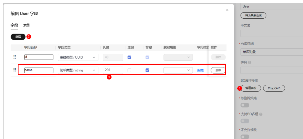
图 2-12 新增 name 字段
