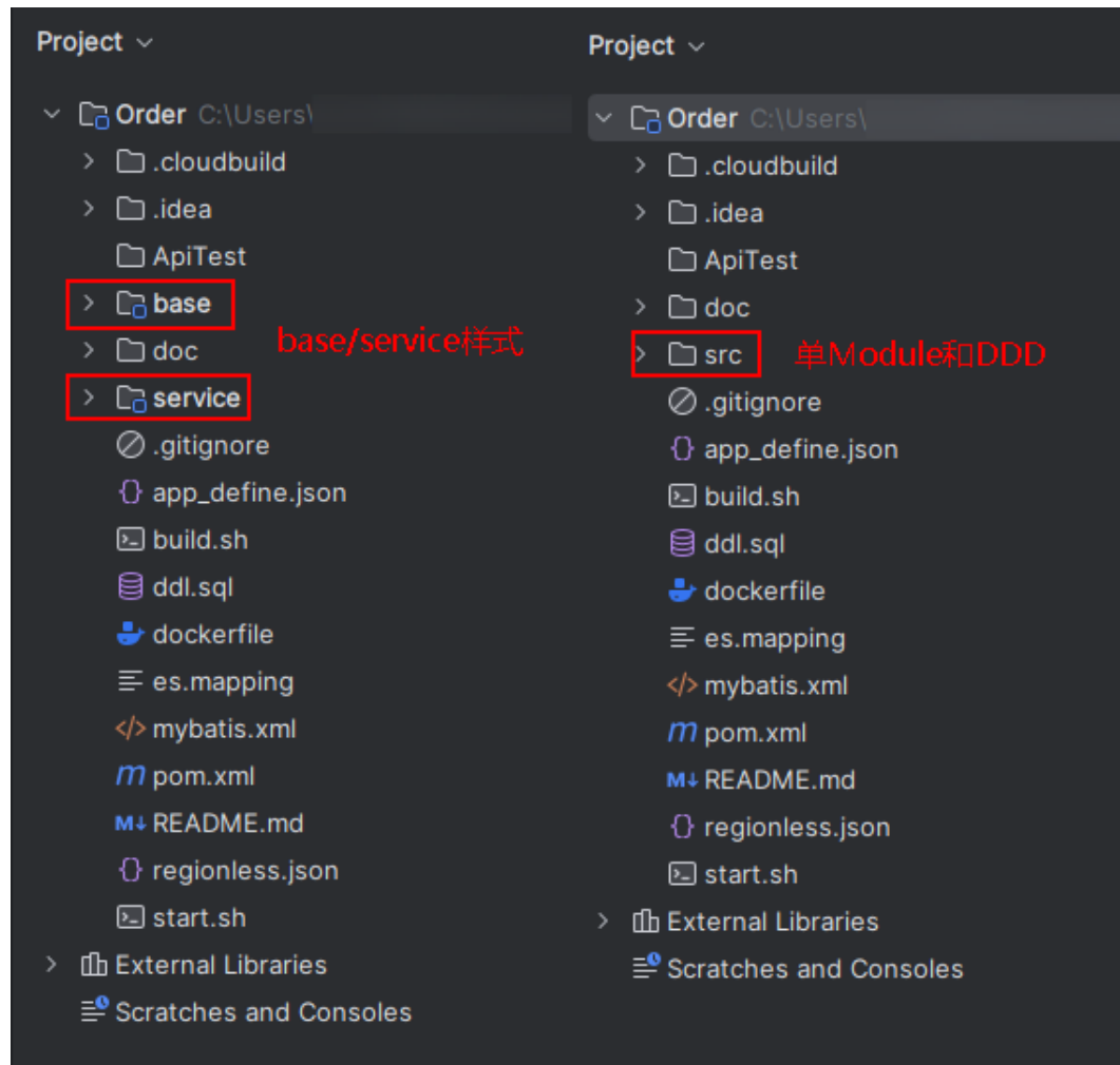
图 2-21 工程目录不同类型设置效果
