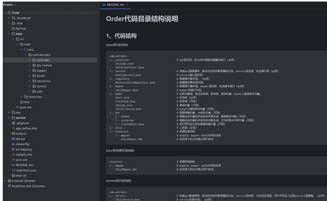
图 2-19 代码目录结构说明
