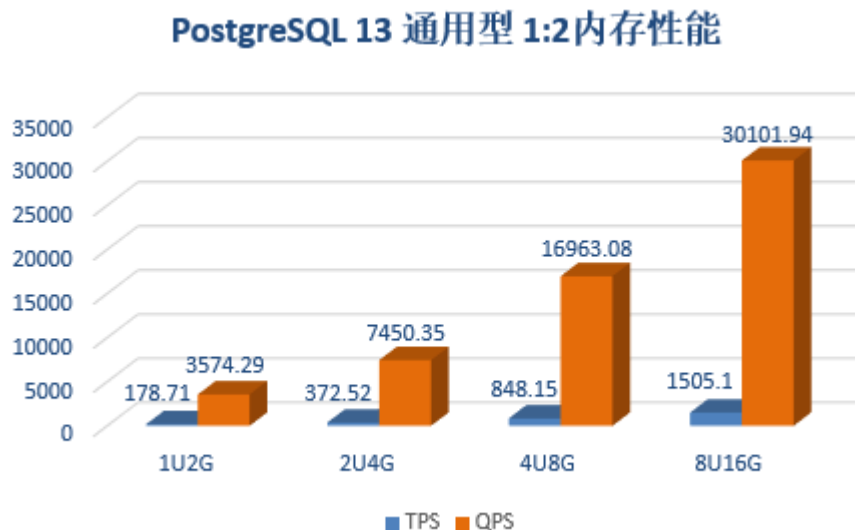
图 3-1 CPU:内存=1:2
