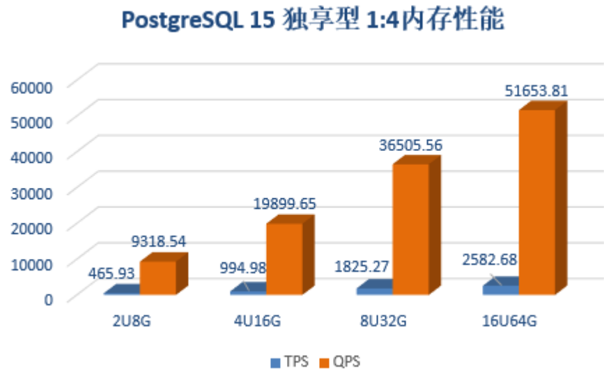
图 5-4 CPU:内存=1:4
