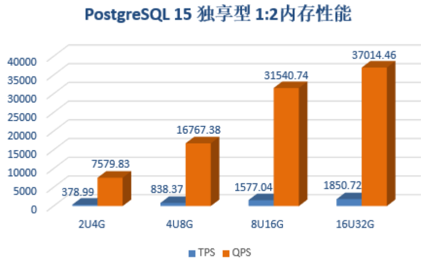
图 5-3 CPU:内存=1:2
