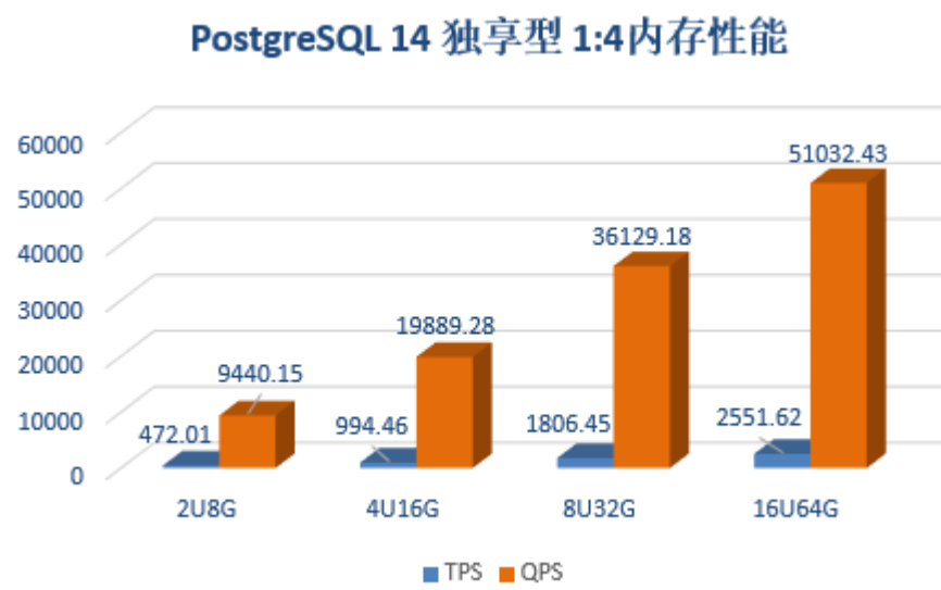
图 4-4 CPU:内存=1:4
