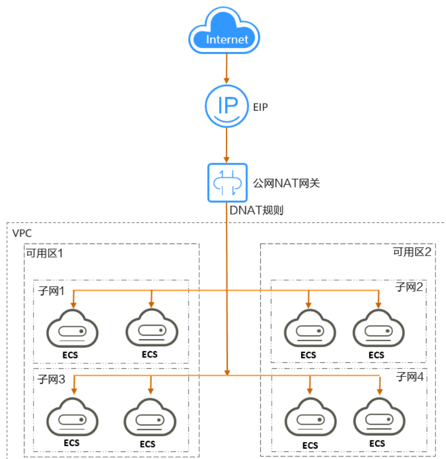
图 1-2 DNAT 架构图
