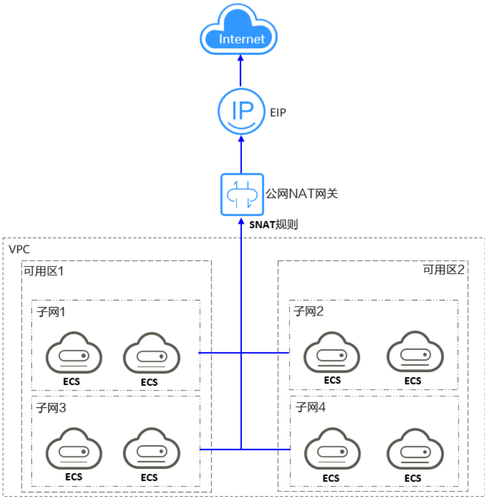
图 1-1 SNAT 架构图
