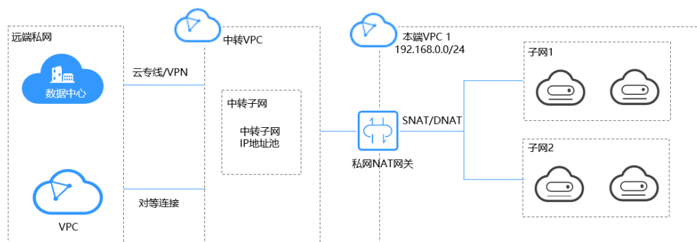
图 1-3 私网 NAT 网关
