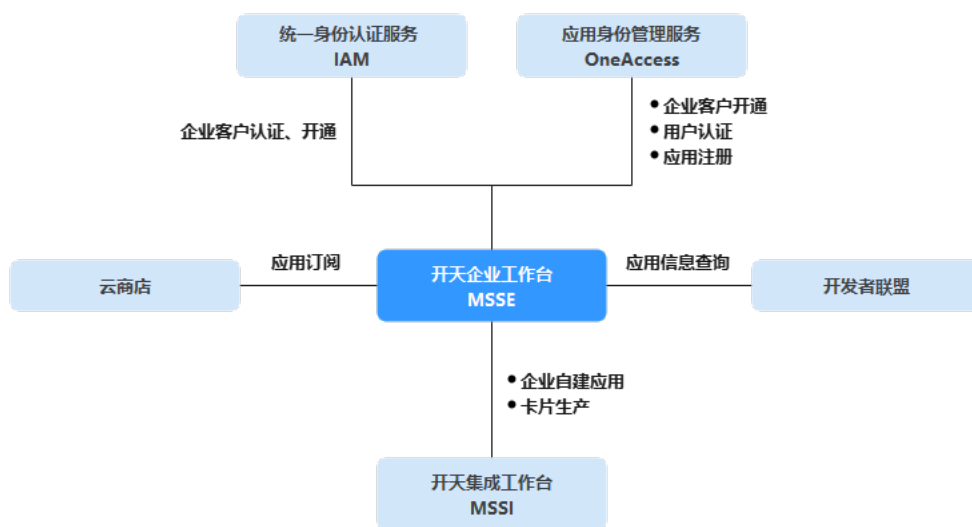
图 10-1 开天企业工作台与其他服务的关系
