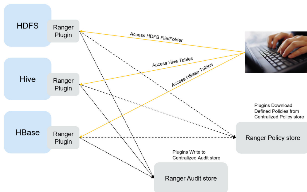
图 7-90 Ranger 与组件的关系
