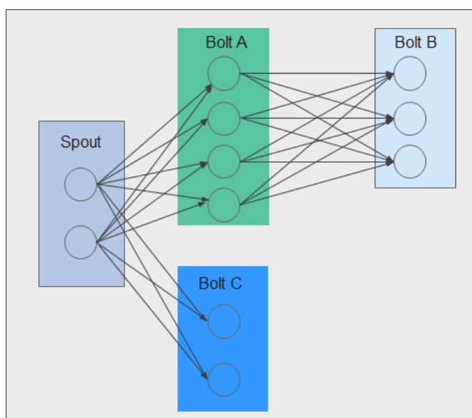
图 7-130 Topology 示意图
