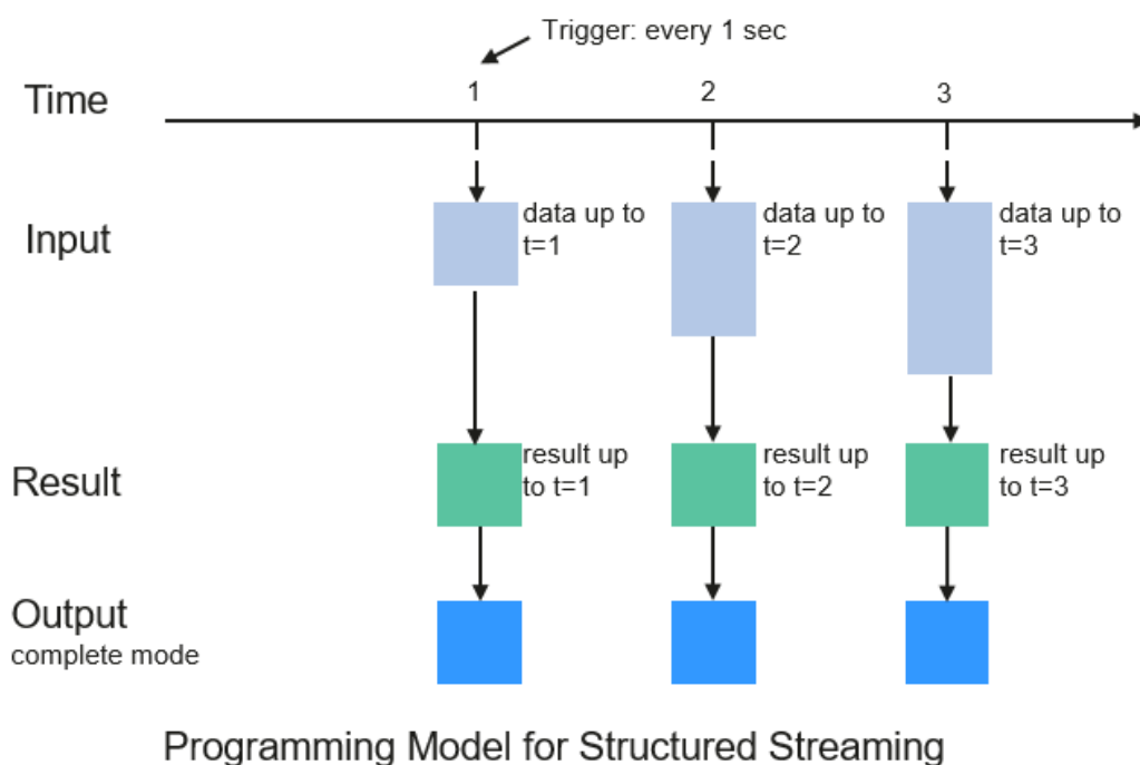
图 7-99 Structured Streaming 数据处理模型
