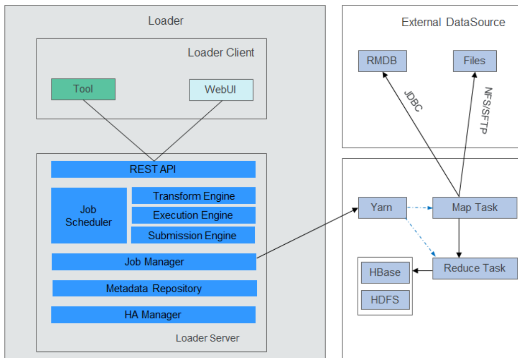
图 7-79 Loader 模型
