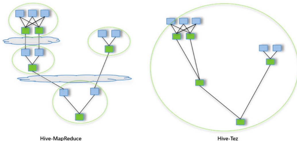
图 7-132 Hive 基于 MapReduce 提交任务和基于 Tez 提交任务流程图
