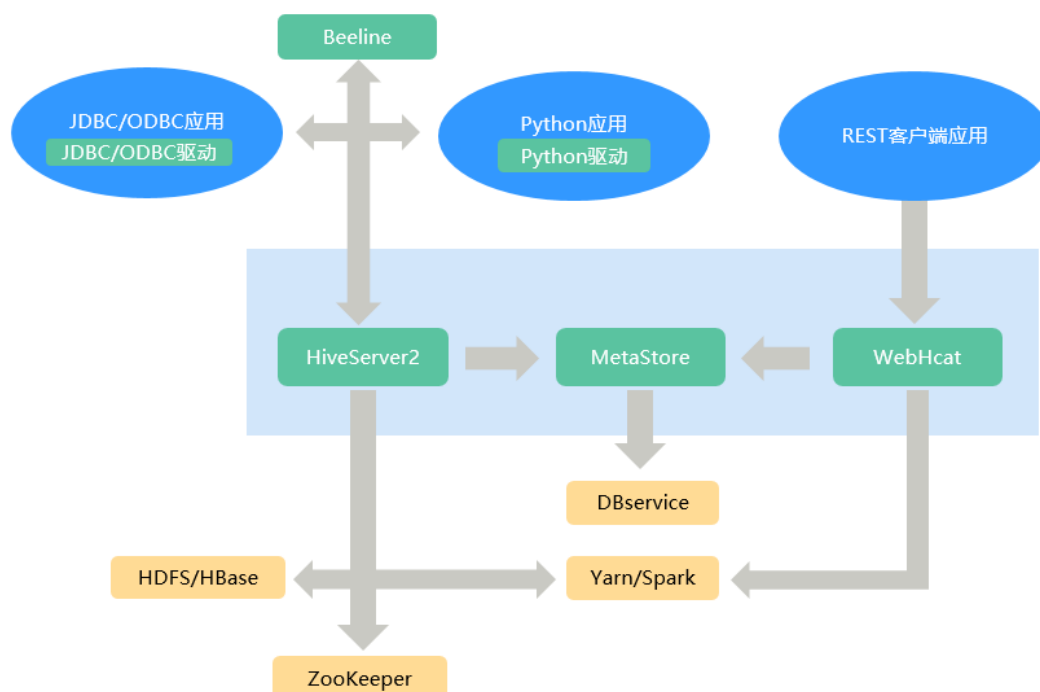
图 7-57 Hive 结构
