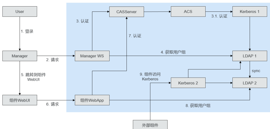
图 7-74 安全认证场景架构
