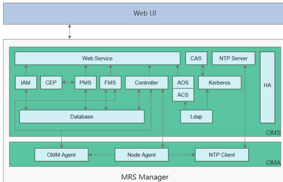
图 7-80 Manager 逻辑架构
