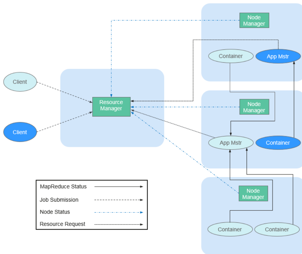
图 7-133 YARN 结构
