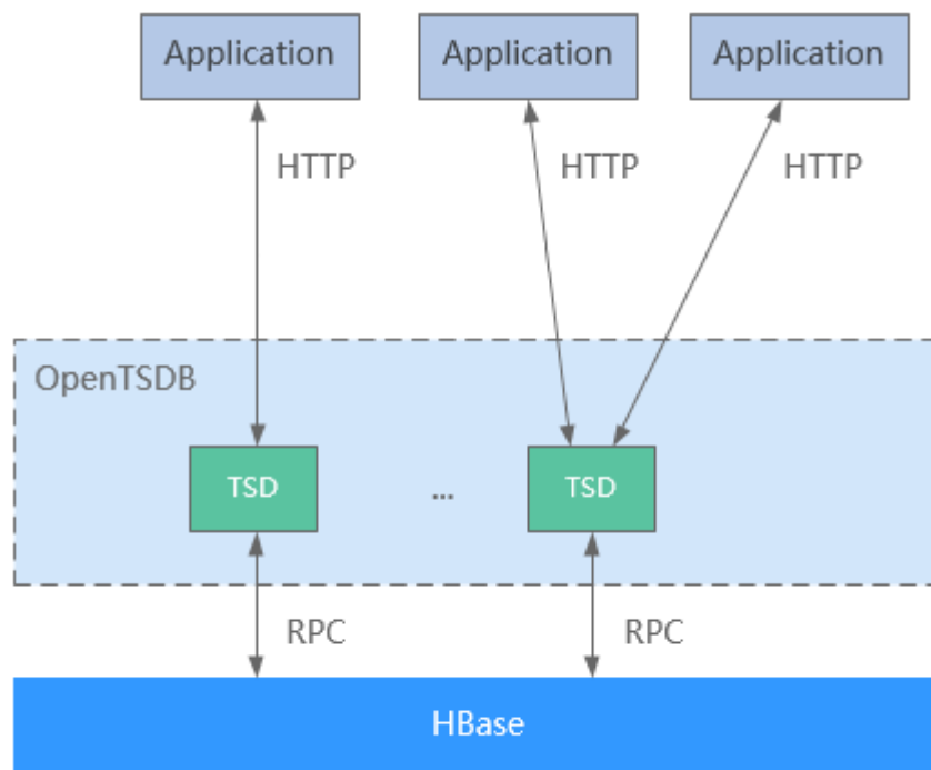
图 7-87 OpenTSDB 架构
