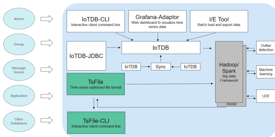
图 7-68 IoTDB 结构
