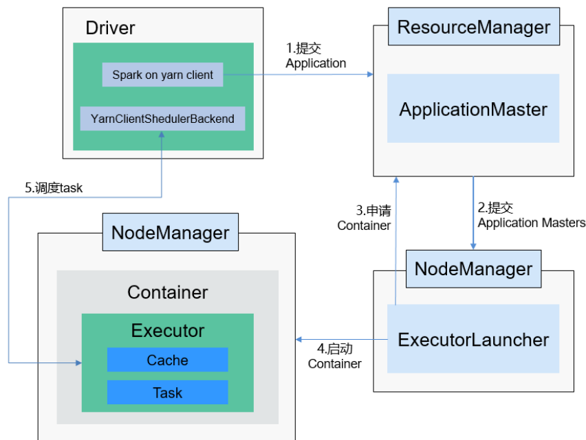
图 7-137 Spark on yarn-client 运行框架
