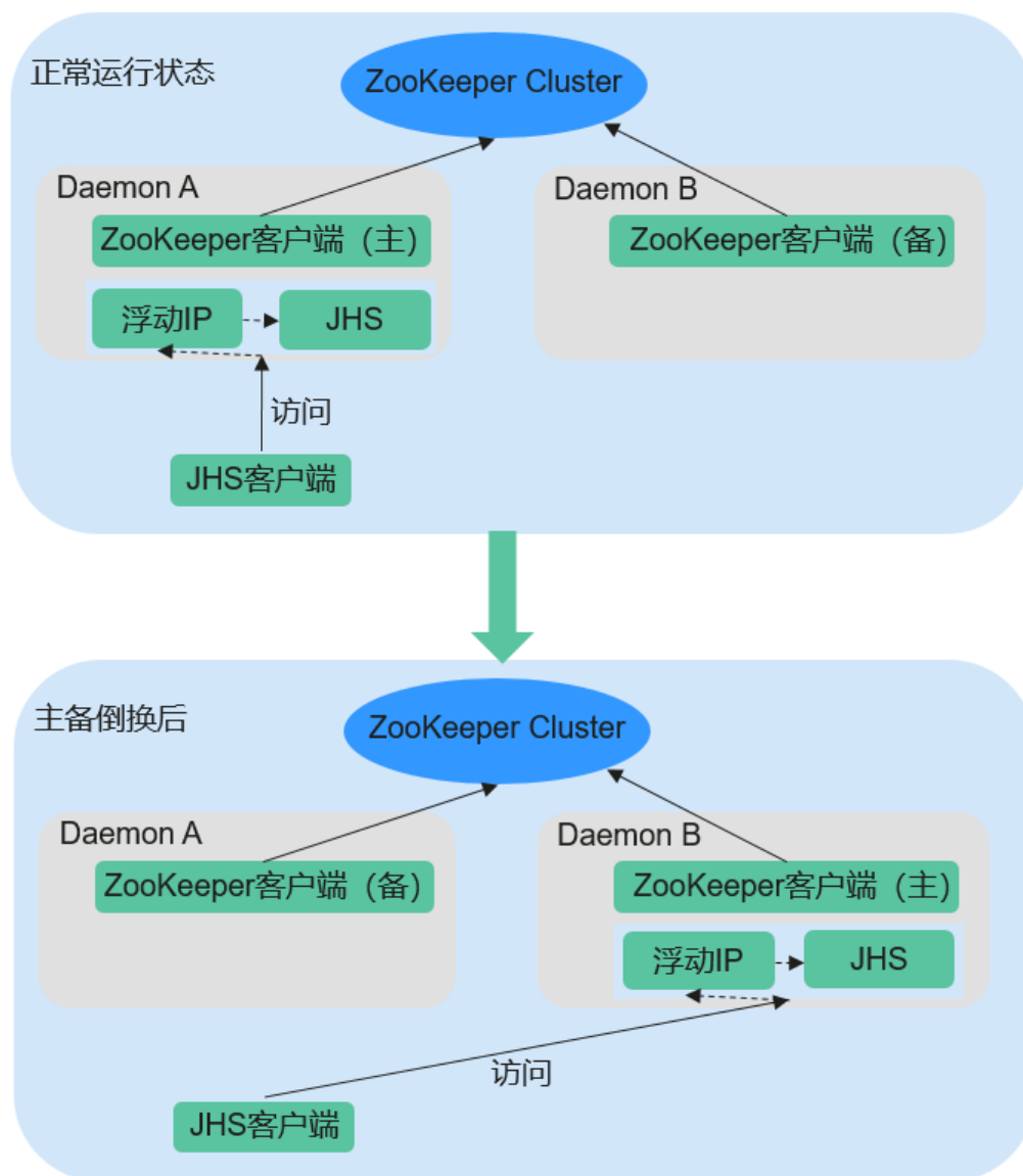
图 7-82 JobHistoryServer HA 主备倒换的状态转移过程
