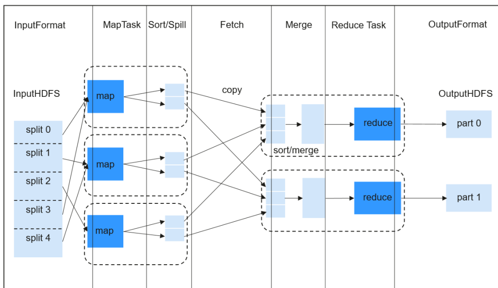
图 7-83 MapReduce 作业
