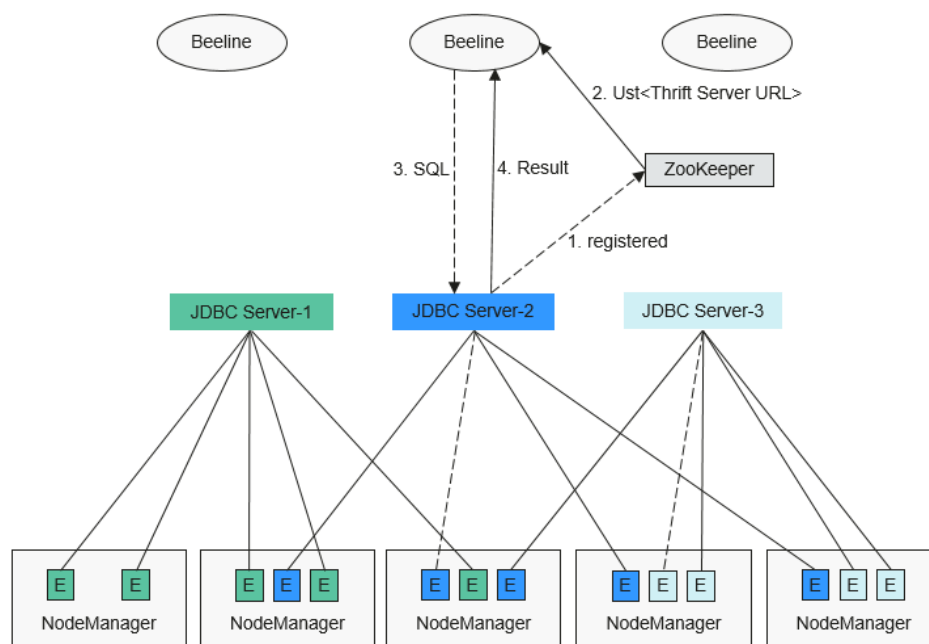
图 7-103 Spark JDBCServer HA
