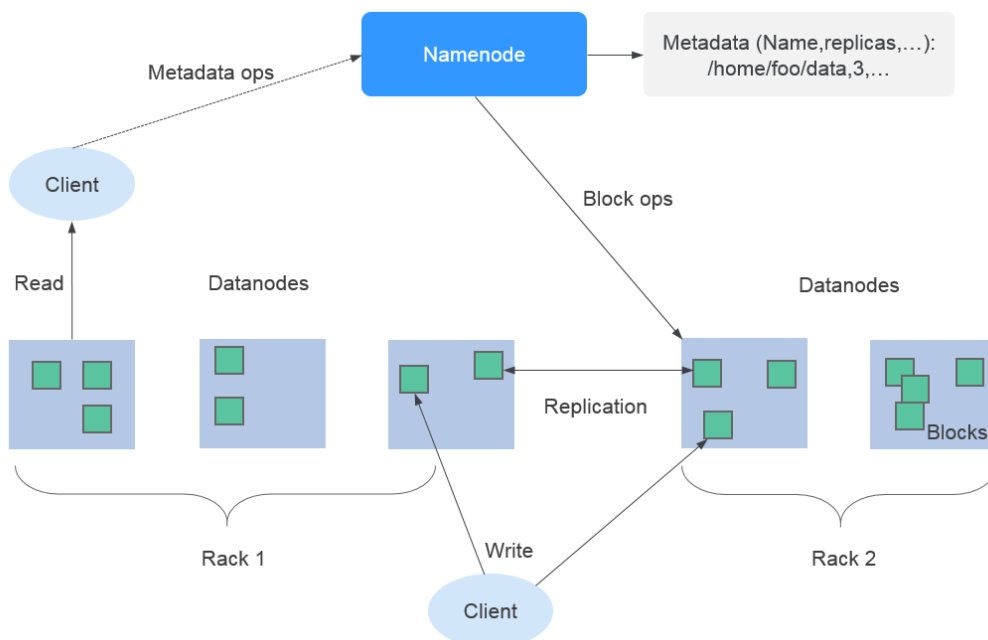
图 7-42 HDFS 架构
