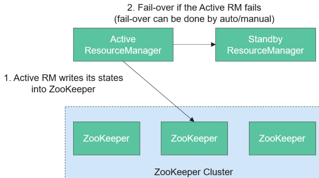
图 7-135 ResourceManager 高可用性实现架构
