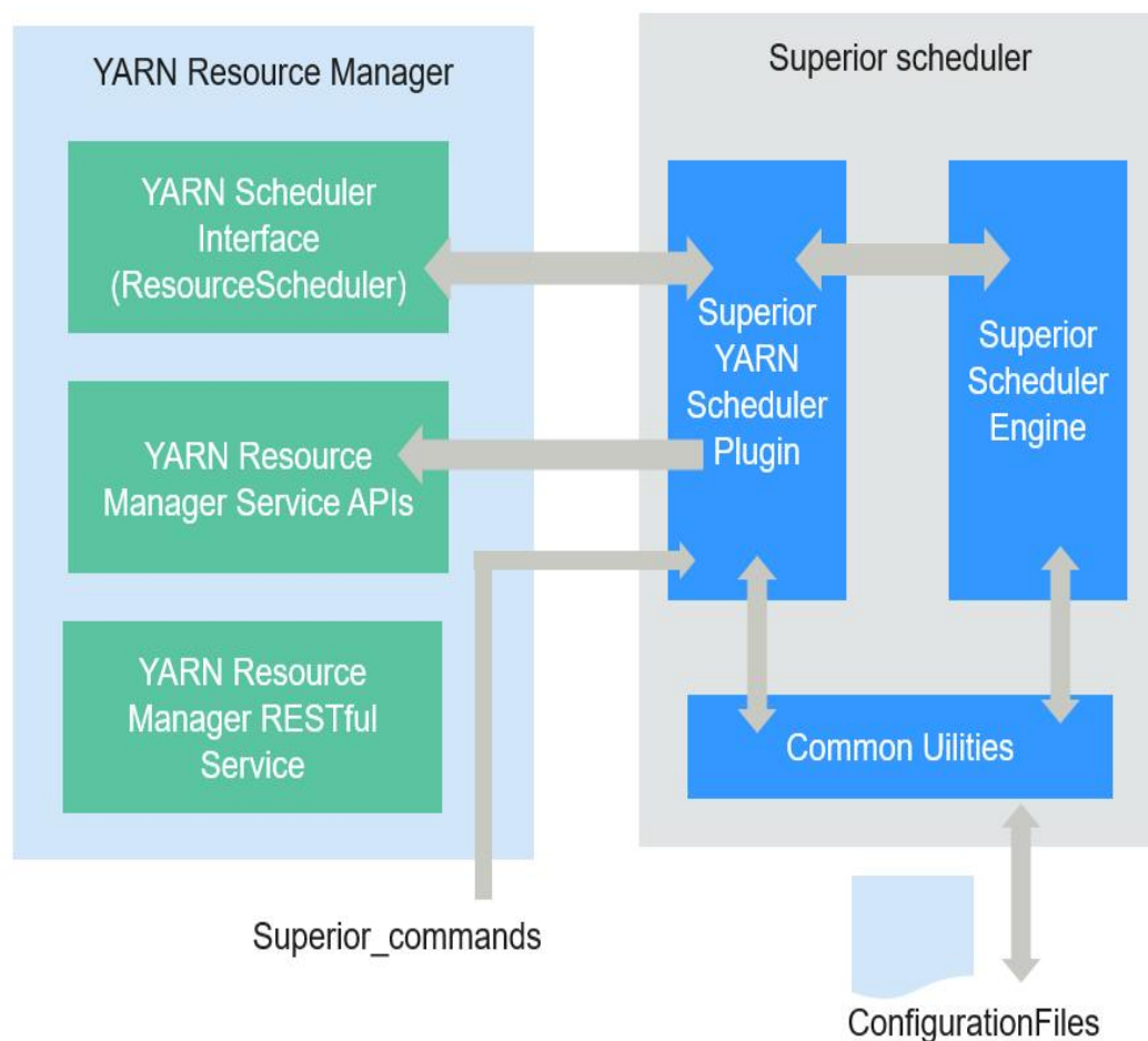
图 7-139 Superior Scheduler 内部架构
