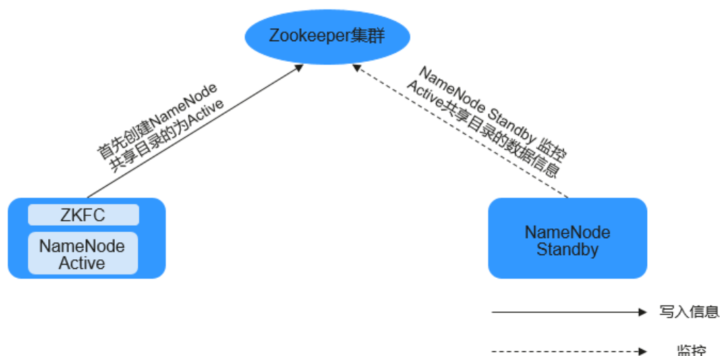
图 7-145 ZooKeeper 和 HDFS 的关系
