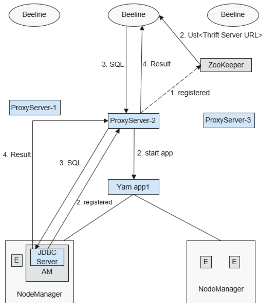
图 7-122 Spark JDBCServer 多租户
