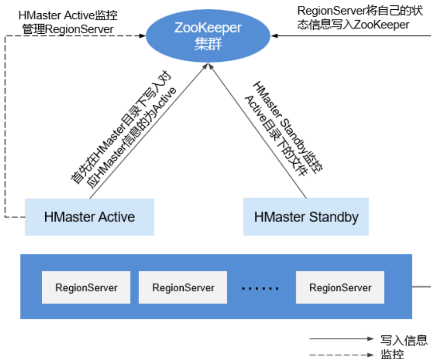
图 7-147 ZooKeeper 和 HBase 的关系
