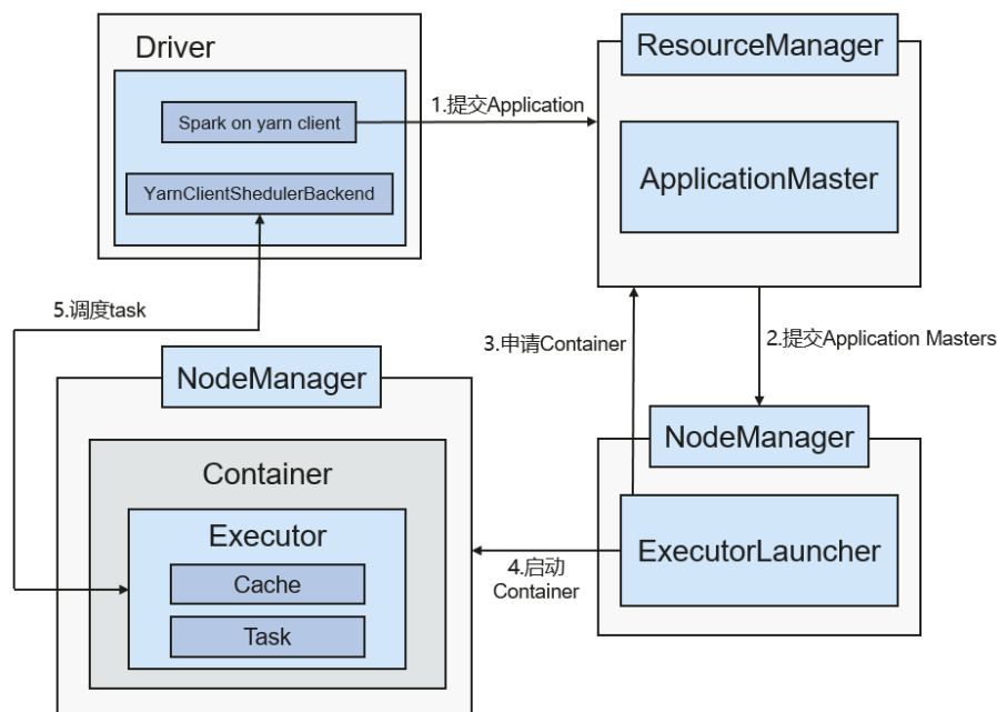
图 7-126 Spark on yarn-client 运行框架
