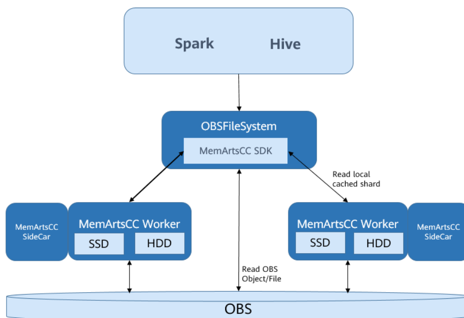
图 7-85 MemArtsCC 结构
