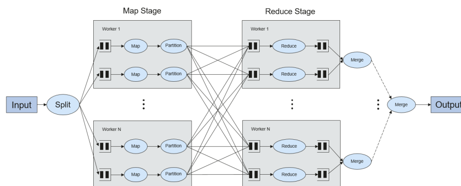
图 7-120 算法流程
