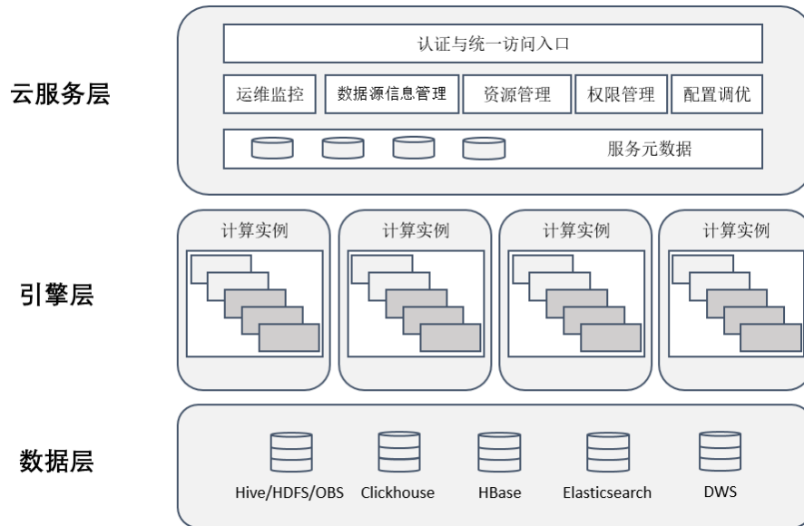
图 7-54 HetuEngine 结构图
