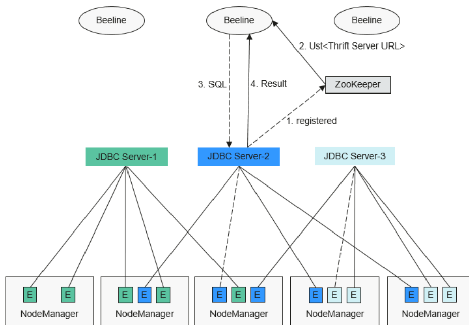
图 7-121 Spark JDBCServer HA
