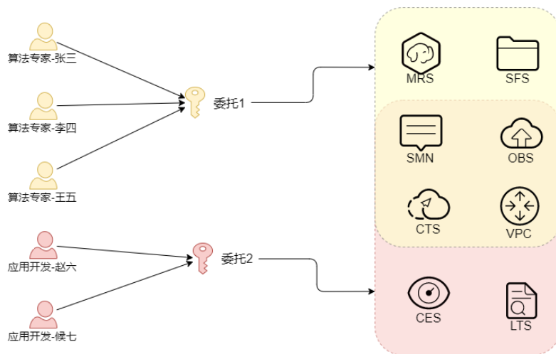
图 9-4 用户与委托对应关系
