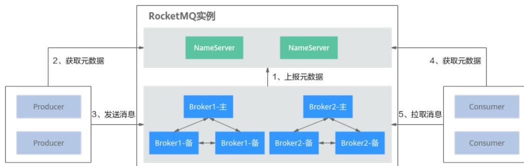
图 2-1 产品架构示意图
