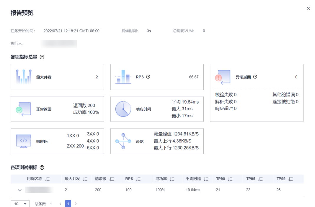
图 3-12 解决方案工作台验证中心 - 性能自动化
