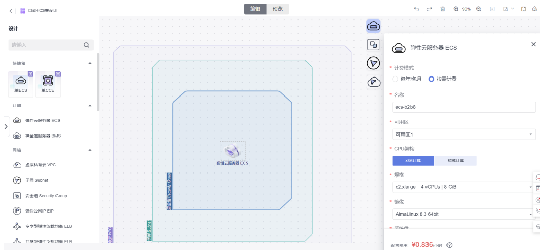
图 3-6 自动化部署
