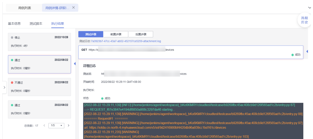
图 3-11 API 自动化
