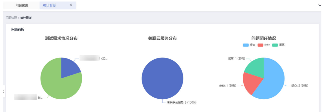
图 3-14 问题管理
