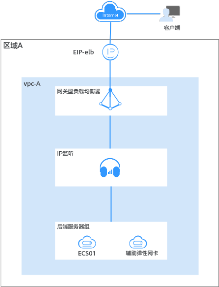
图 2-1 GWLB 组成
