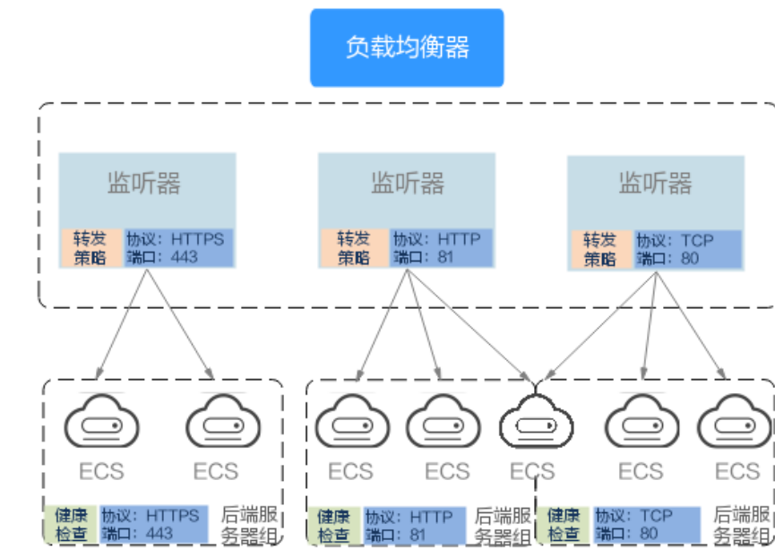
图 1-2 弹性负载均衡组件图
