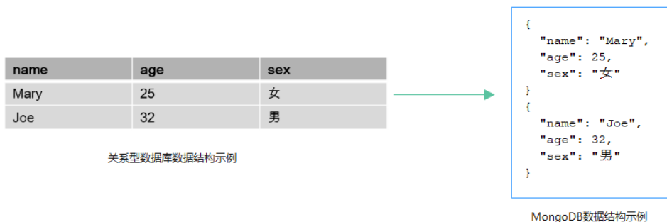
图 1-2 数据结构
