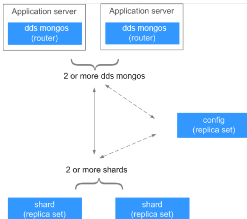
图 10-1 分片集群示意图
