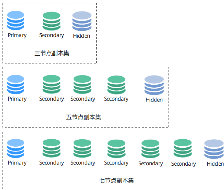
图 7-3 副本集实例节点说明
