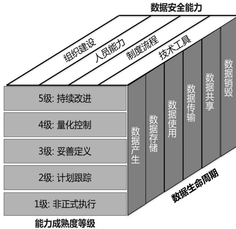
图 7-11 数据安全能力成熟度模型
