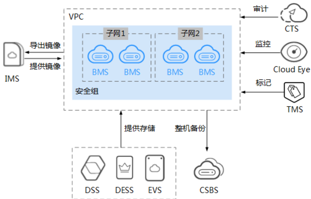
图 13-1 裸金属服务器与其他服务的关系
