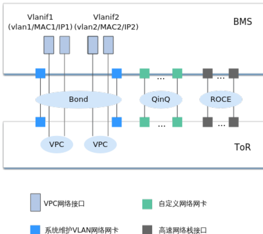
图 8-1 裸金属服务网络
