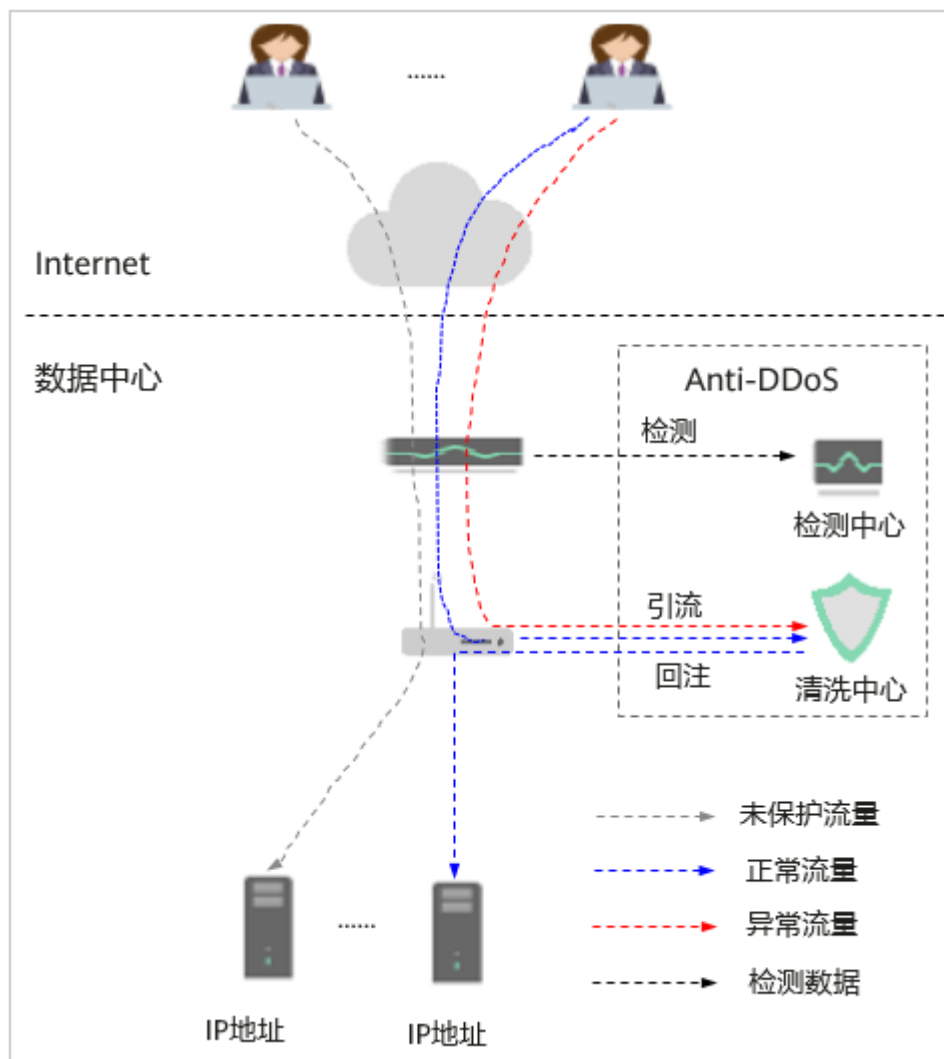
图 2-2 网络拓扑架构图
