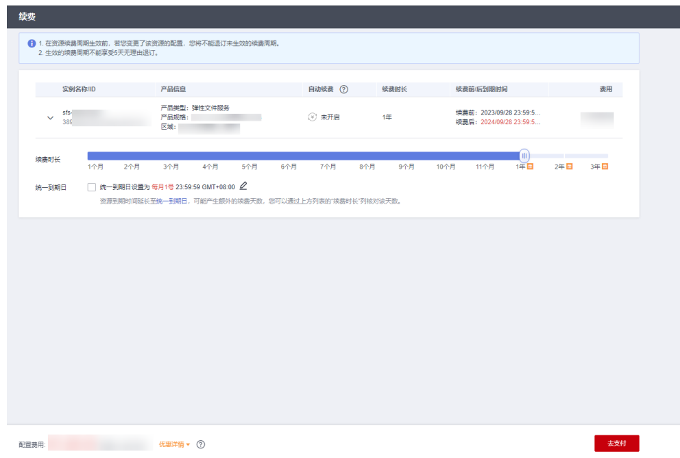
图 6-2 续费确认
