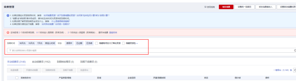
图 6-9 续费管理
