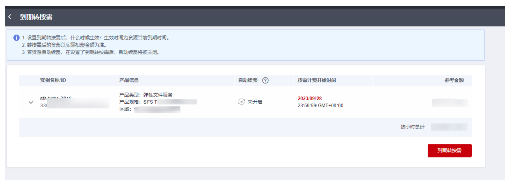
图 5-5 到期转按需
