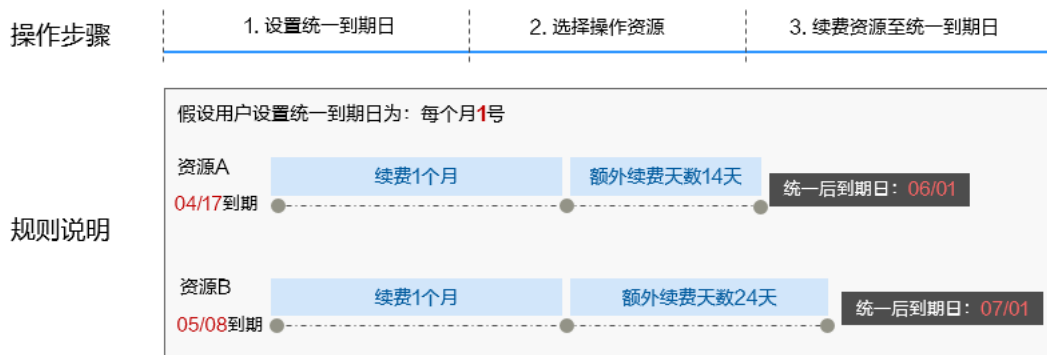
图 6-7 统一到期日
