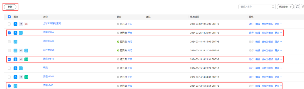
图 10-1 删除流
