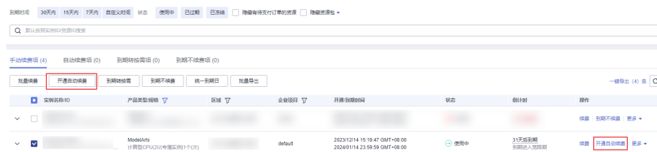
图 5-4 续费管理
