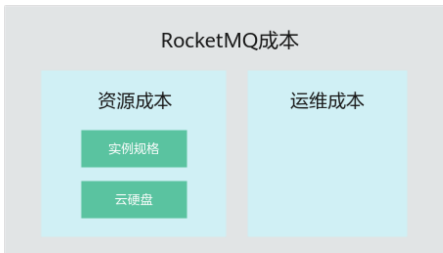
图 10-1 RocketMQ 成本
