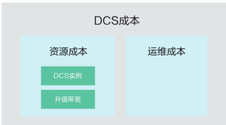
图 9-1 DCS 成本
