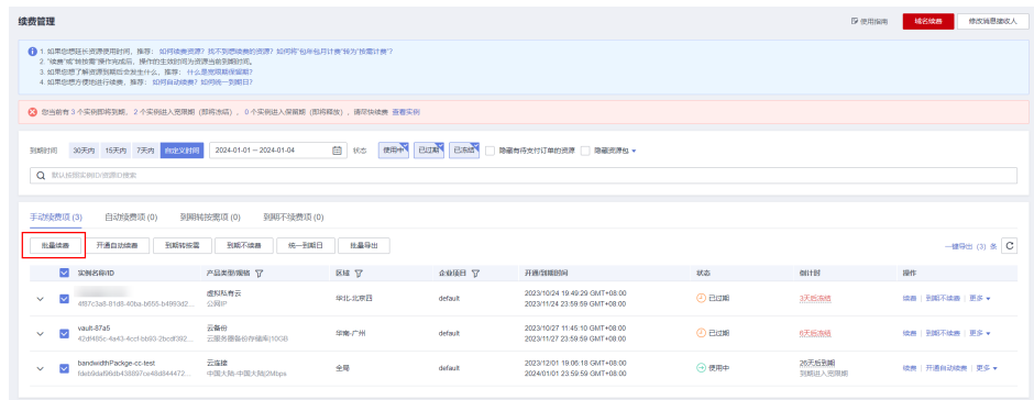
图 6-5 批量续费
