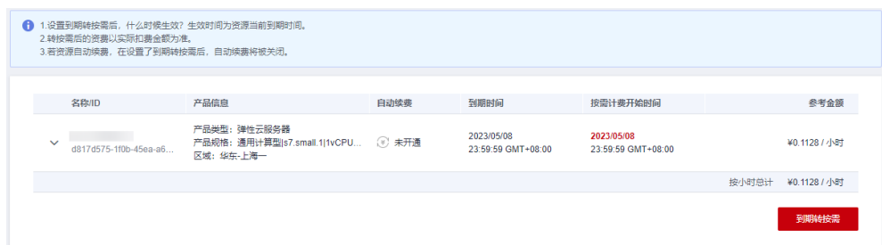
图 5-8 到期转按需
