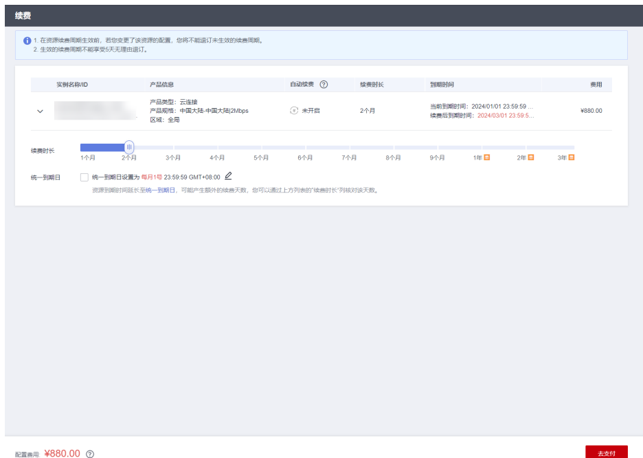
图 6-6 续费确认
