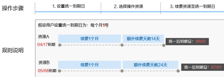
图 6-7 统一到期日
