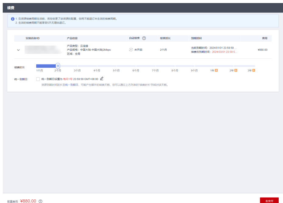
图 6-2 续费确认
