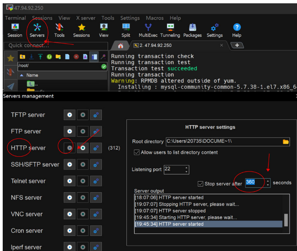
图 5-36 设置 “Stop server after”
