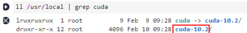
图 5-6 查看当前环境的 cuda 版本
