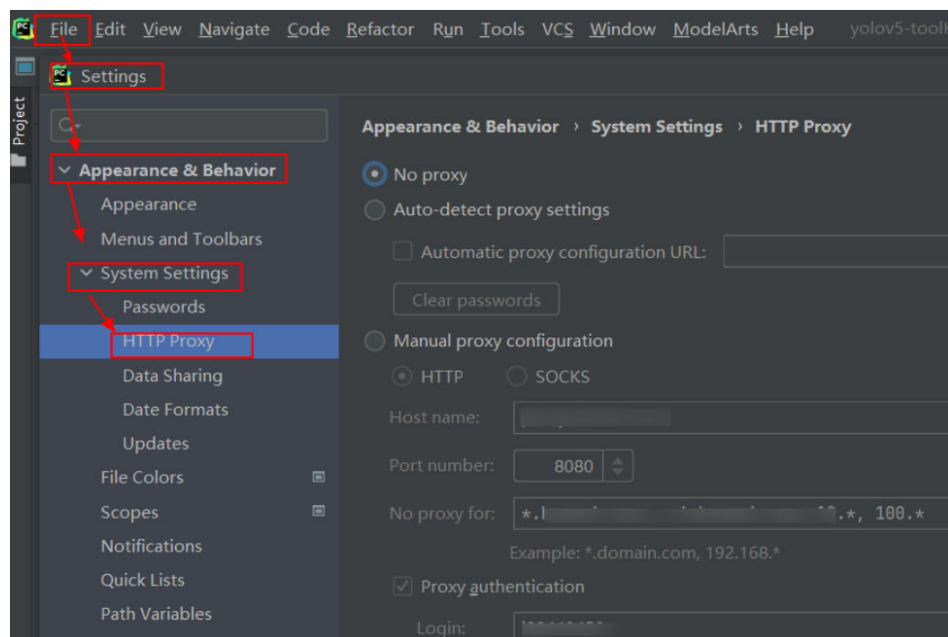
图 5-19 PyCharm 网络代理设置
