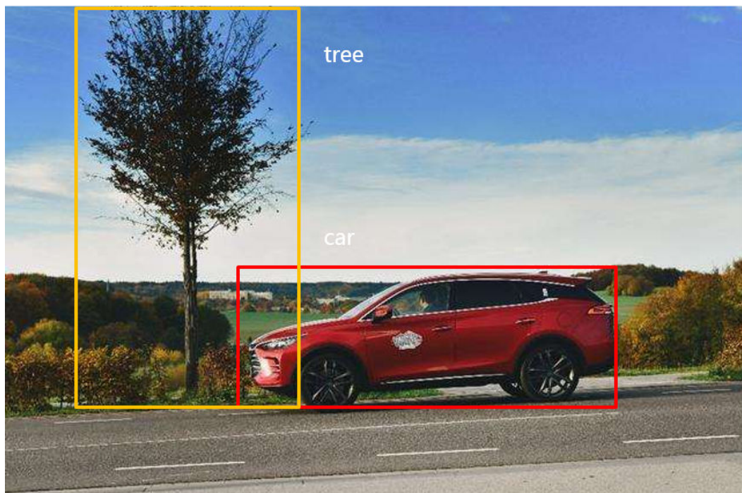
图 3-2 物体检测
