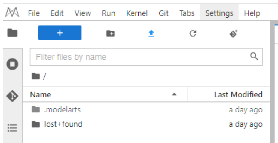
图 5-5 Notebook 的 JupyterLab
