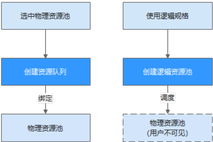
图 10-2 逻辑资源池，资源队列与物理资源池的关系
