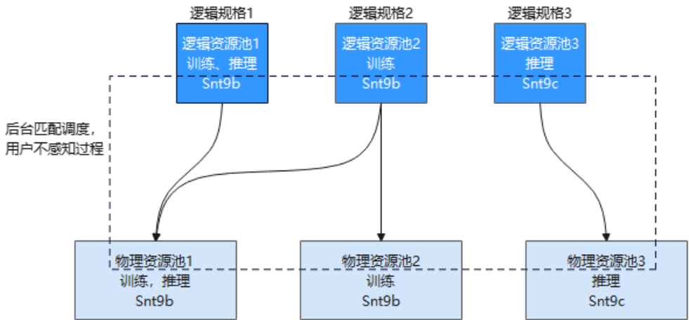
图 10-3 逻辑资源池原理示意图
