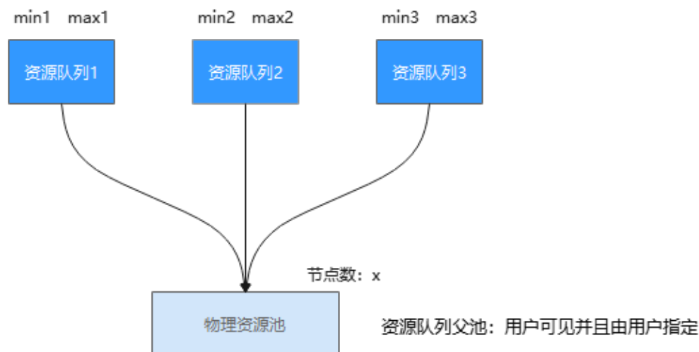
图 10-4 资源队列原理示意图
