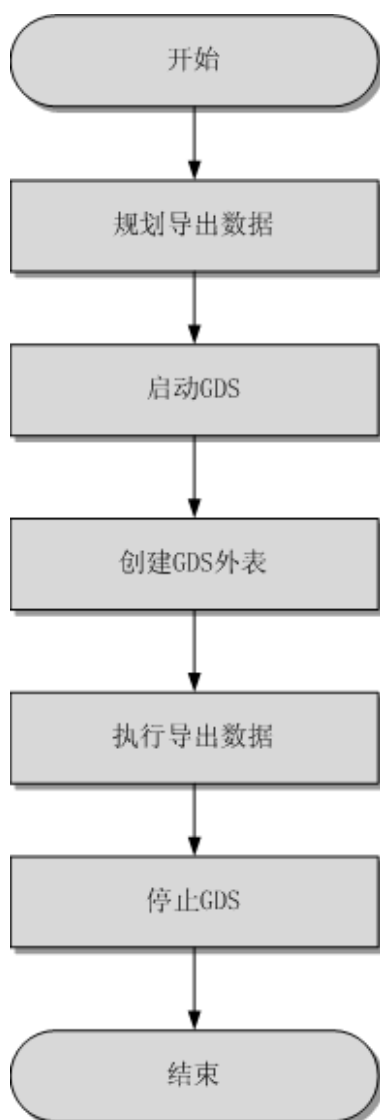
图 7-4 并行导出流程
