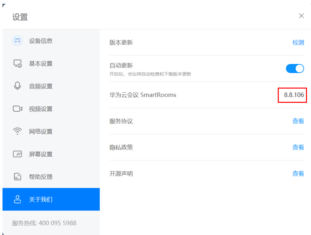
图 6-6 SmartRooms 版本
