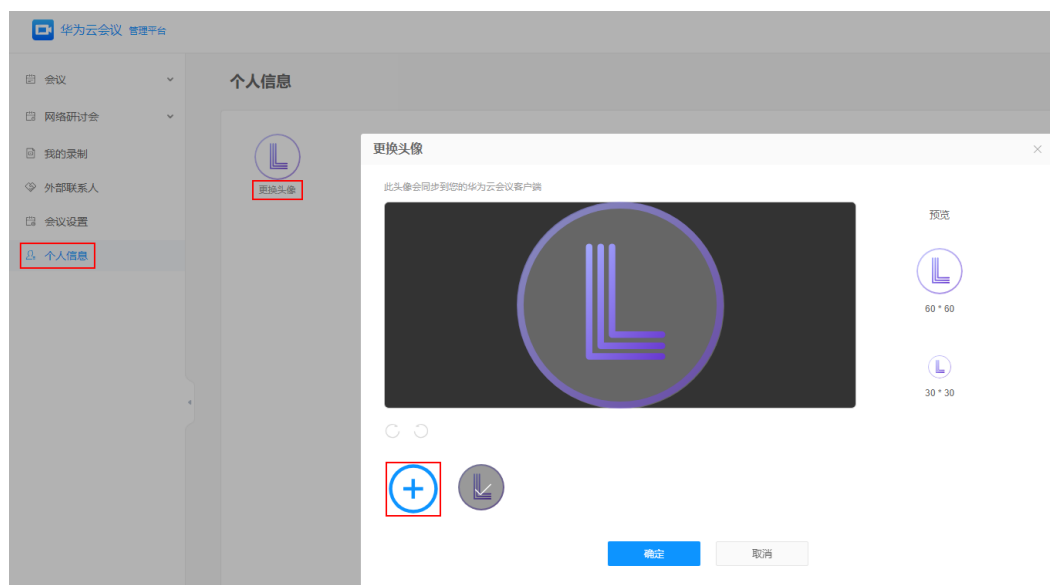
图 6-27 更换头像
