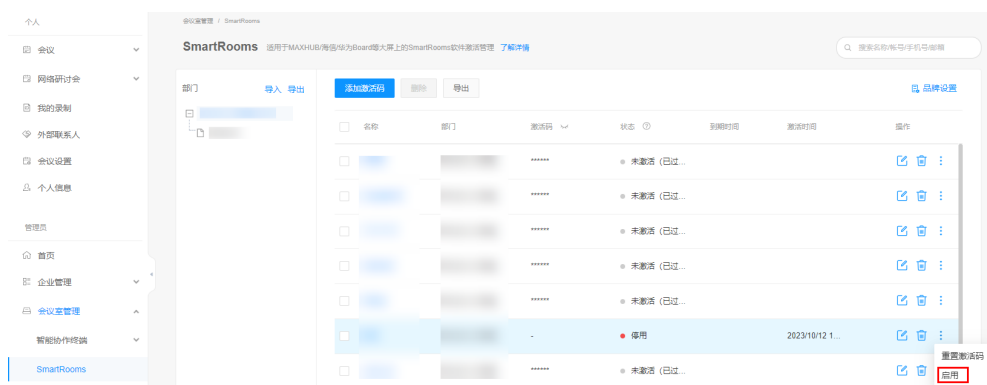
图 10-6 启用设备
