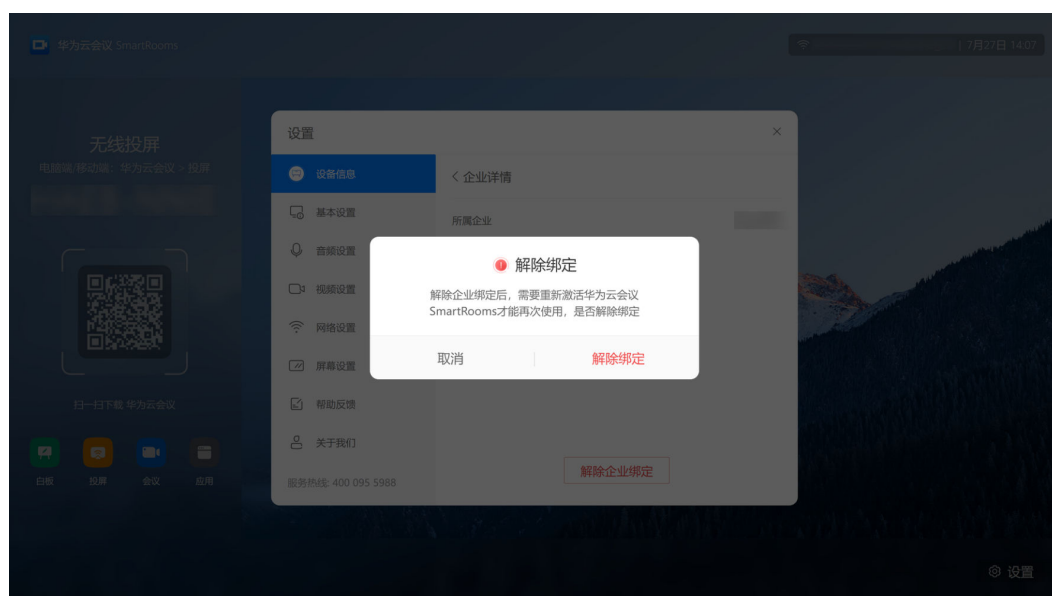
图 6-22 解除绑定
