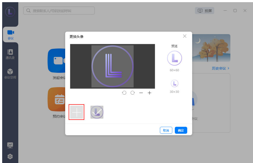
图 6-26 添加头像
