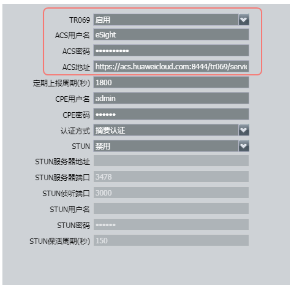
图 10-1 TR069 参数
