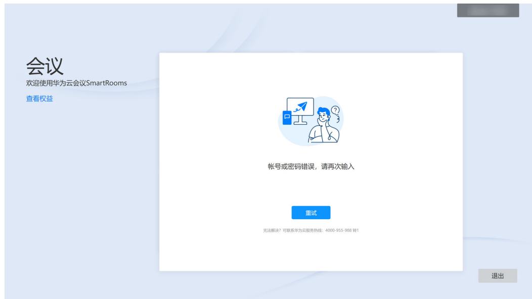
图 6-20 提示
