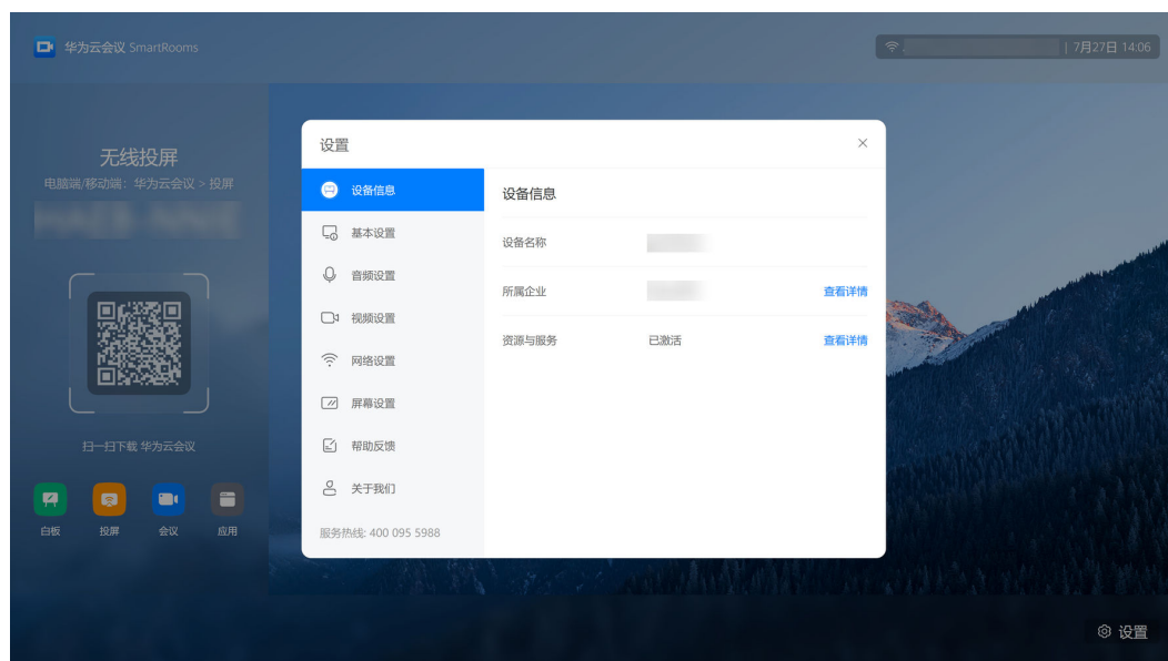
图 6-21 企业详情
