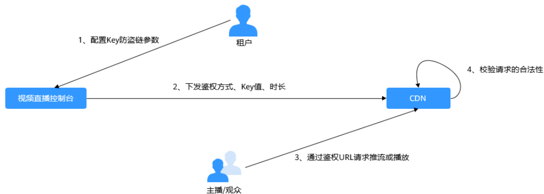
图 7-11 Key 防盗链工作原理
