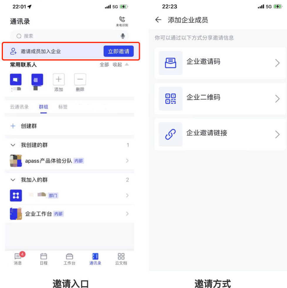
图 4-25 app 端邀请
