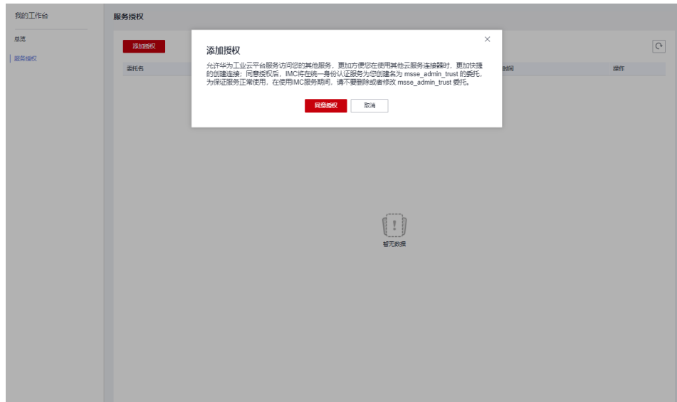
图 2-4 同意授权
