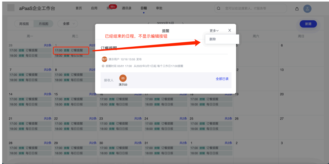
图 5-26 已结束日程
