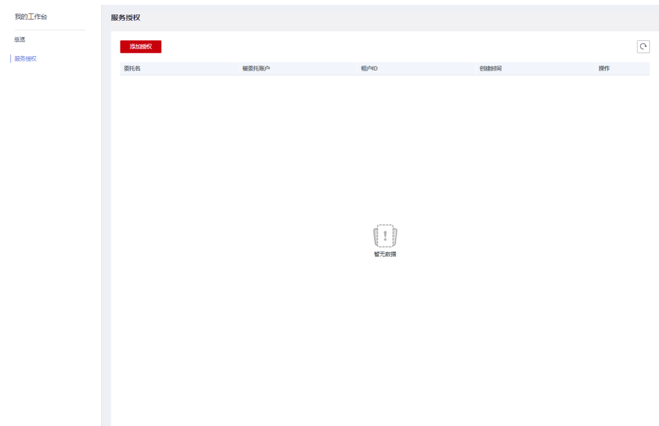
图 2-3 添加授权
