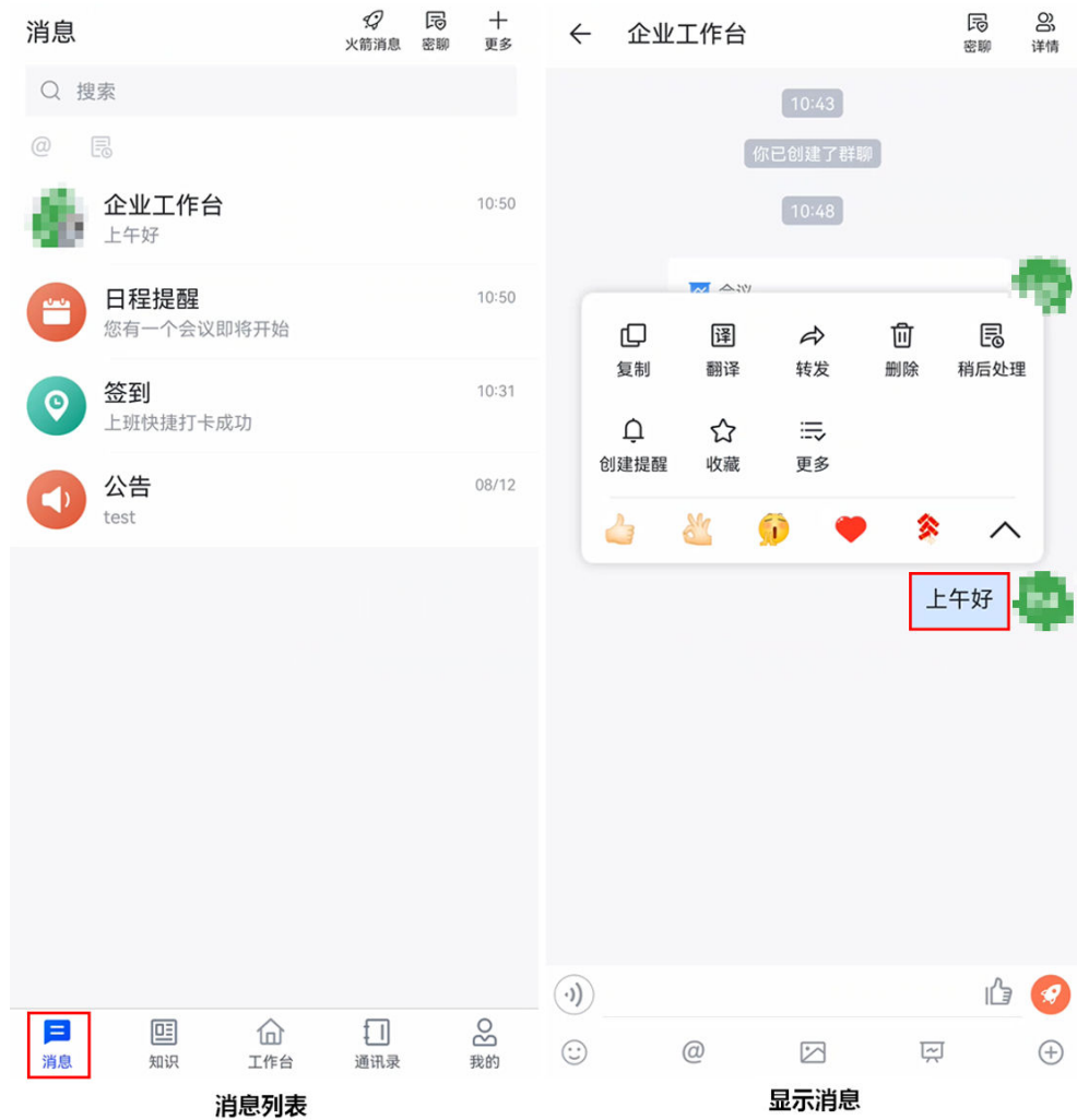
图 6-8 查看消息
