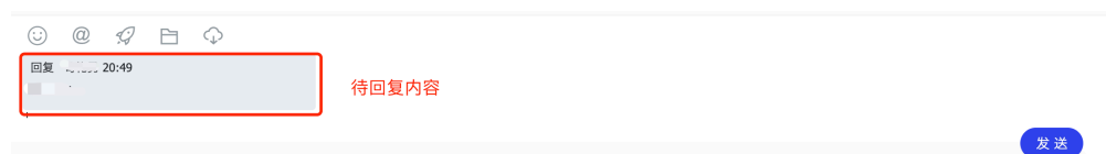
图 5-12 待回复内容
