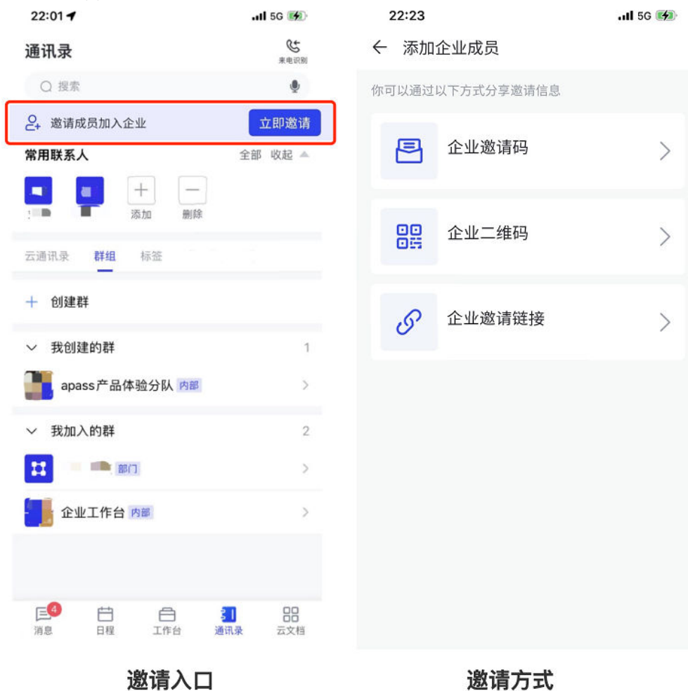
图 6-19 app 端邀请
