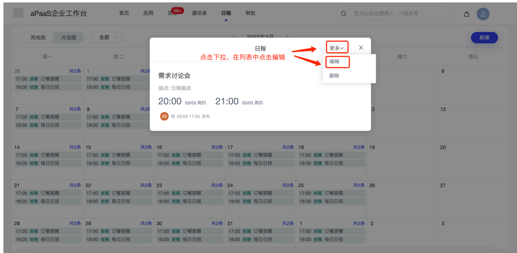
图 5-24 编辑日程
