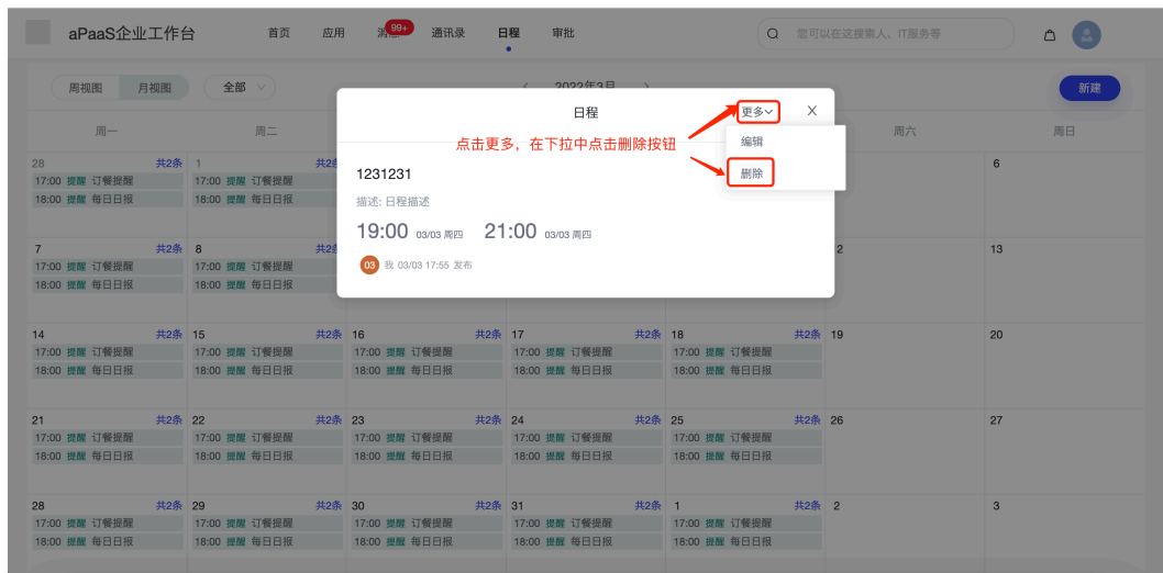
图 5-27 删除日程
