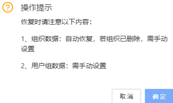
图 4-31 操作提示
