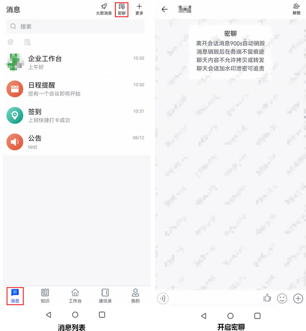
图 6-7 密聊
