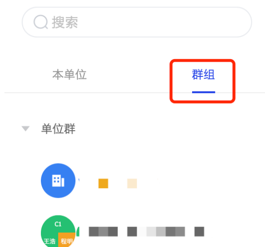
图 5-30 查看群组
