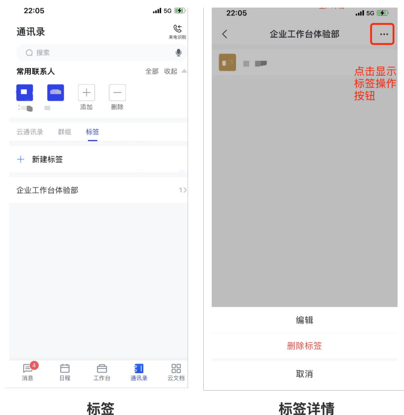
图 6-23 标签
