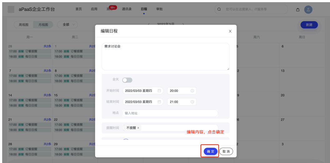
图 5-25 编辑详情页
