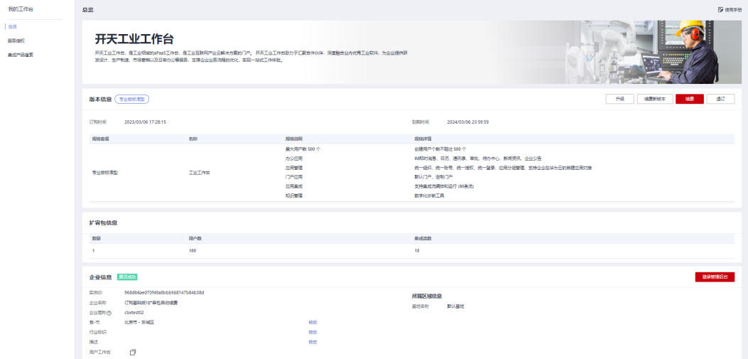
图 3-2 总览页面
