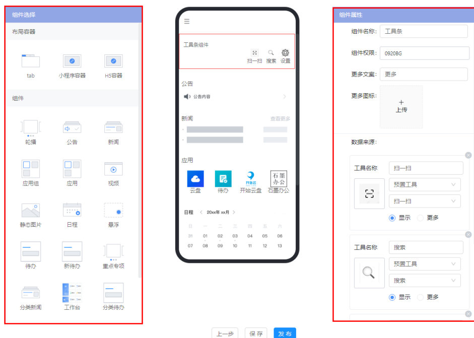
图 4-6 页面编辑
