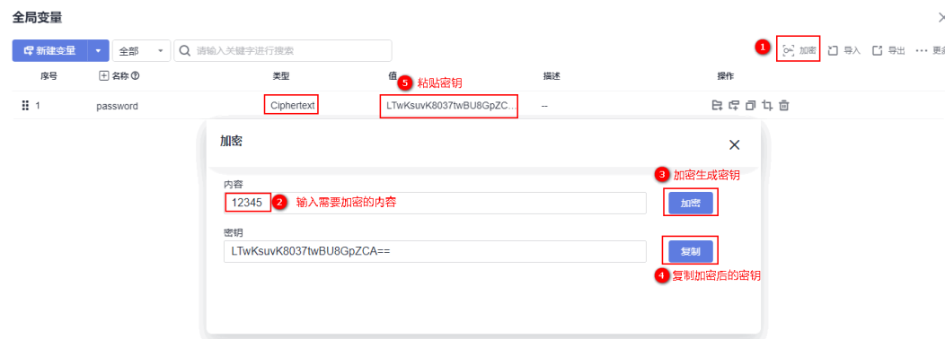
图 5-15 变量加密
