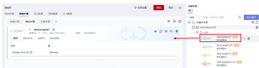
图 5-11 调用接口
