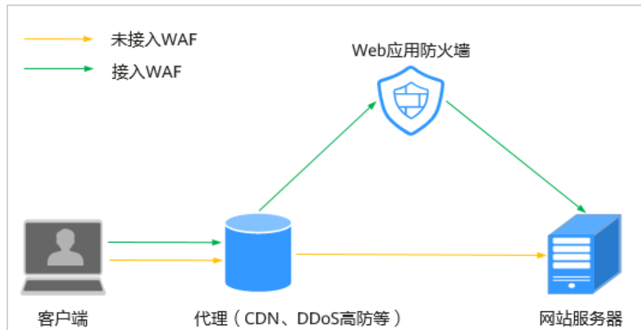
图 7-1 使用代理配置原理图
