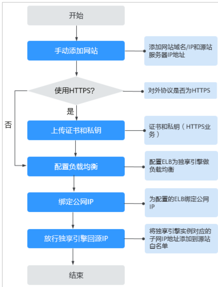
图 7-33 网站接入 WAF 的操作流程图-独享模式
