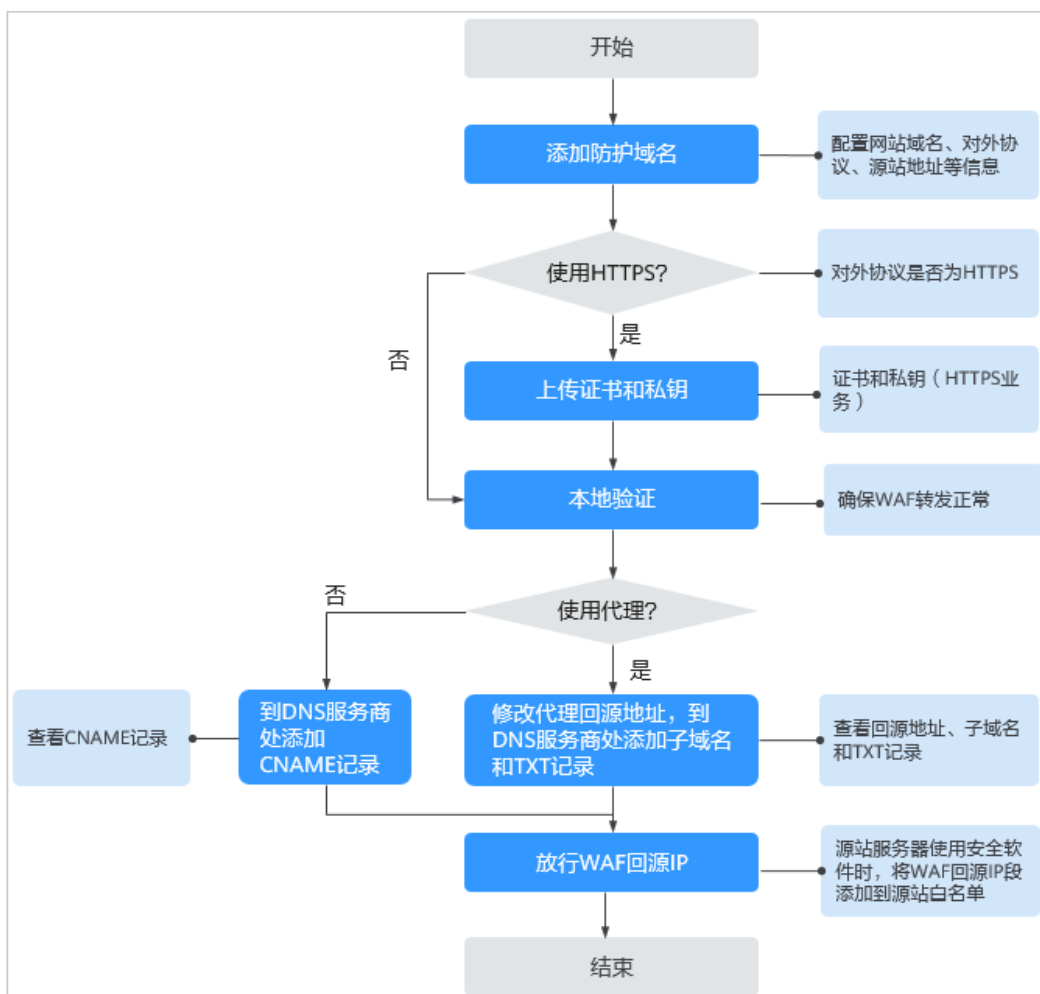
图 7-3 网站接入 WAF 的操作流程图-云模式（CNAME 接入）
