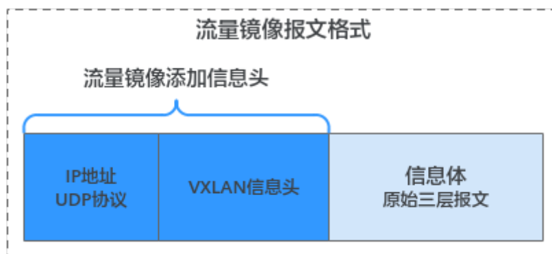
图 12-4 流量镜像报文格式
