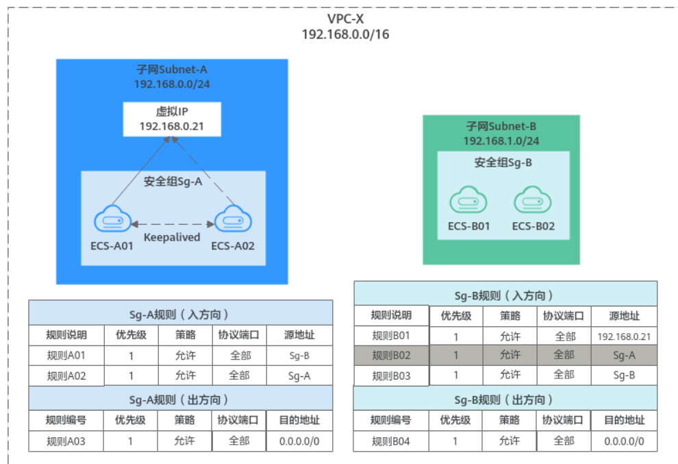
图 6-7 控制虚拟 IP 访问安全组内实例
