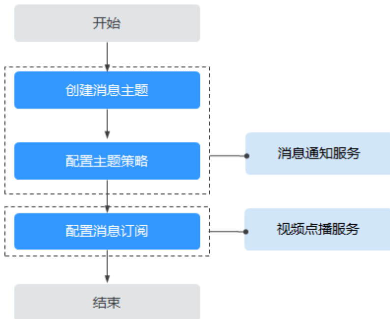
图 5-14 消息订阅配置流程图
