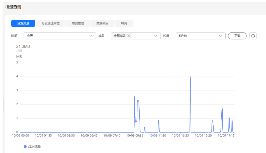
图 10-1 CDN 总流量
