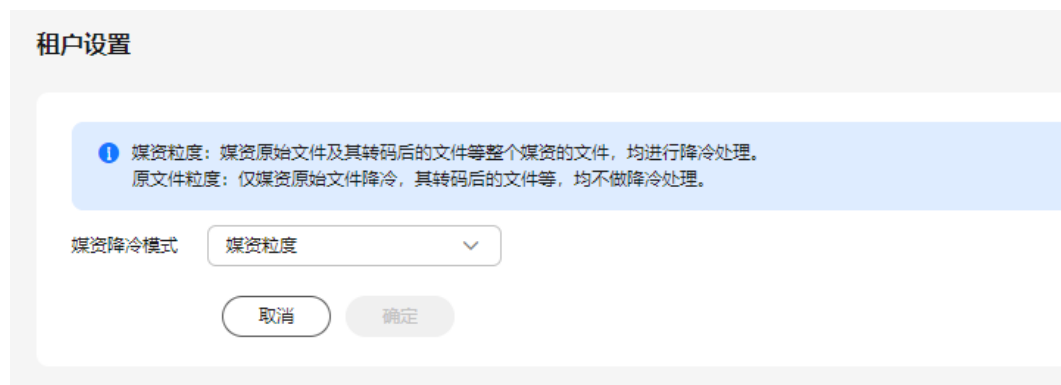
图 8-10 租户设置
