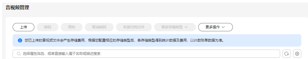
图 6-4 音视频搜索
