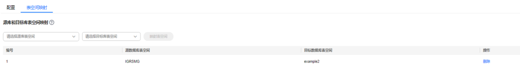
图 4-6 表空间映射
