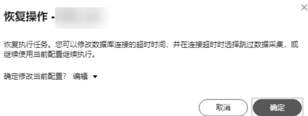
图 3-3 恢复操作
