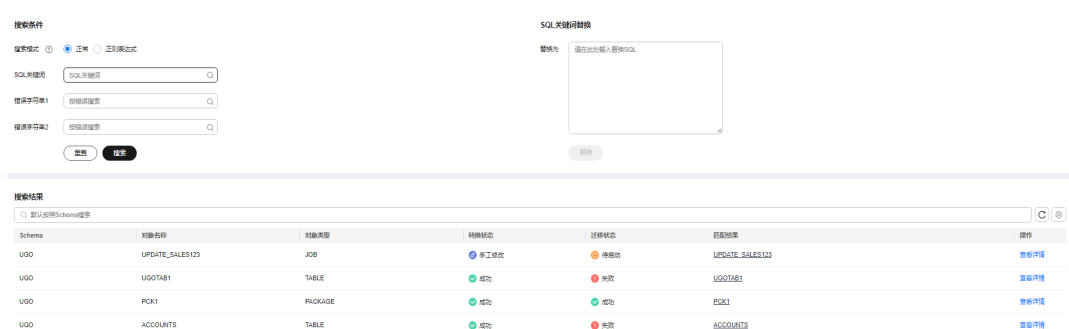
图 4-14 批量修改
