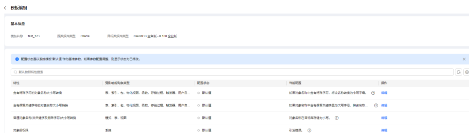
图 6-3 模板编辑
