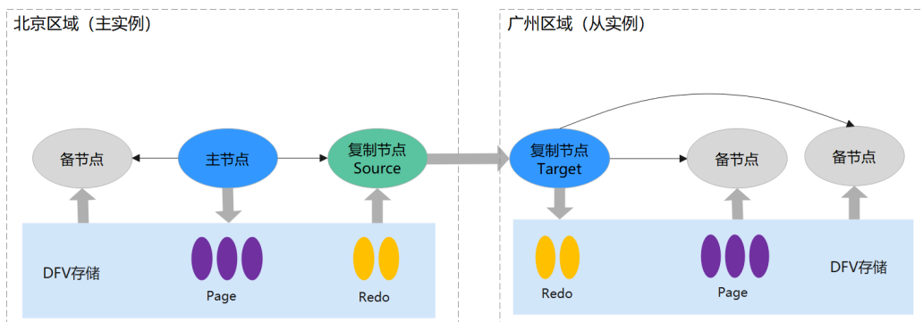
图 19-2 架构原理
