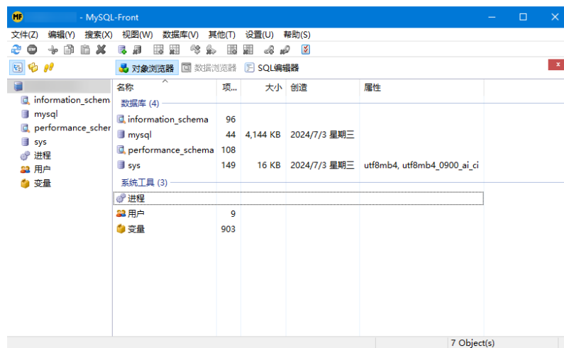
图 3-34 登录成功
