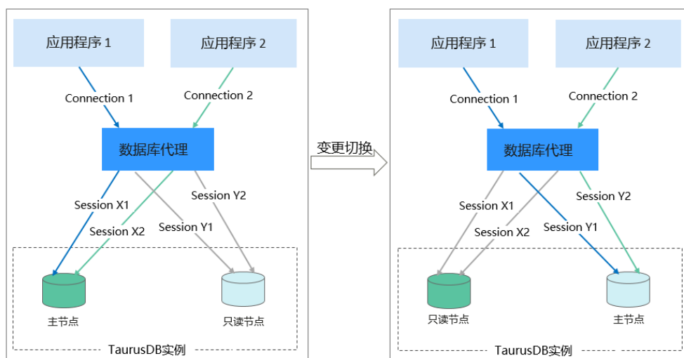
图 17-1 架构图
