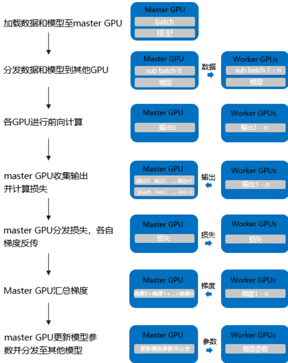
图 8-16 单机多卡数据并行训练
