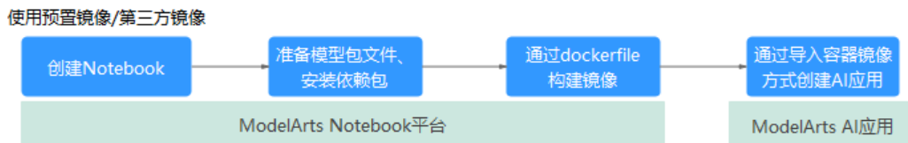
图 10-26 AI 应用的自定义镜像制作场景二
