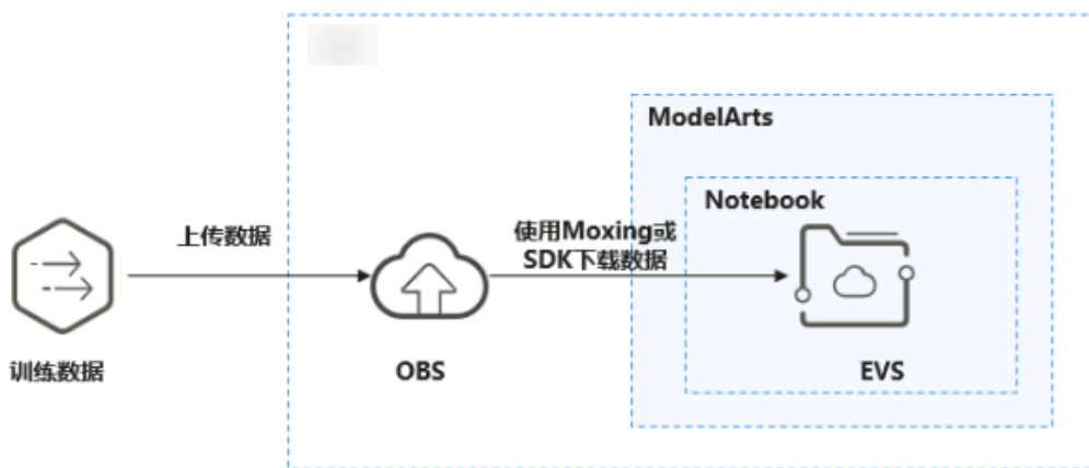
图 6-103 数据通过 OBS 中转上传到 Notebook
