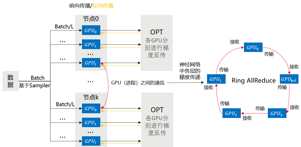
图 8-17 多机多卡数据并行训练
