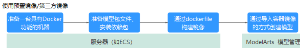
图 10-27 模型的自定义镜像制作场景三
