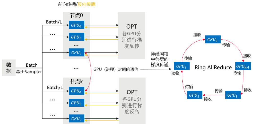
图 8-16 多机多卡数据并行训练
