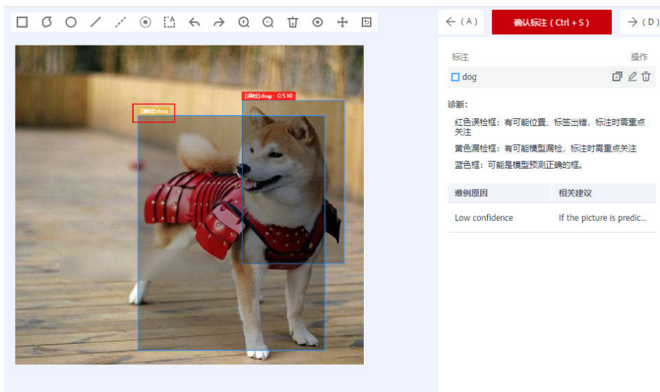
图 7-66 物体检测的难例确认
