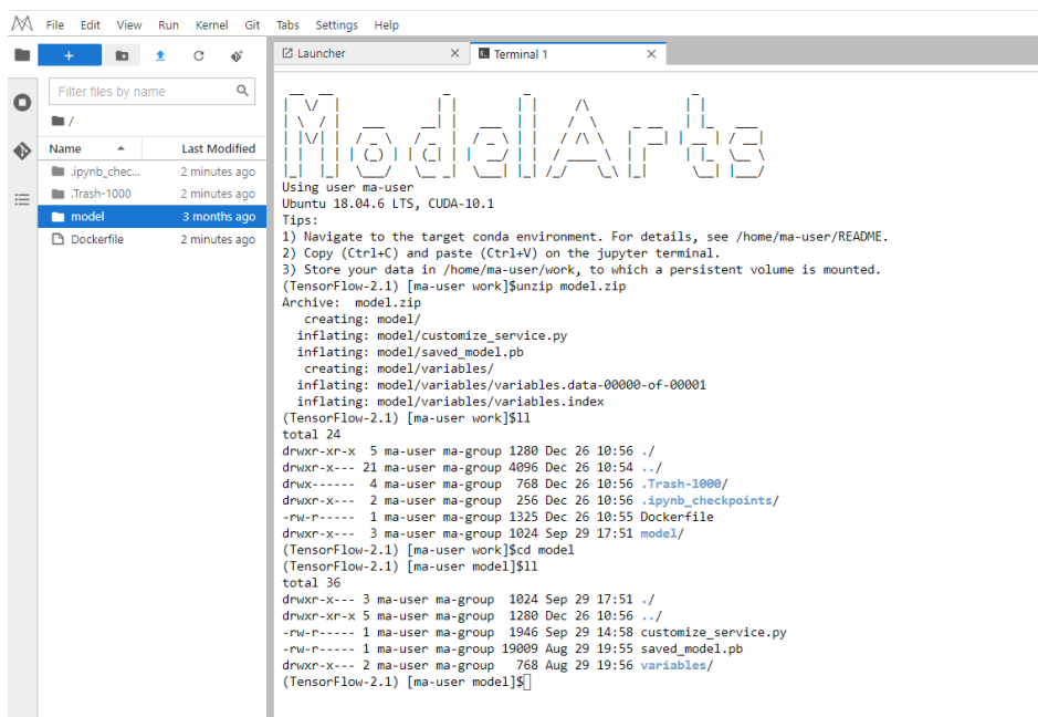
图 10-43 在 Terminal 终端中解压 model.zip
