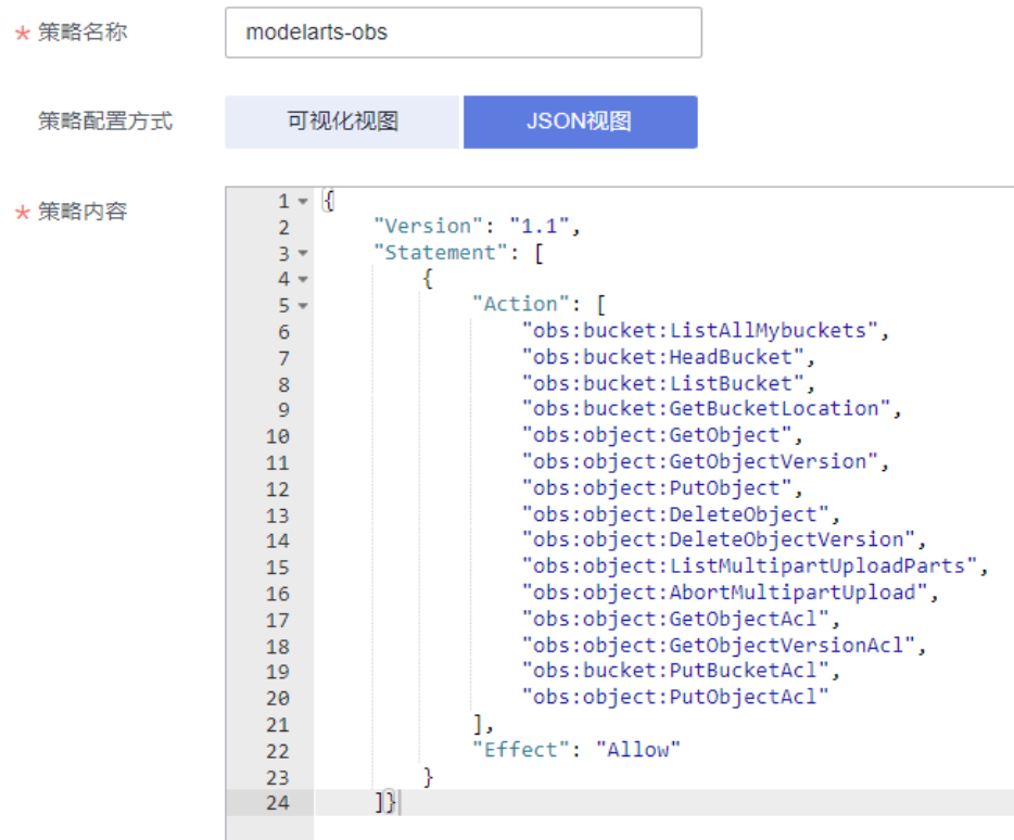
图 2-12 OBS 相关的最大化权限
