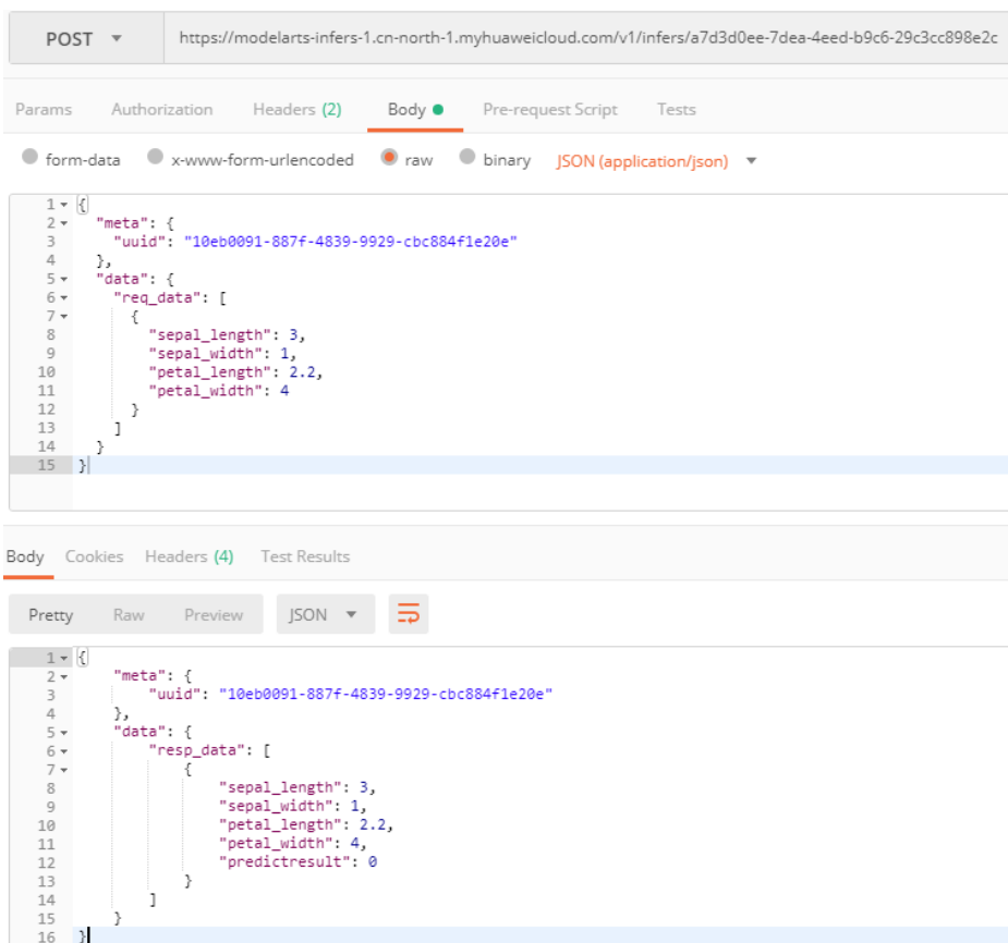
图 9-20 文本输入预测结果
