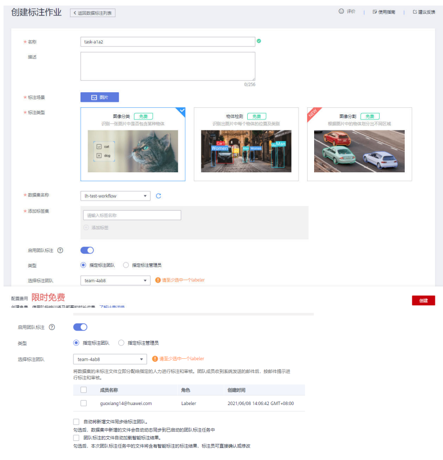
图 7-74 创建团队标注任务
