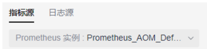
图 11-2 选择指标源
