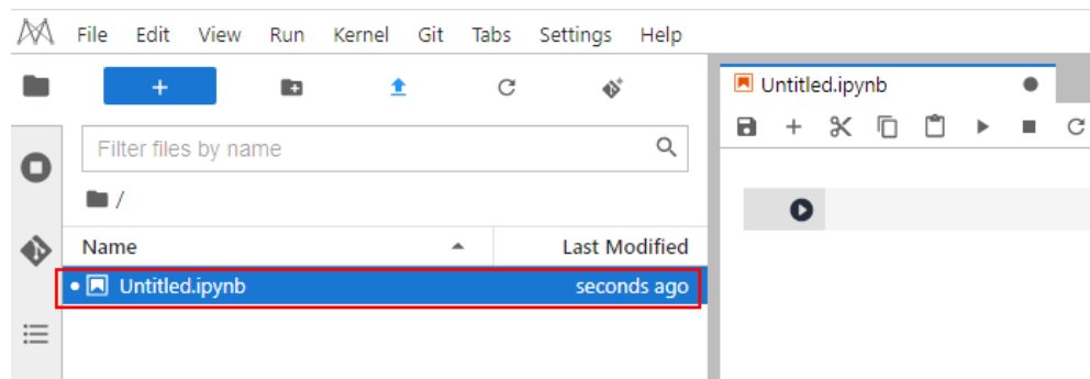
图 6-14 新建文件
