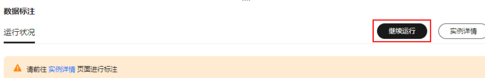
图 4-20 继续运行
