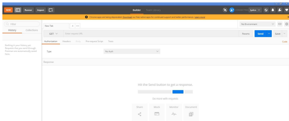
图 9-16 Postman 界面
