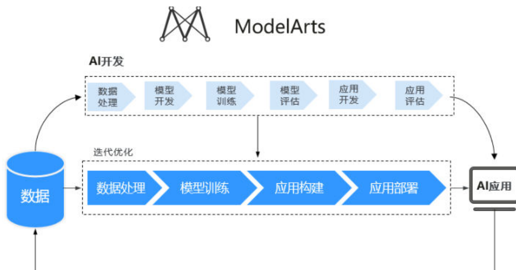
图 5-2 Workflow
