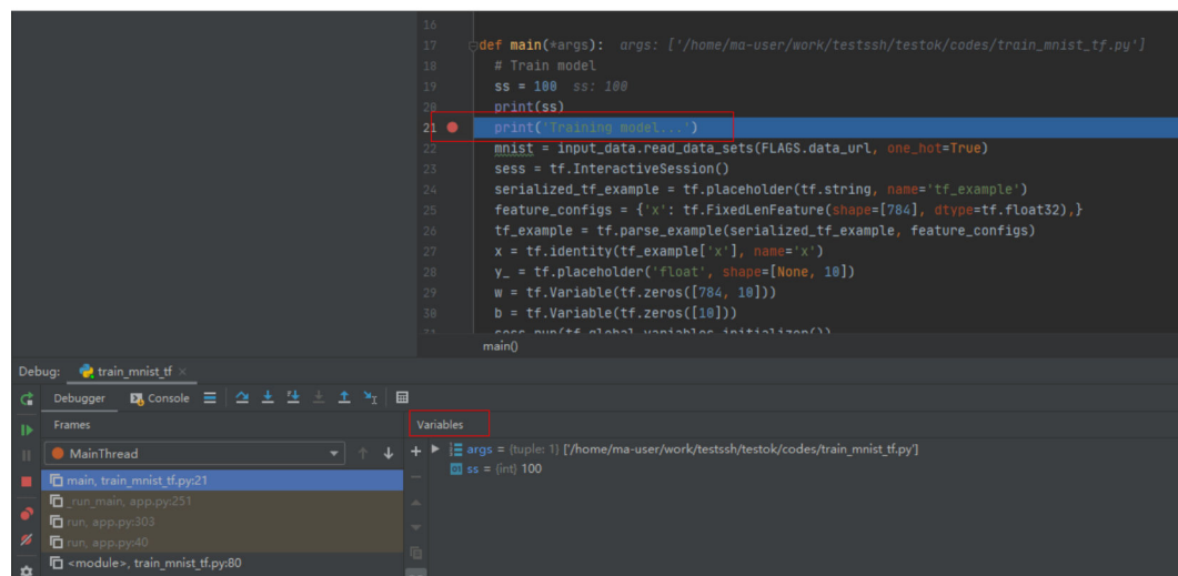
图 6-110 Debug 模式
