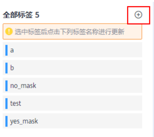
图 7-27 全部标签
