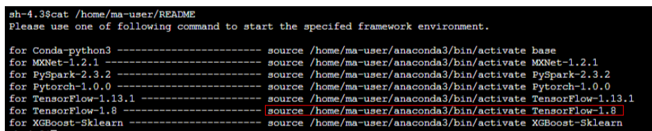
图 6-12 激活环境
