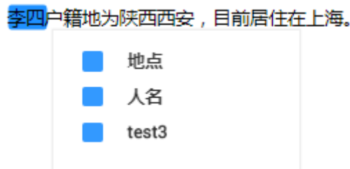
图 7-42 实体标注
