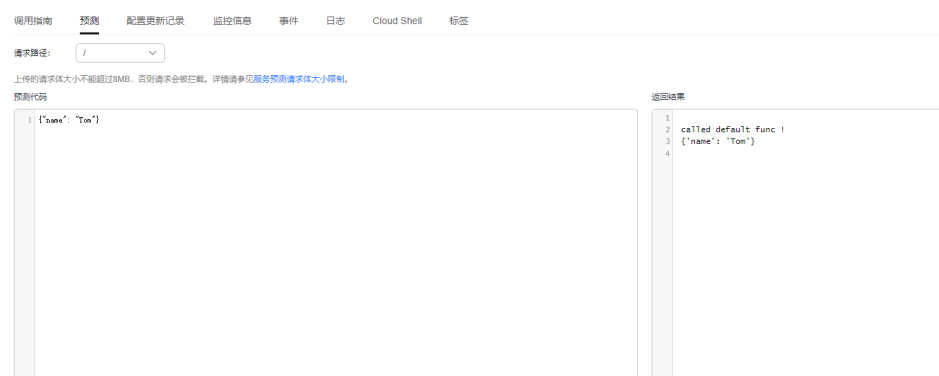
图 9-8 服务预测
