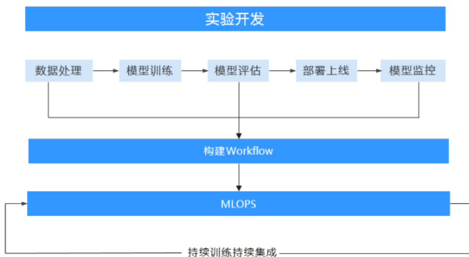
图 5-1 MLOps
