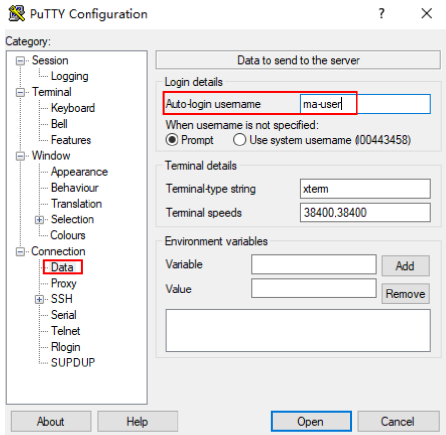
图 6-144 填写用户名
