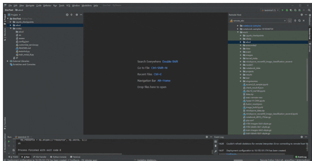
图 6-103 配置 SSH
