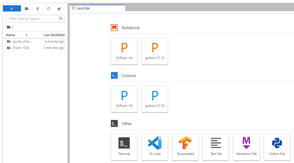
图 6-10 JupyterLab 主页
