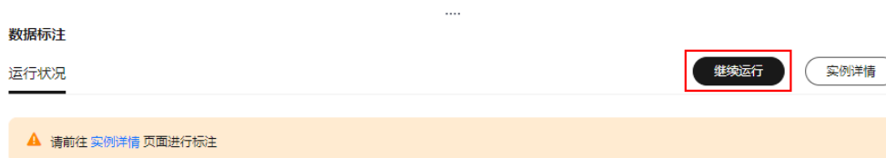
图 4-10 继续运行
