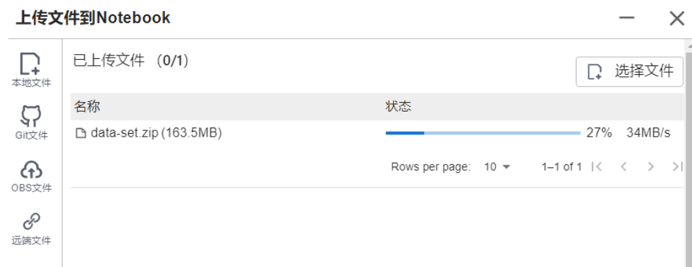
图 6-58 上传文件
