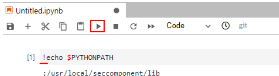
图 6-19 运行代码
