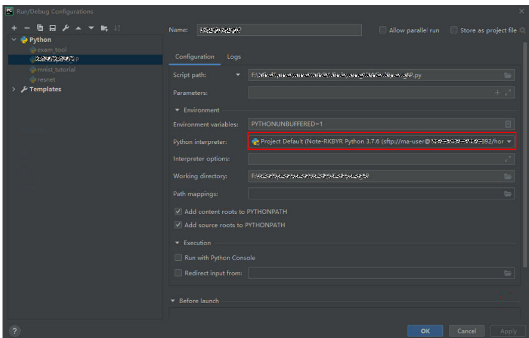
图 6-99 设置运行参数 (2)
