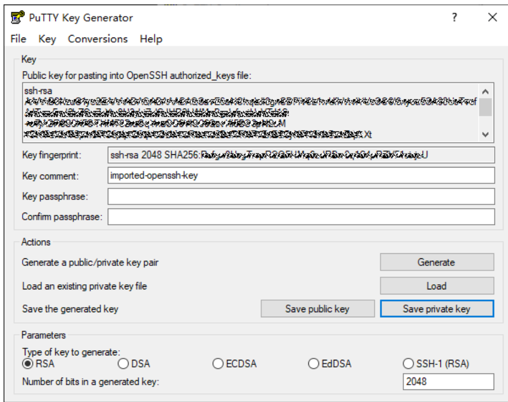
图 6-141 将密钥对.pem 文件转成.ppk 文件
