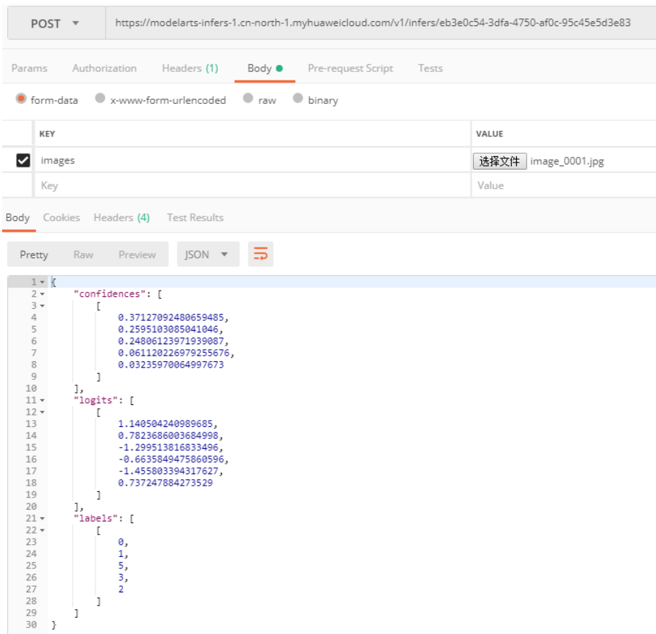
图 9-19 文件输入预测结果
