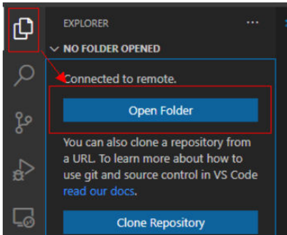
图 6-126 Open Folder
