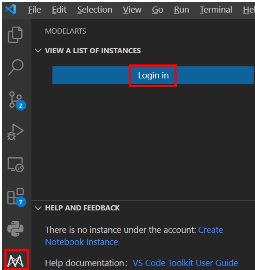
图 6-118 安装完成
