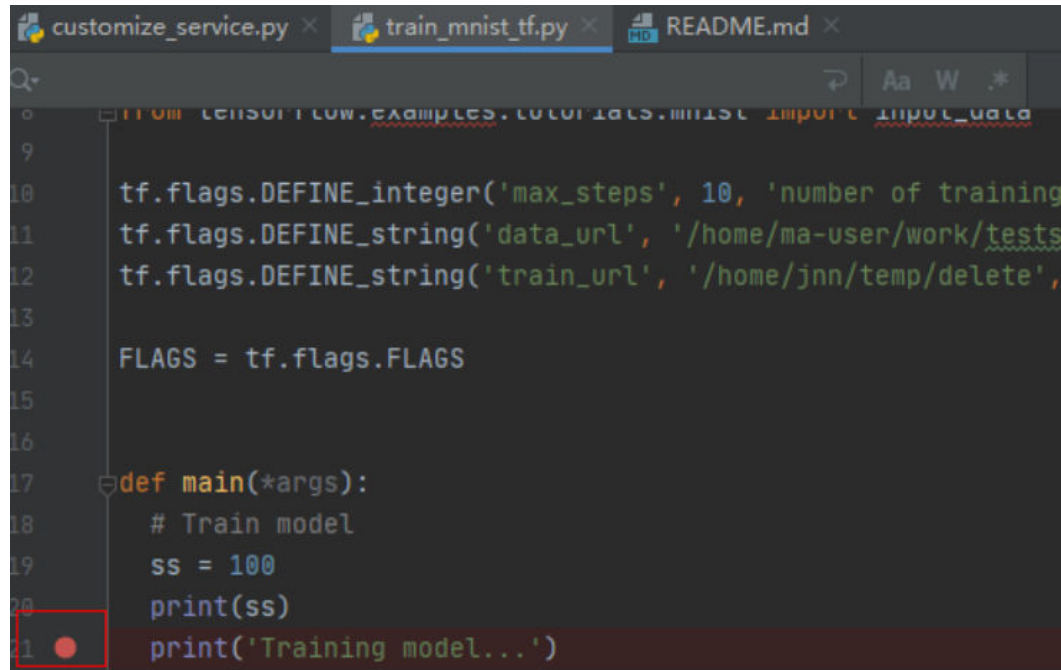
图 6-108 代码打断点
