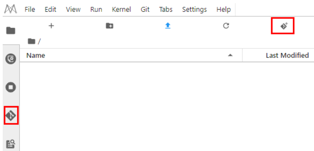
图 6-32 Git 插件
