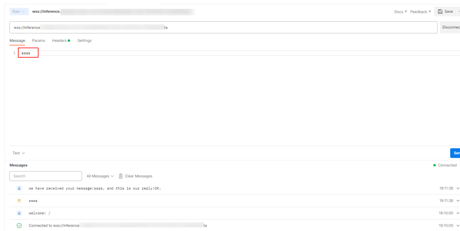
图 9-42 发送数据
