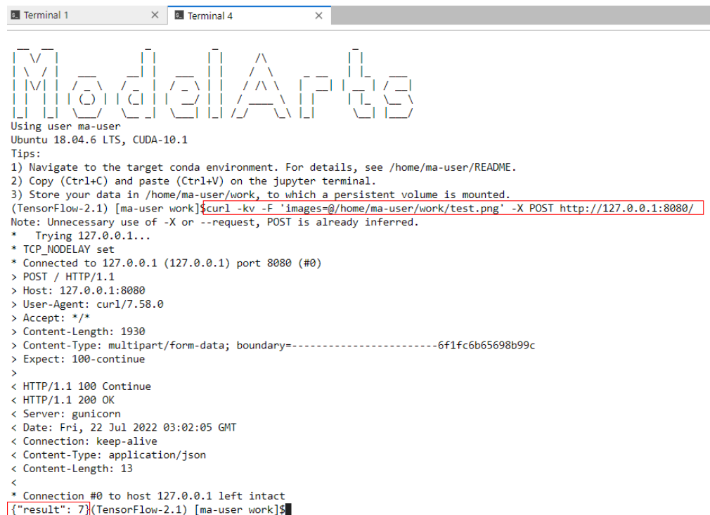
图 10-52 预测
