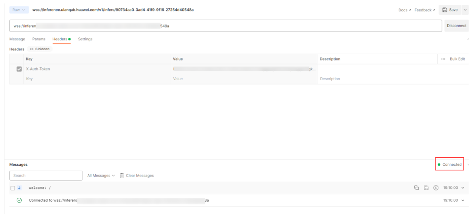
图 9-41 连接成功
