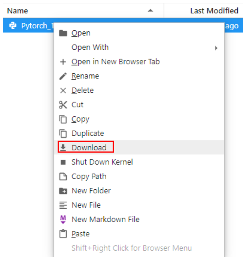
图 6-80 下载文件
