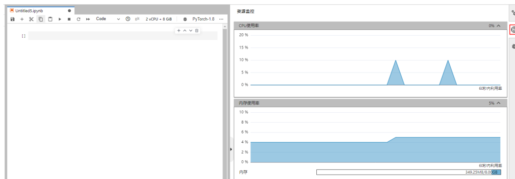
图 6-31 资源监控
