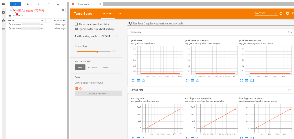
图 6-86 TensorBoard 界面 (1)
