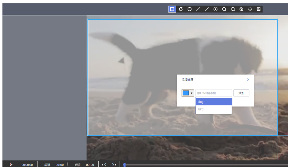
图 7-51 视频标注
