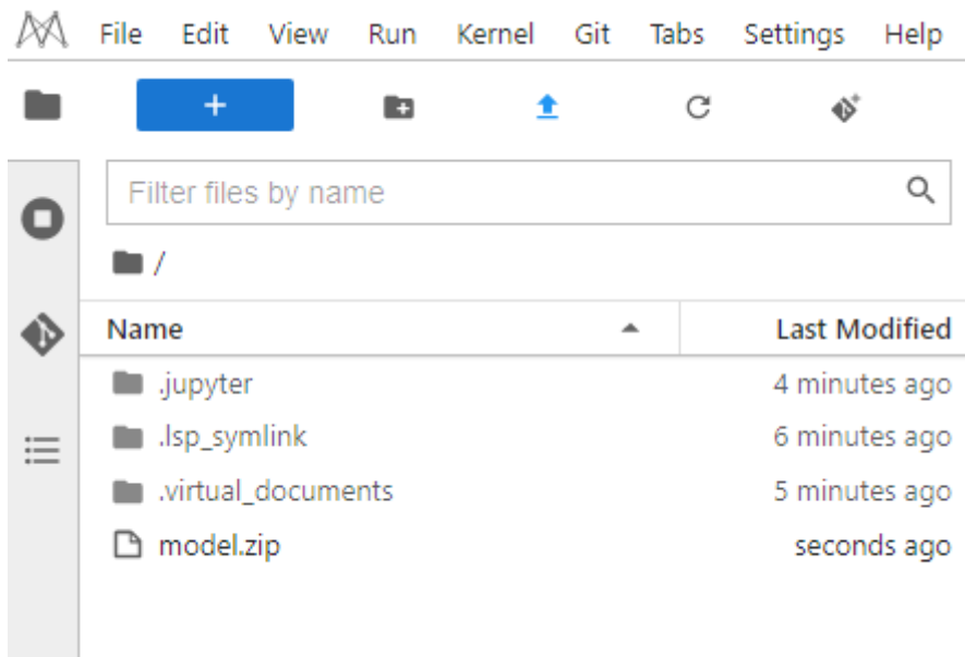
图 10-30 上传模型包
