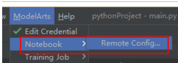
图 6-90 配置插件
