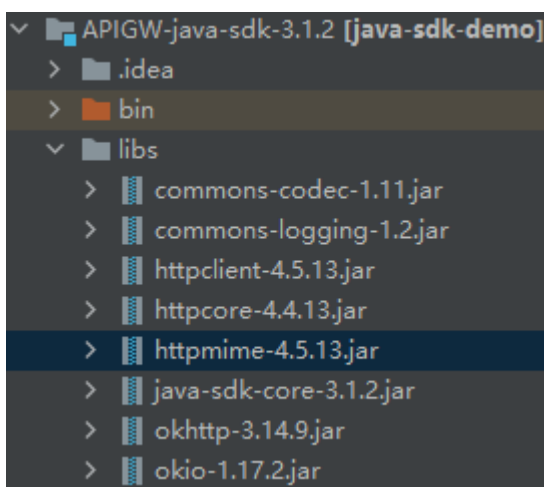
图 9-29 Java 依赖库
