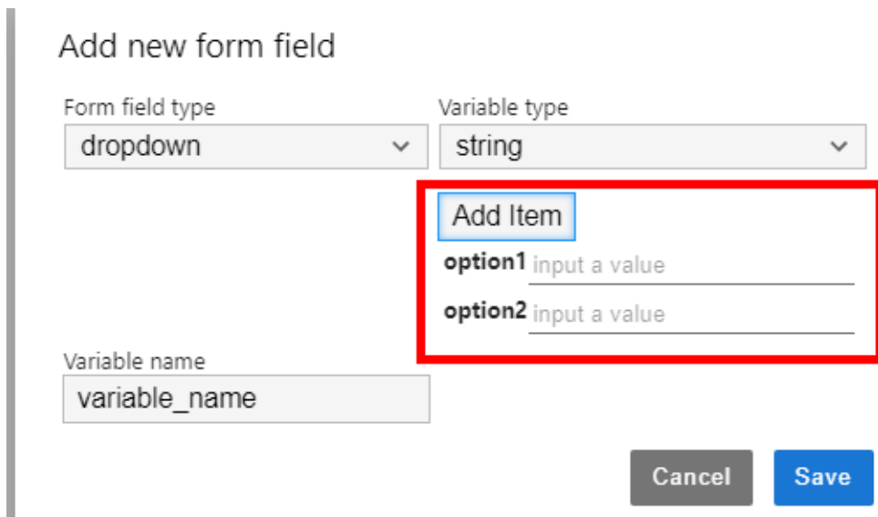
图 6-29 创建“dropdown”类型的表单
