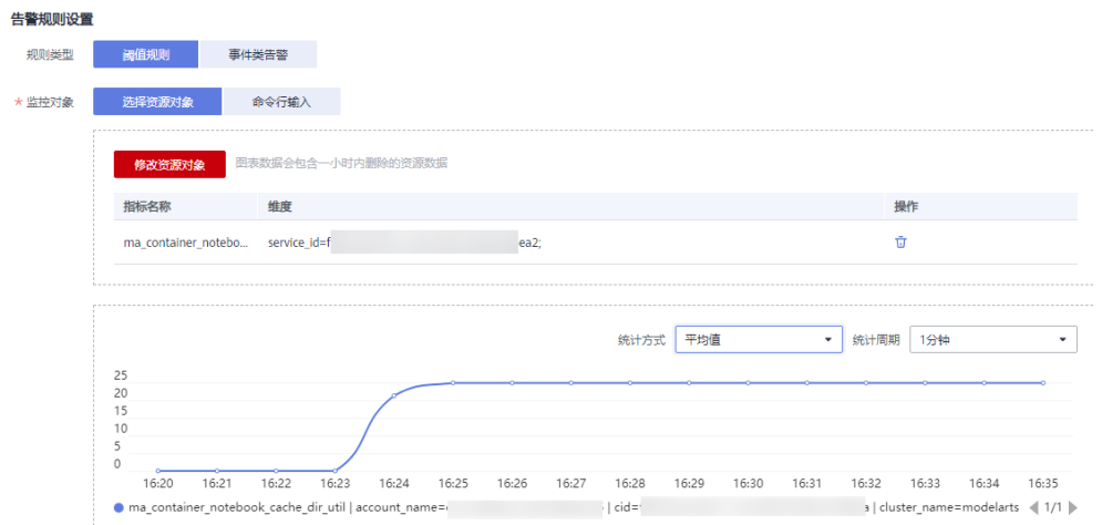
图 6-161 设置指标统计方式
