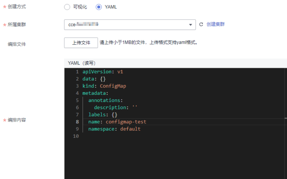
图 3-7 YAML 方式设置配置项参数
