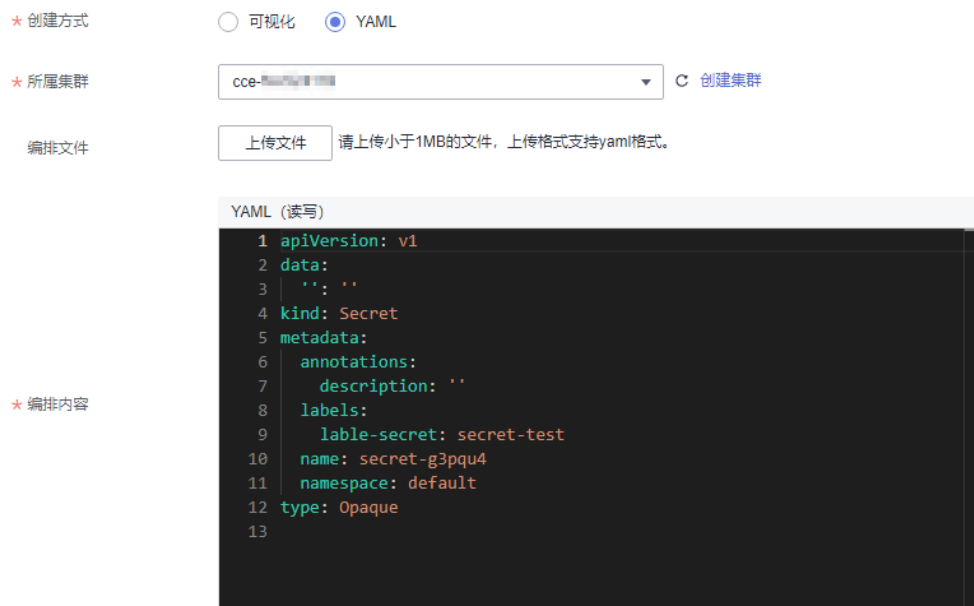
图 3-9 YAML 方式设置密钥参数
