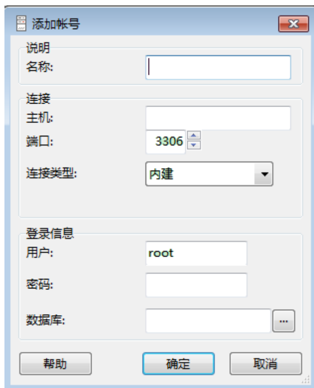
图 1-27 添加信息
