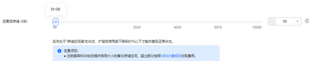
图 4-23 扩容磁盘
