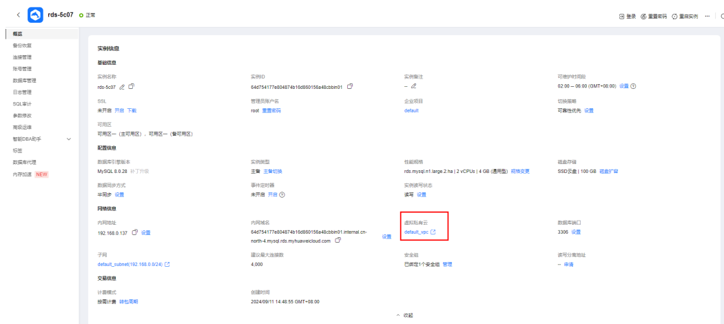
图 1-13 MySQL 概览
