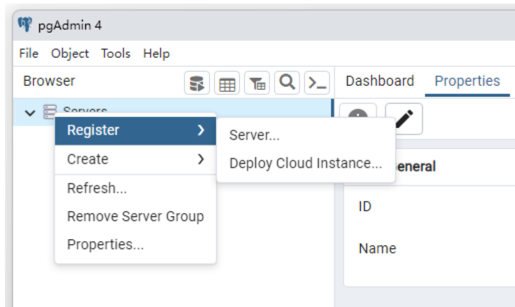
图 3-27 Servers
