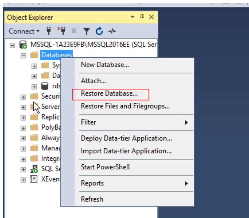
图 4-48 选择数据库
