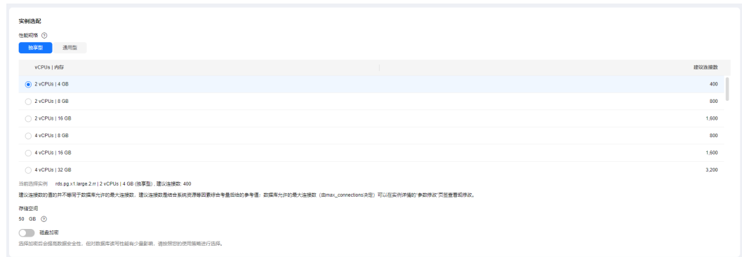
图 3-61 规格与存储
