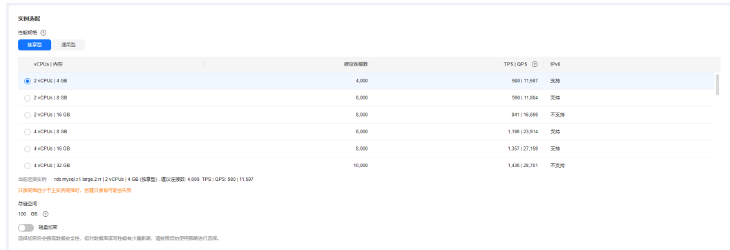
图 1-99 实例选配
