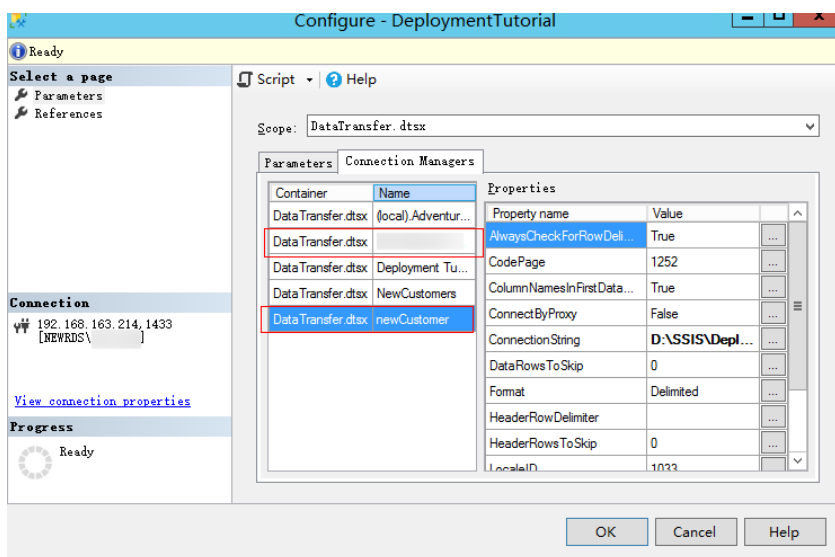
图 4-91 配置参数
