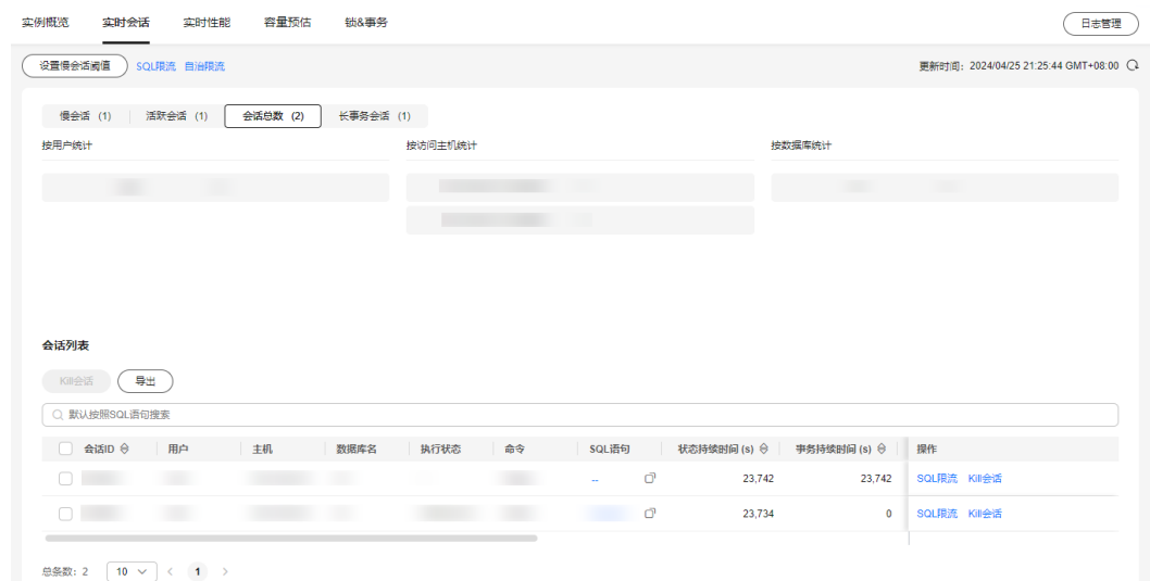
图 1-144 实时会话
