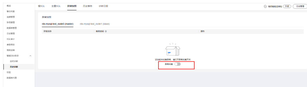
图 1-163 异常快照
