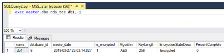
图 4-85 开启状态
