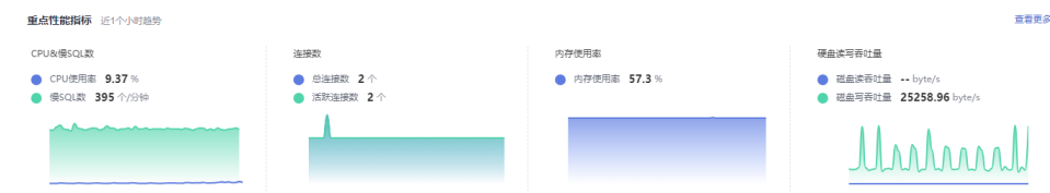
图 2-59 性能指标
