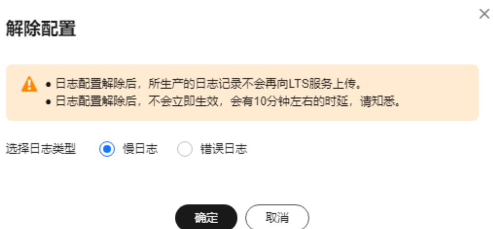
图 1-204 解除配置
