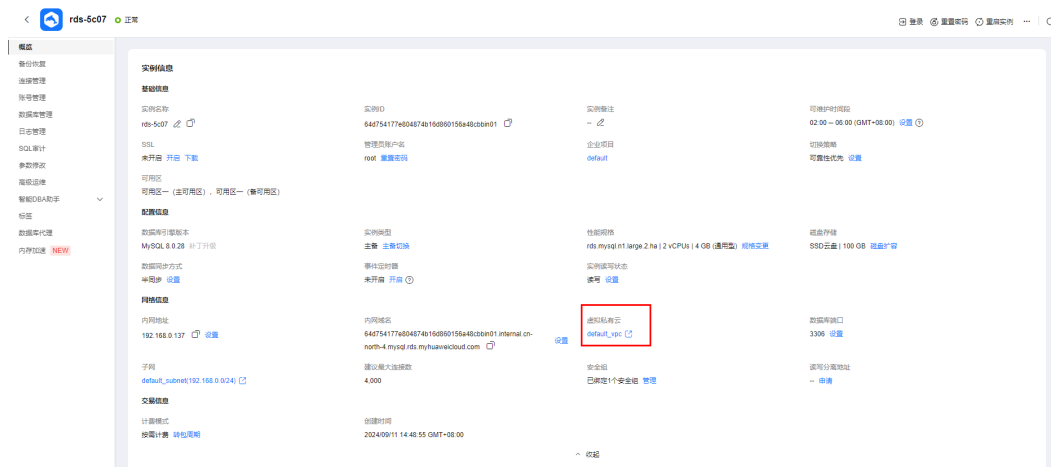
图 1-20 MySQL 概览
