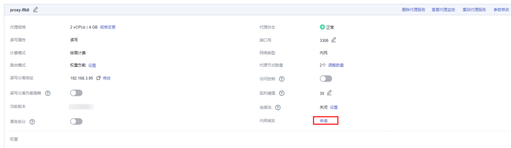
图 1-129 代理信息
