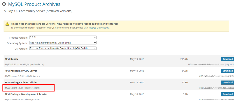
图 1-25 下载
