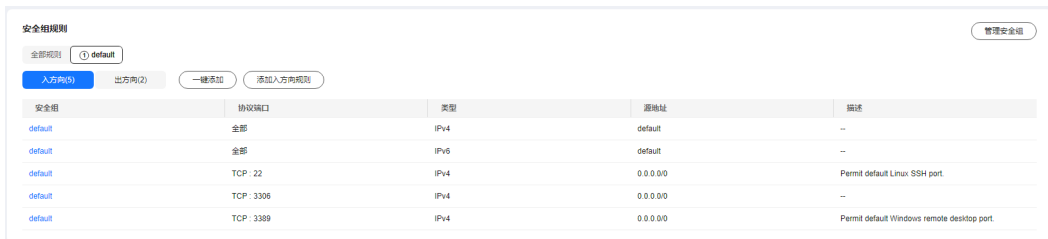
图 1-114 放通 3306 端口
