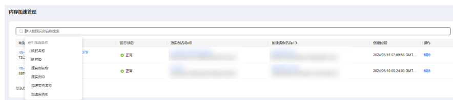
图 1-241 映射列表
