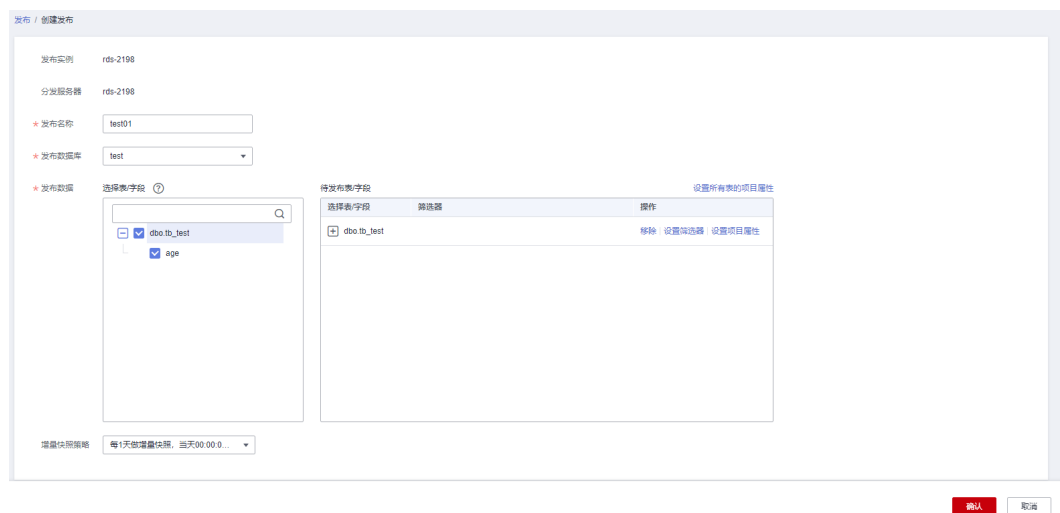
图 4-115 创建发布
