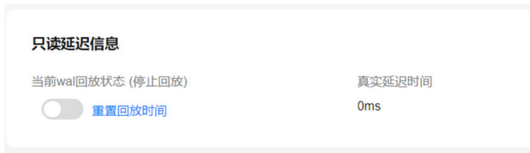
图 3-68 回放完成
