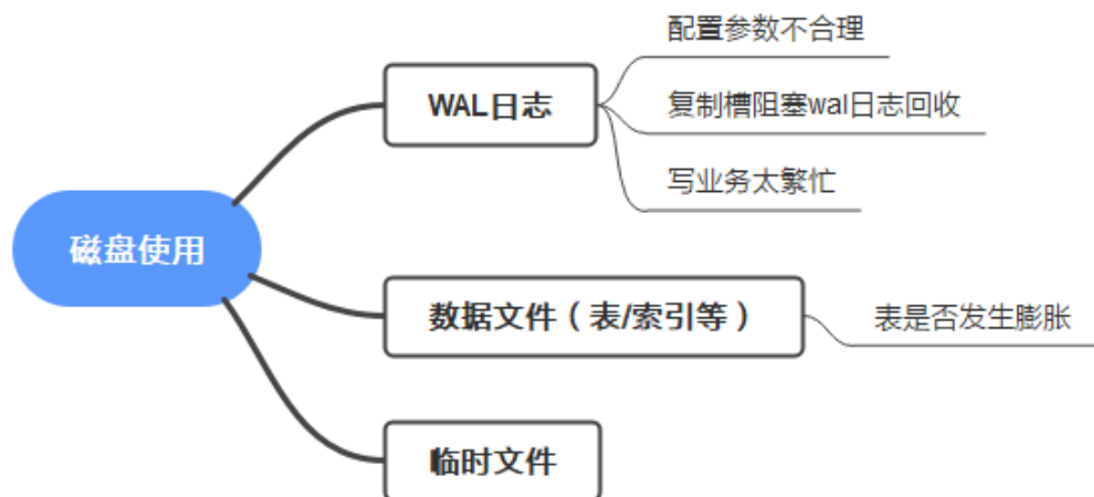
图 3-41 排查思路
