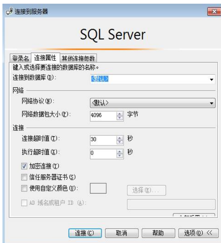
图 4-16 连接属性
