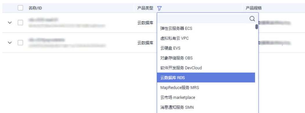
图 1-224 筛选服务
