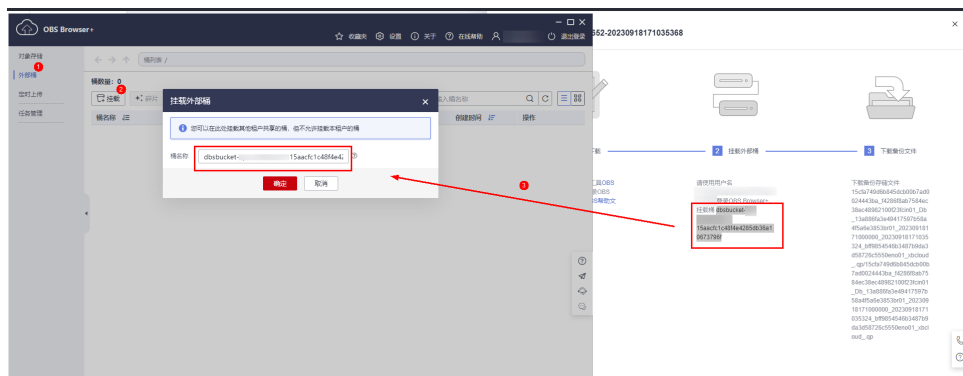
图 4-43 挂载外部桶
