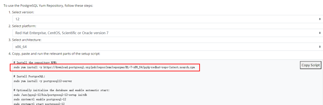
图 3-23 安装客户端
