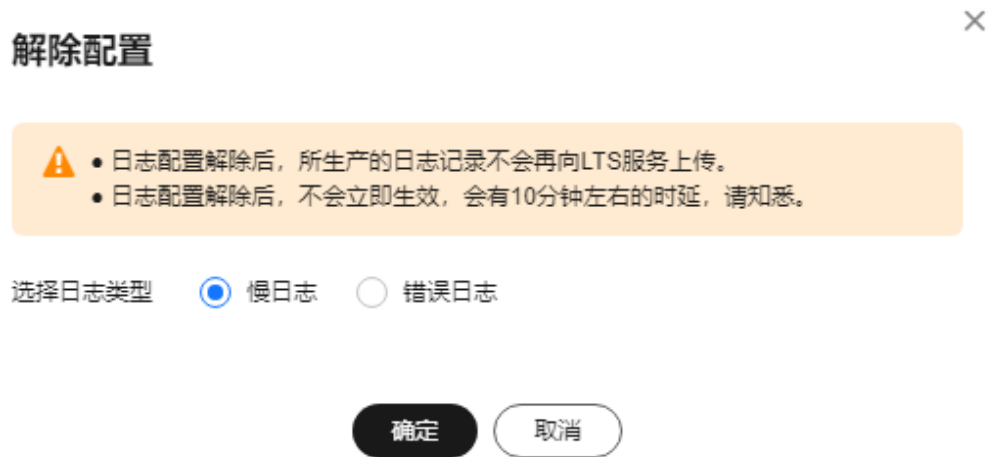
图 3-130 解除配置
