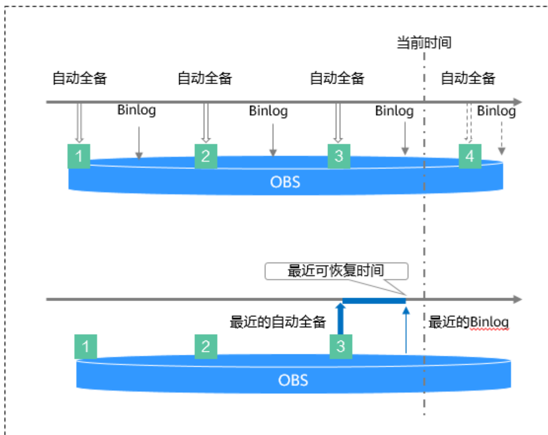
图 1-67 备份原理
