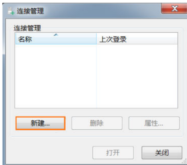
图 1-26 连接管理
