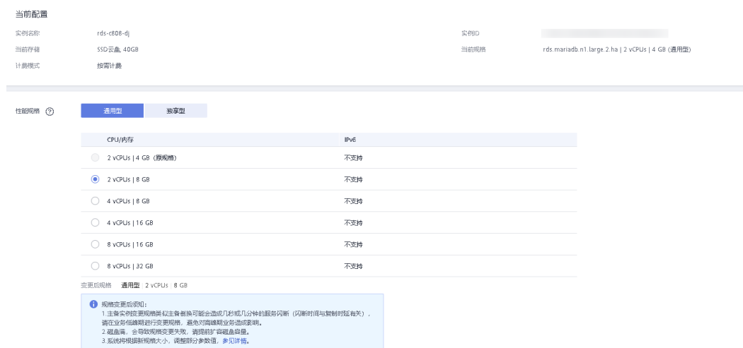
图 2-14 规格变更
