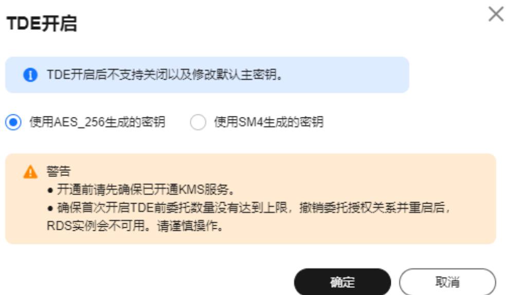
图 1-183 TDE 开启
