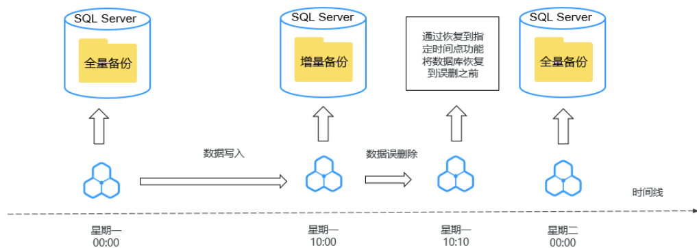
图 4-38 备份原理
