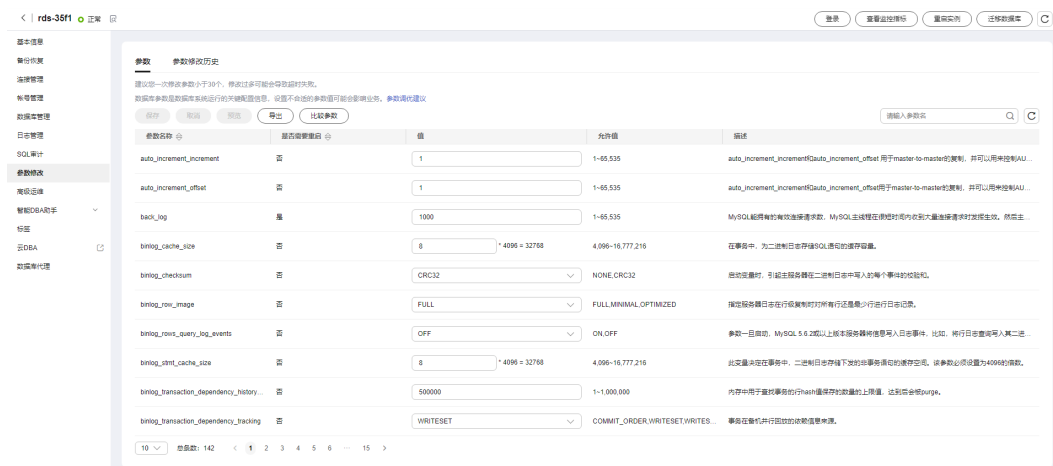
图 1-189 参数修改
