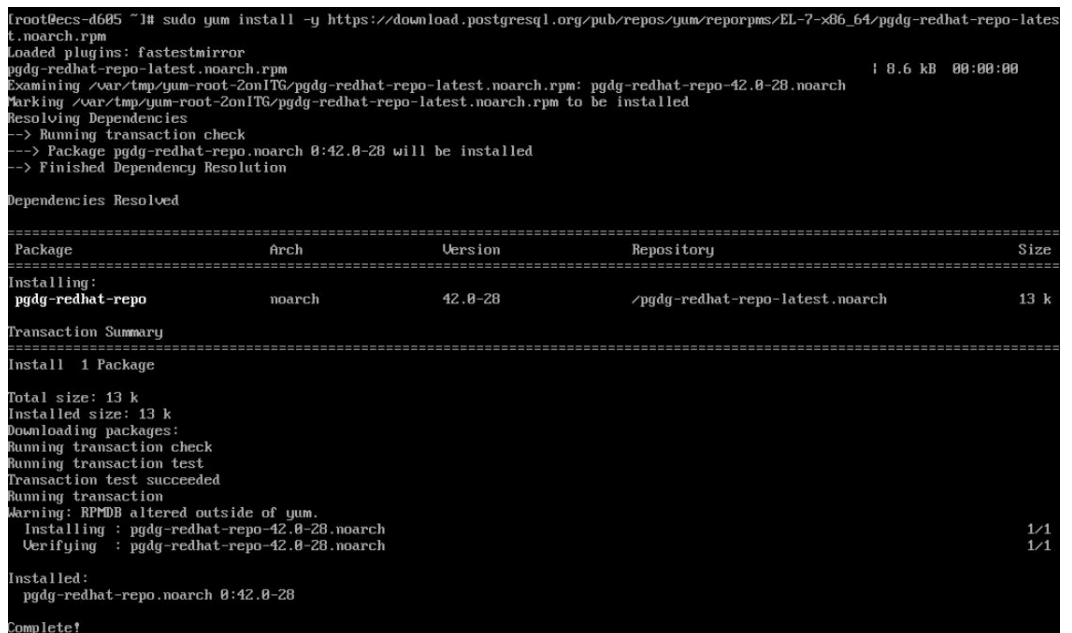
图 3-10 安装 rpm 包
