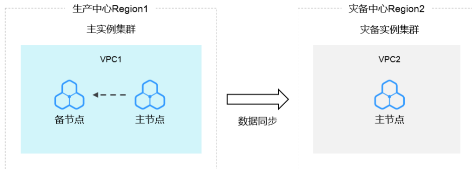
图 3-72 拓扑图
