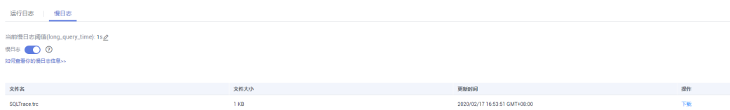
图 4-101 慢日志
