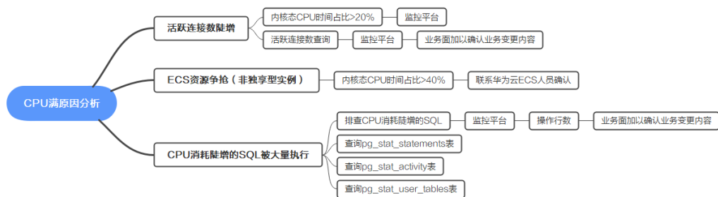
图 3-35 排查思路
