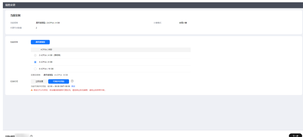
图 1-133 规格变更
