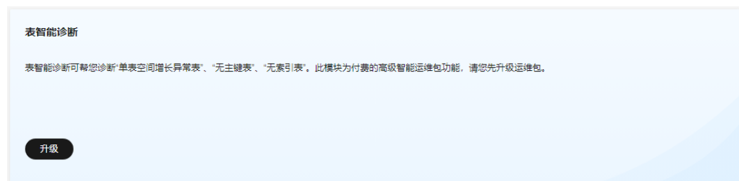
图 1-146 表智能诊断
