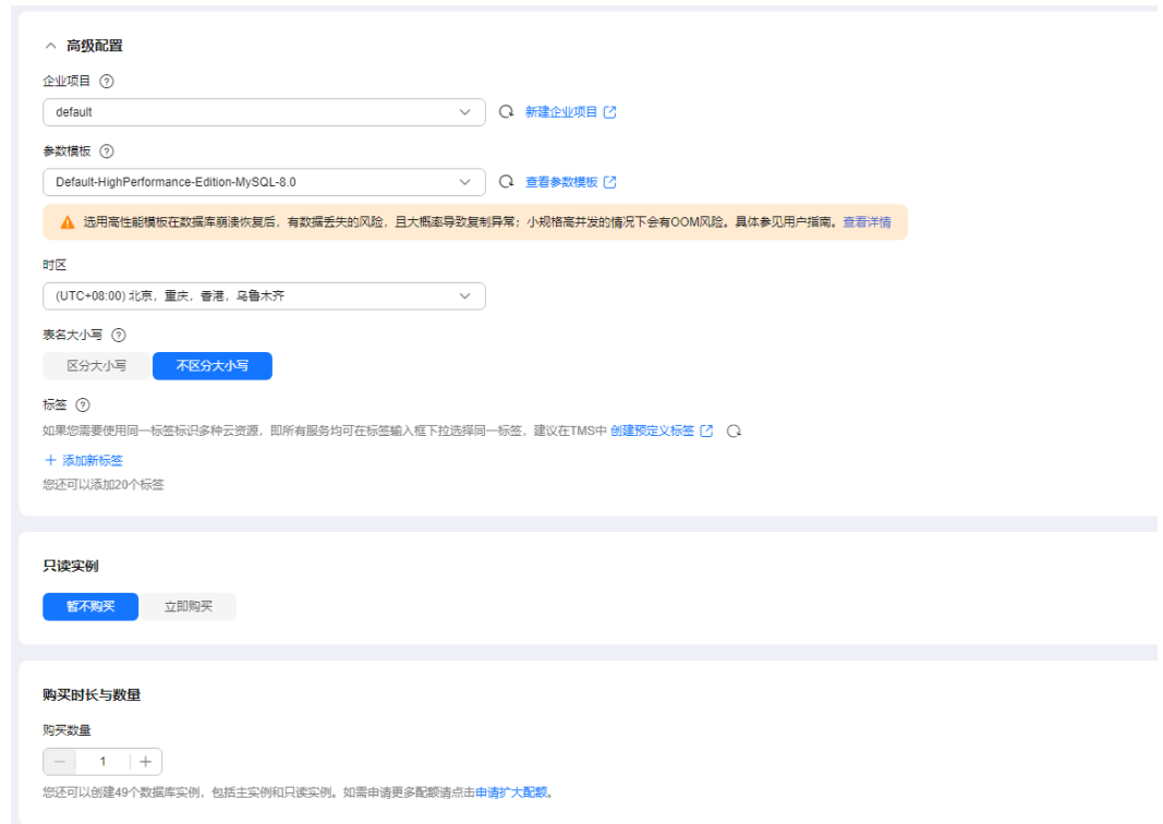
图 1-6 高级配置
