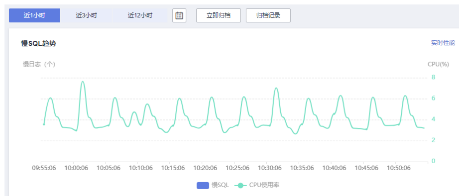
图 2-74 慢 SQL 趋势
