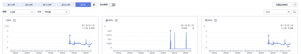
图 3-39 查看 IOPS
