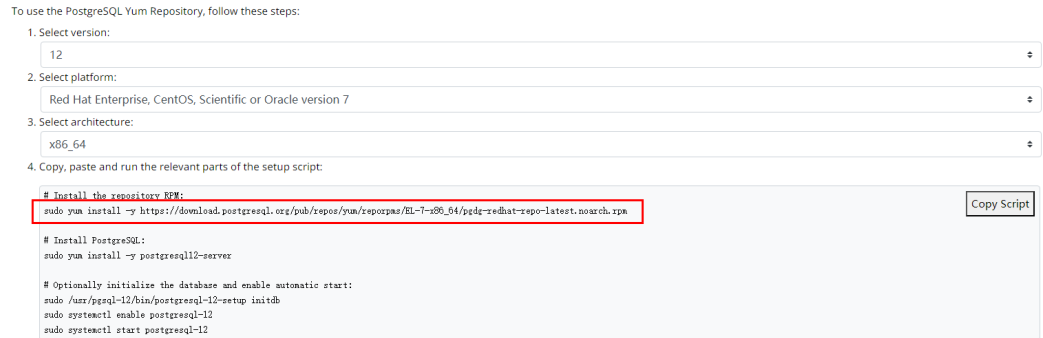
图 3-9 安装客户端
