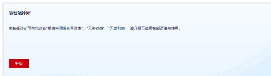
图 2-64 表智能诊断
