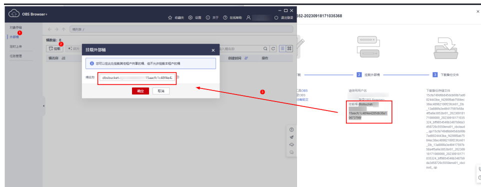
图 1-77 挂载外部桶
