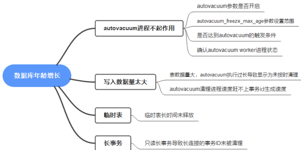
图 3-37 排查思路
