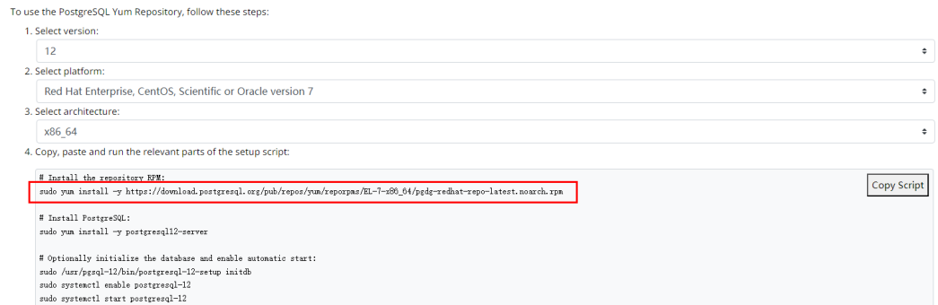
图 3-19 安装客户端
