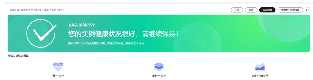
图 1-157 诊断日报
