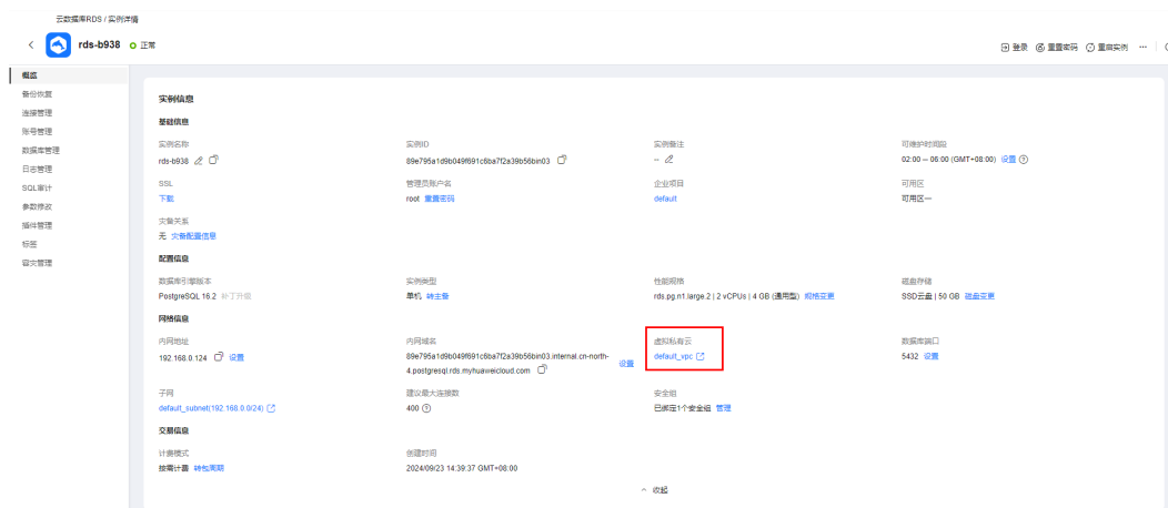
图 3-5 PostgreSQL 概览
