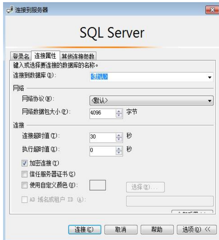
图 4-11 连接属性
