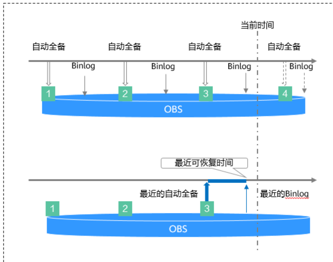
图 1-67 备份原理
