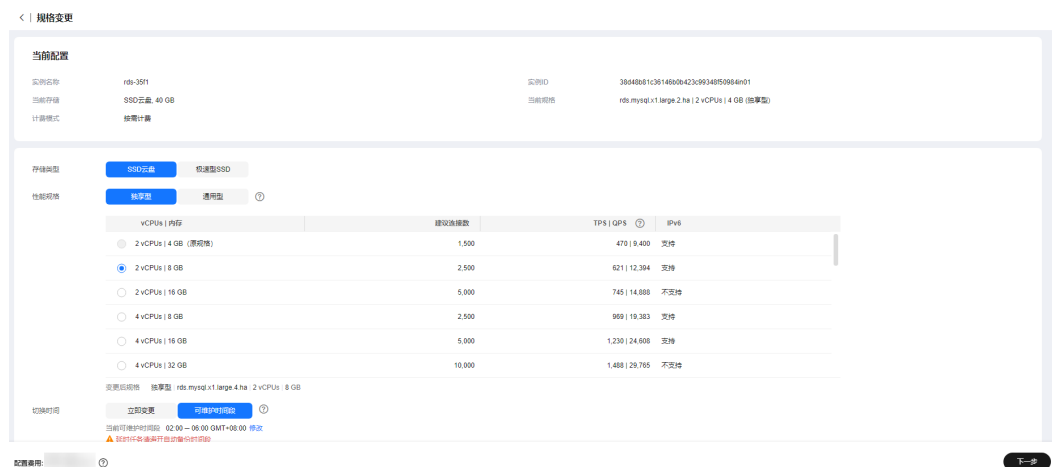
图 1-60 规格变更
