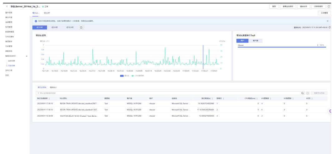
图 4-111 慢 SQL
