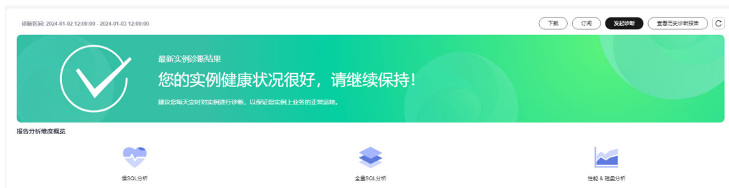
图 1-154 诊断日报
