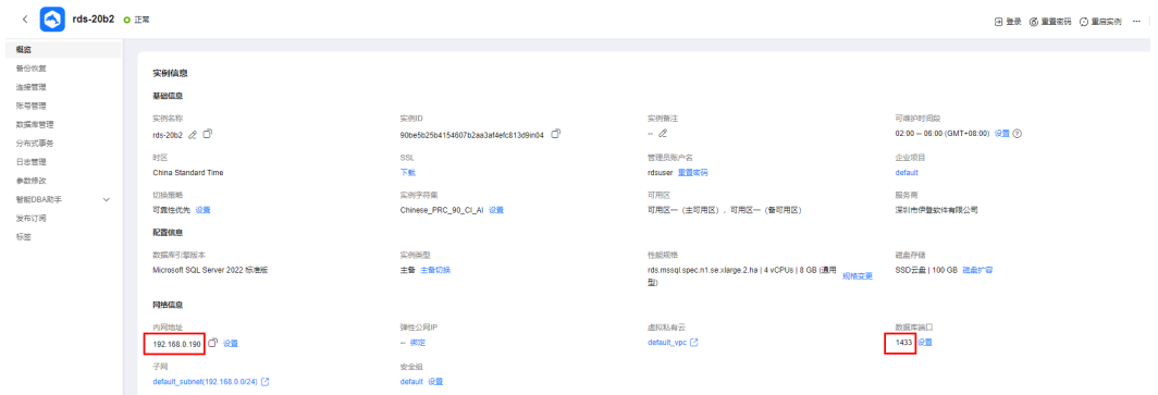
图 4-6 连接信息
