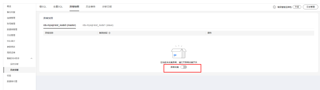
图 1-160 异常快照
