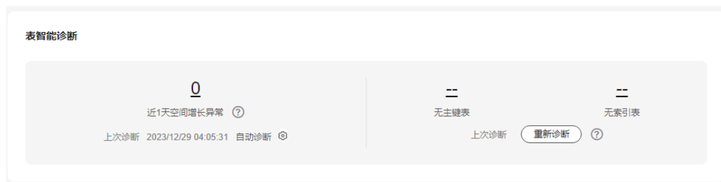
图 1-147 表诊断结果
