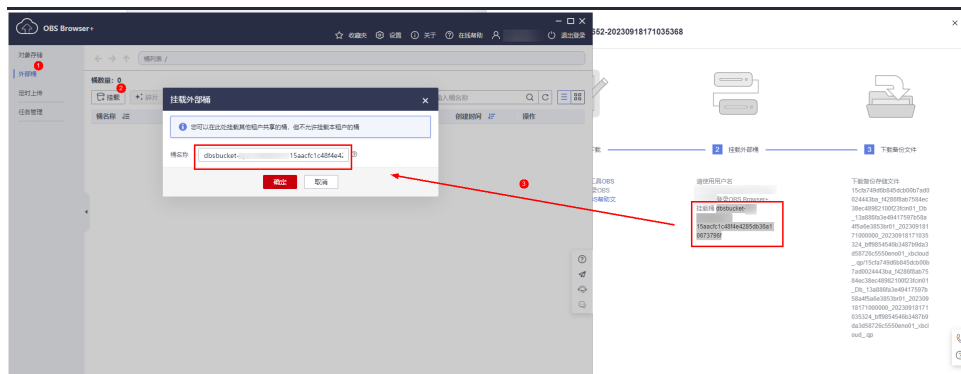
图 3-78 挂载外部桶
