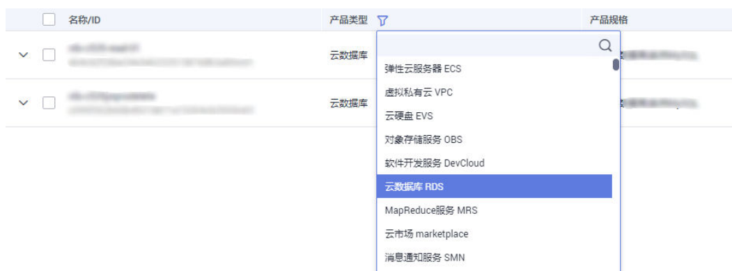
图 4-125 筛选服务
