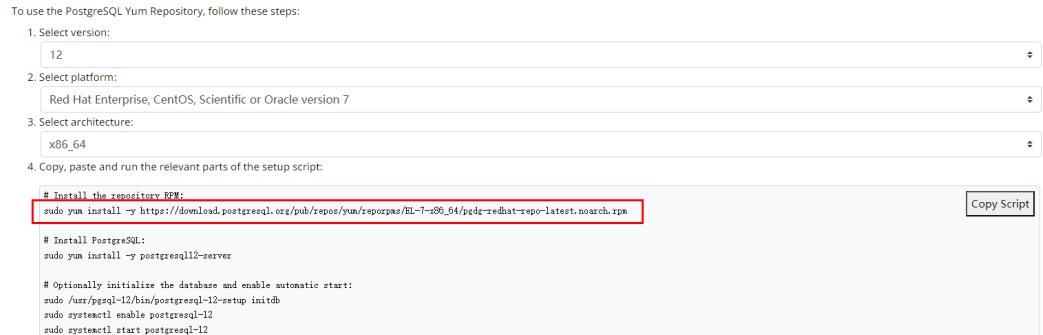
图 3-9 安装客户端
