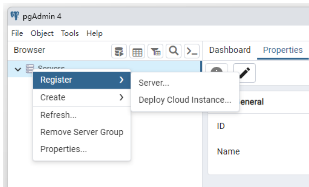
图 3-27 Servers
