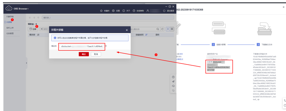
图 4-43 挂载外部桶
