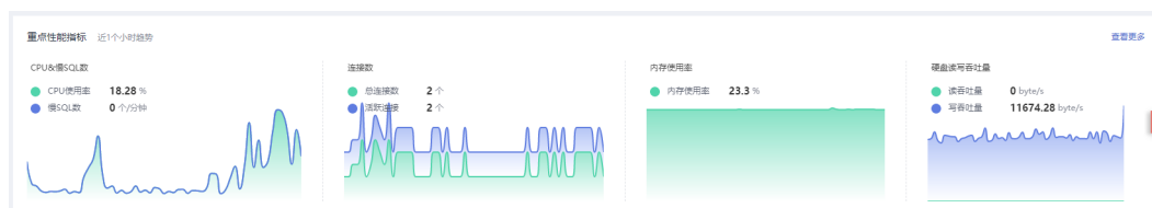
图 1-142 性能指标
