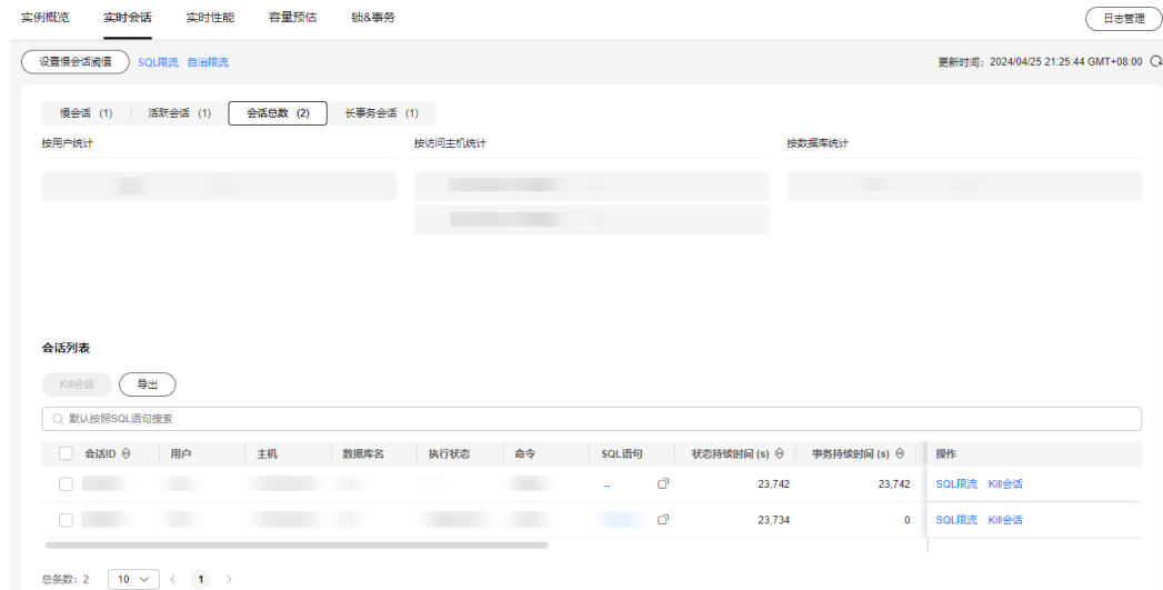
图 1-143 实时会话
