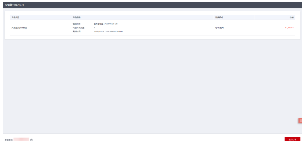
图 1-134 转包周期
