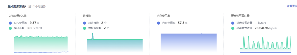
图 2-59 性能指标
