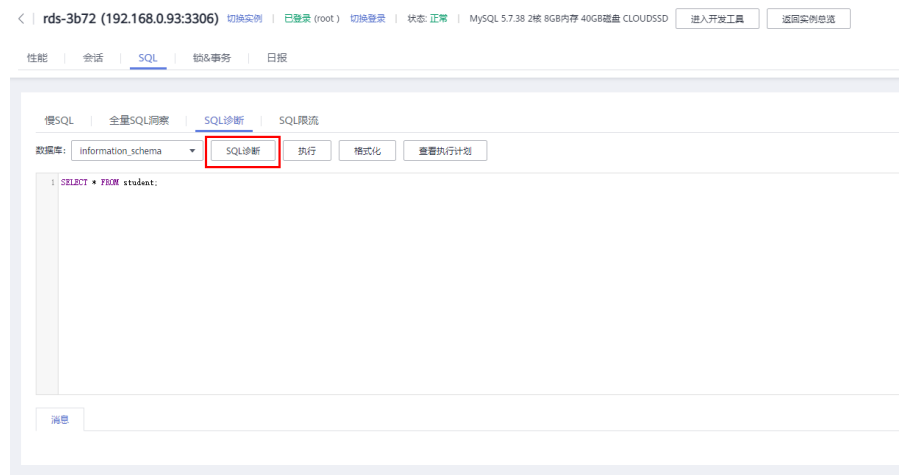
图 1-171 SQL 诊断
