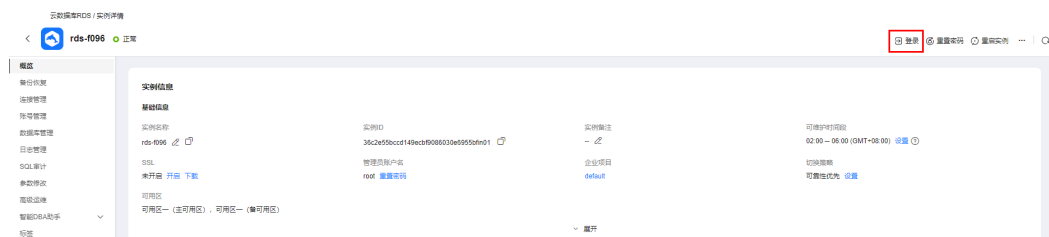
图 1-9 登录实例
