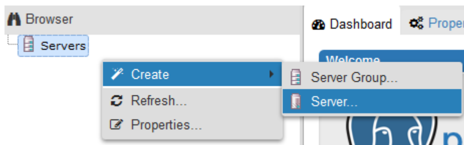
图 3-102 创建
