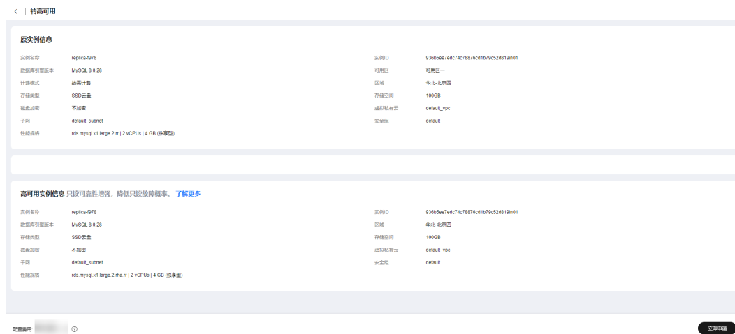
图 1-101 转高可用
