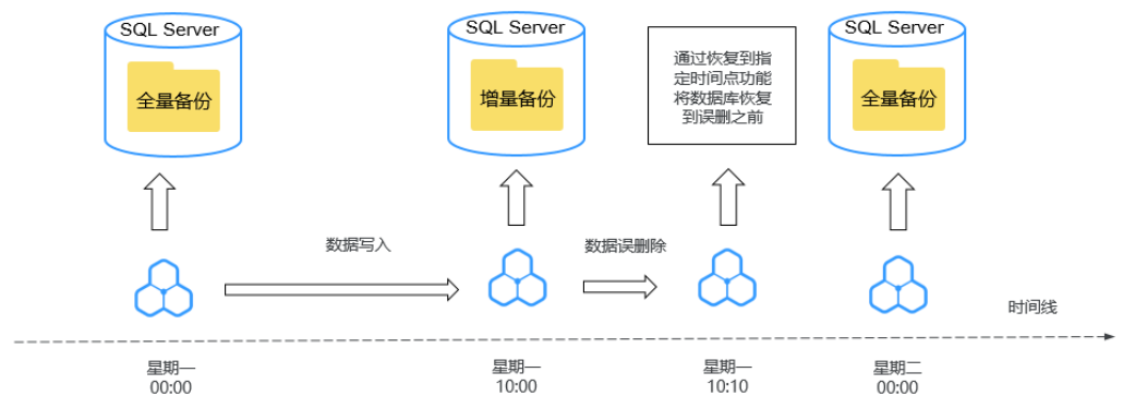
图 4-38 备份原理
