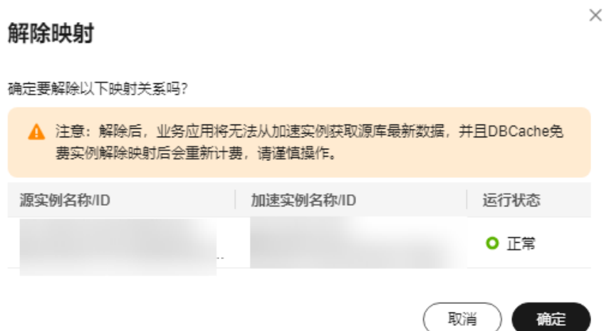
图 1-240 解除映射
