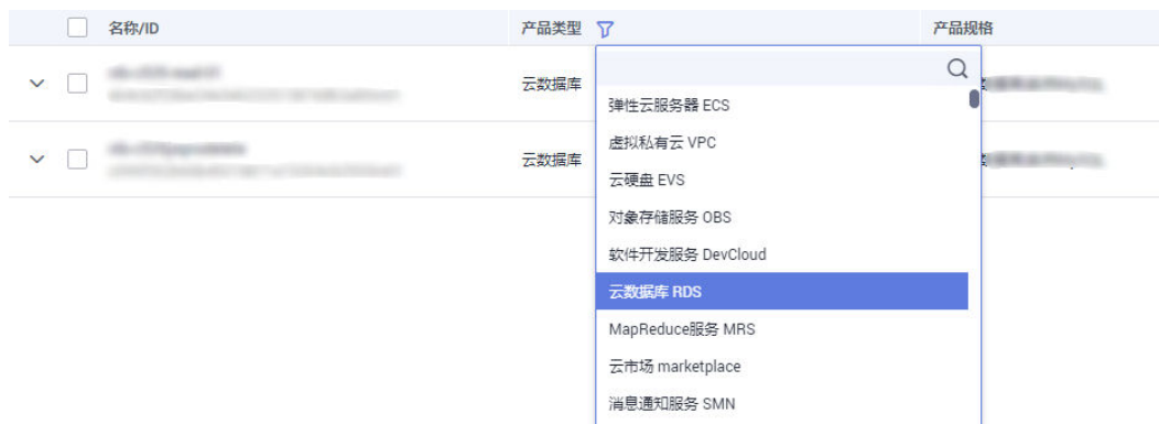
图 3-137 筛选服务
