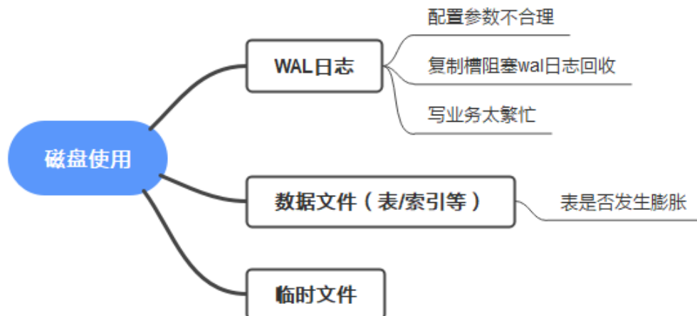
图 3-41 排查思路
