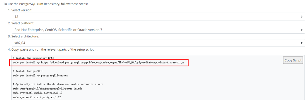
图 3-19 安装客户端
