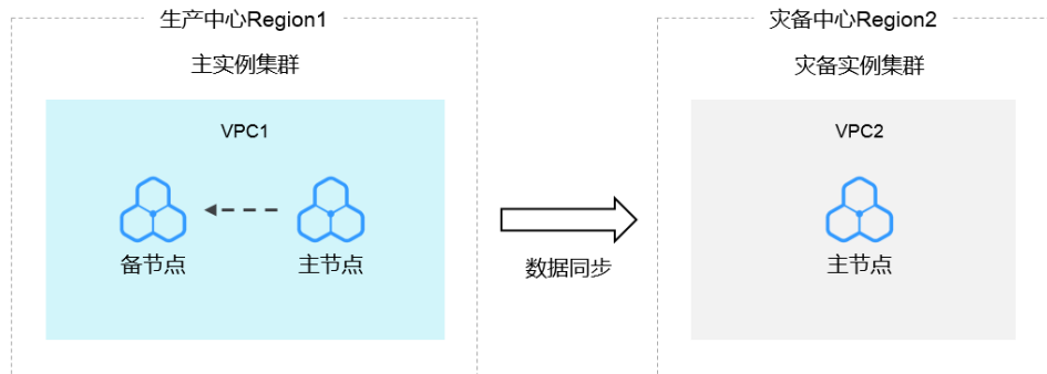
图 3-72 拓扑图
