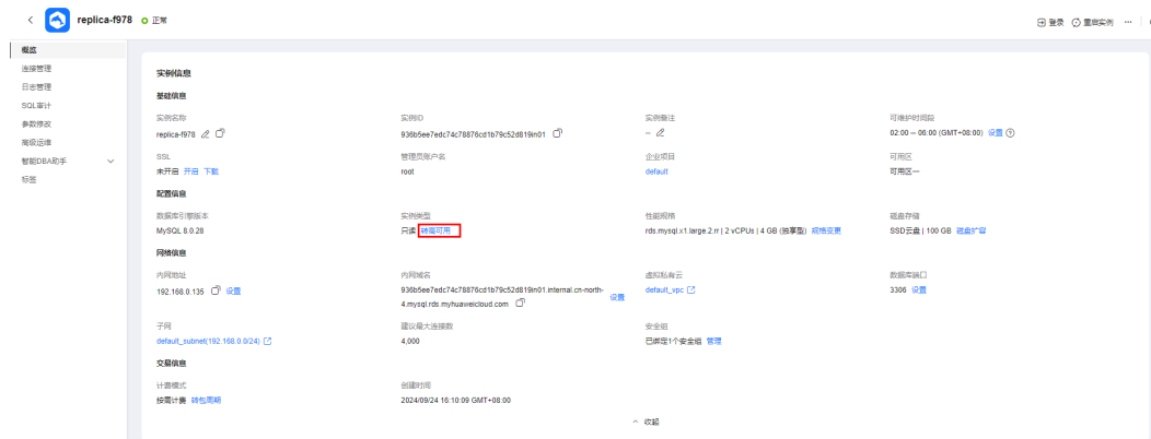
图 1-100 数据库信息
