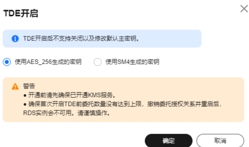
图 1-180 TDE 开启
