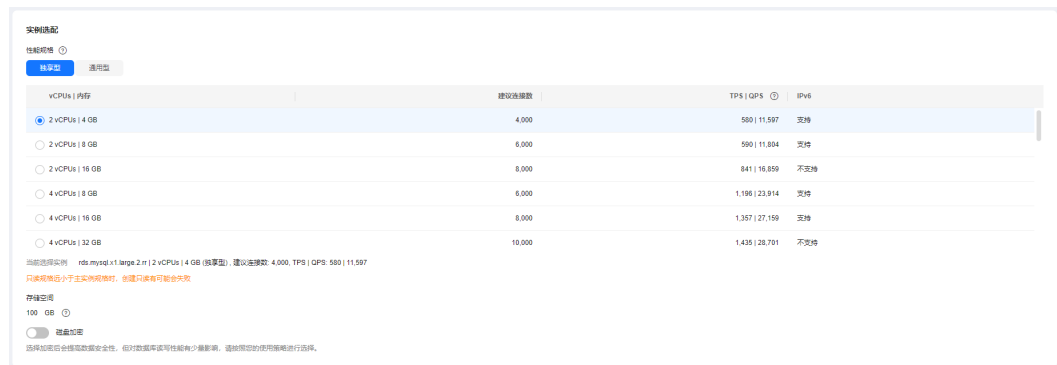
图 1-98 实例选配
