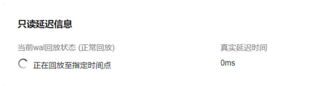
图 3-67 回放中
