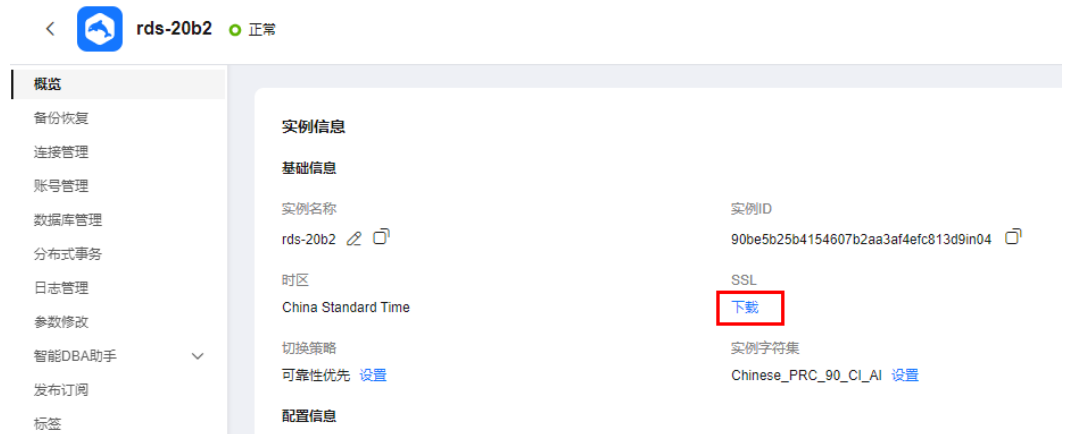
图 4-14 下载证书
