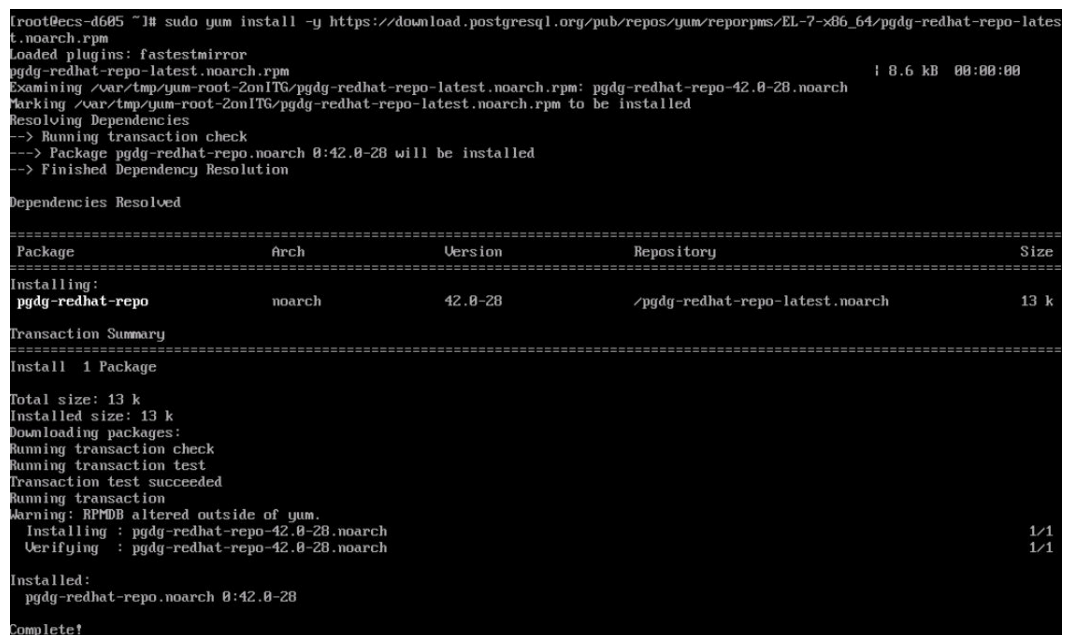
图 3-10 安装 rpm 包
