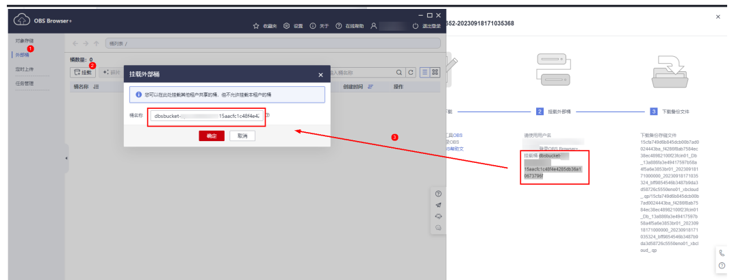
图 2-23 挂载外部桶
