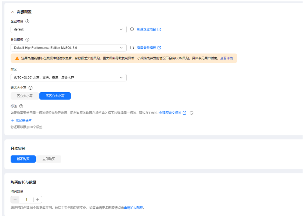
图 1-6 高级配置
