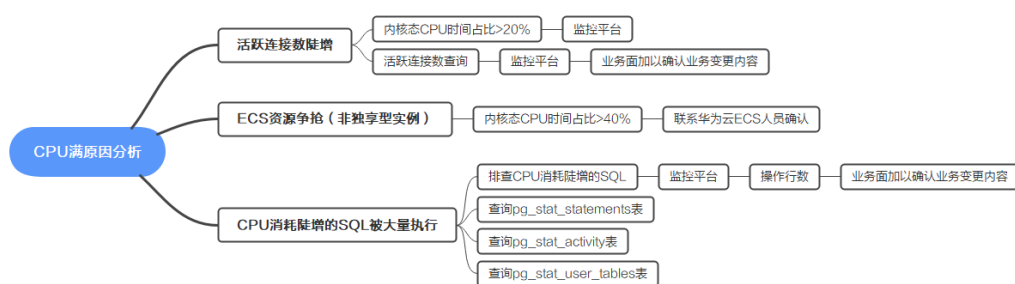
图 3-35 排查思路
