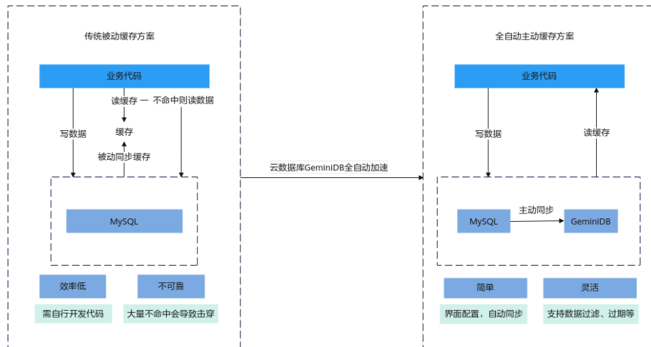
图 1-226 原理图
