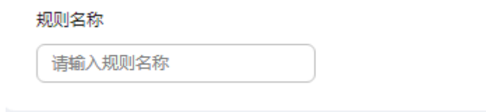
图 1-228 规则名称
