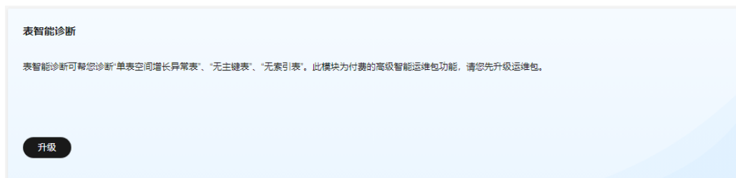
图 1-145 表智能诊断
