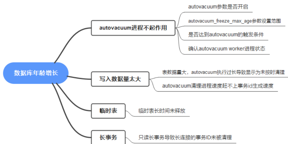
图 3-37 排查思路
