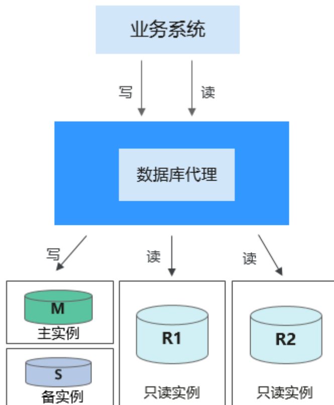
图 1-102 单个数据库代理原理图
