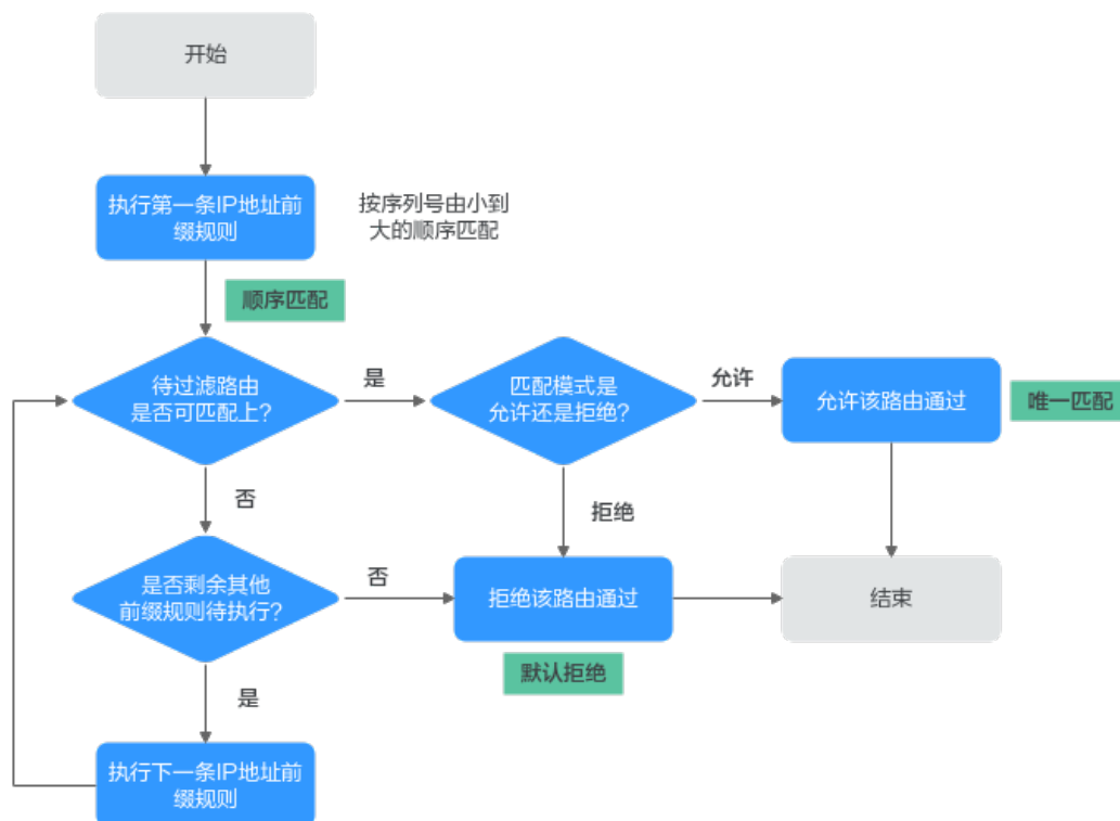
图 2-1 IP 地址前缀匹配规则
