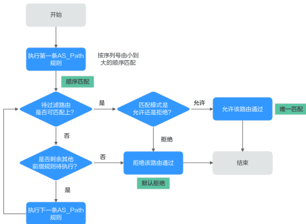
图 3-2 AS_Path 匹配规则
