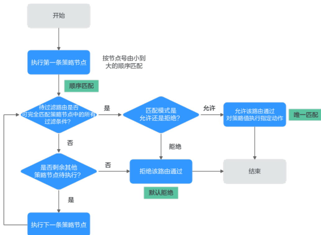
图 1-1 路由策略匹配规则
