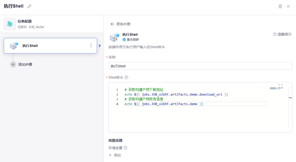
图 14-4 执行 Shell
