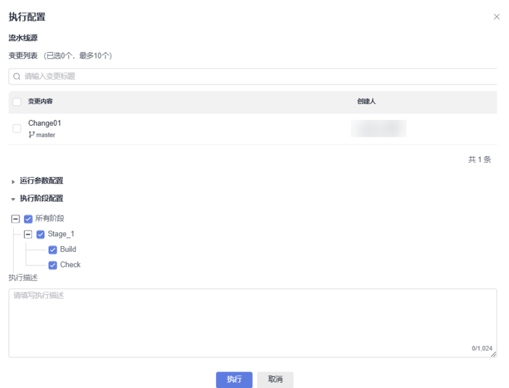
图 10-5 配置变更流水线执行信息
