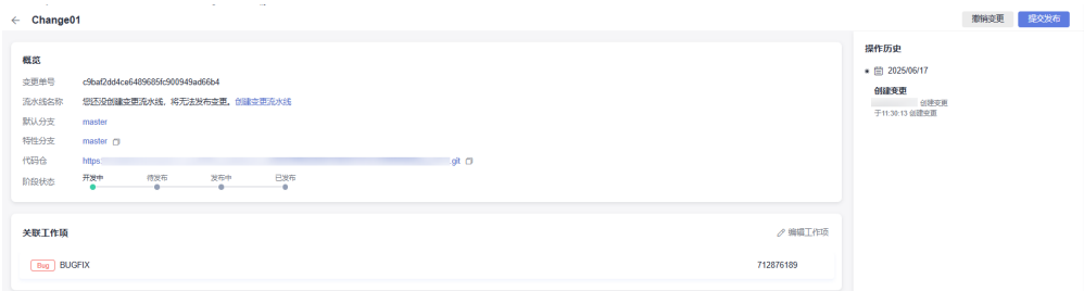
图 10-4 变更详情
