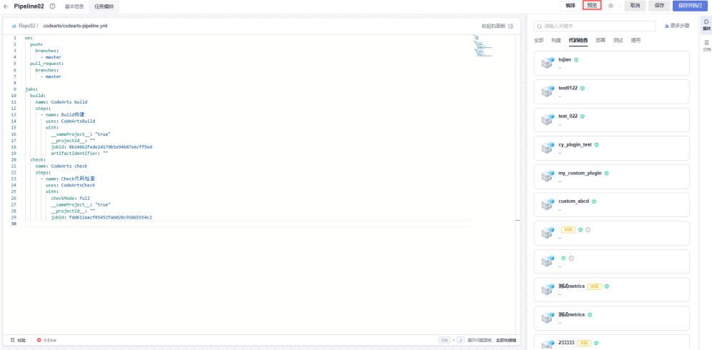
图 4-5 任务编排
