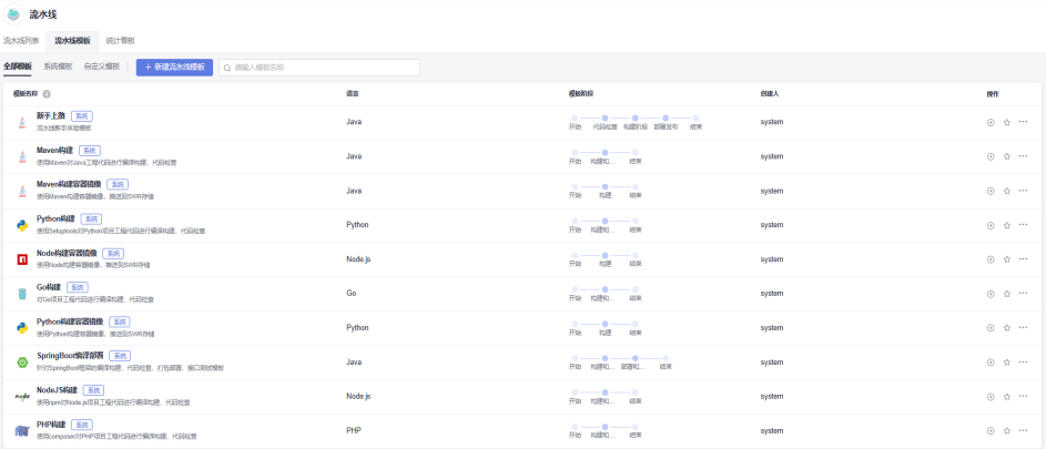
图 4-2 流水线模板
