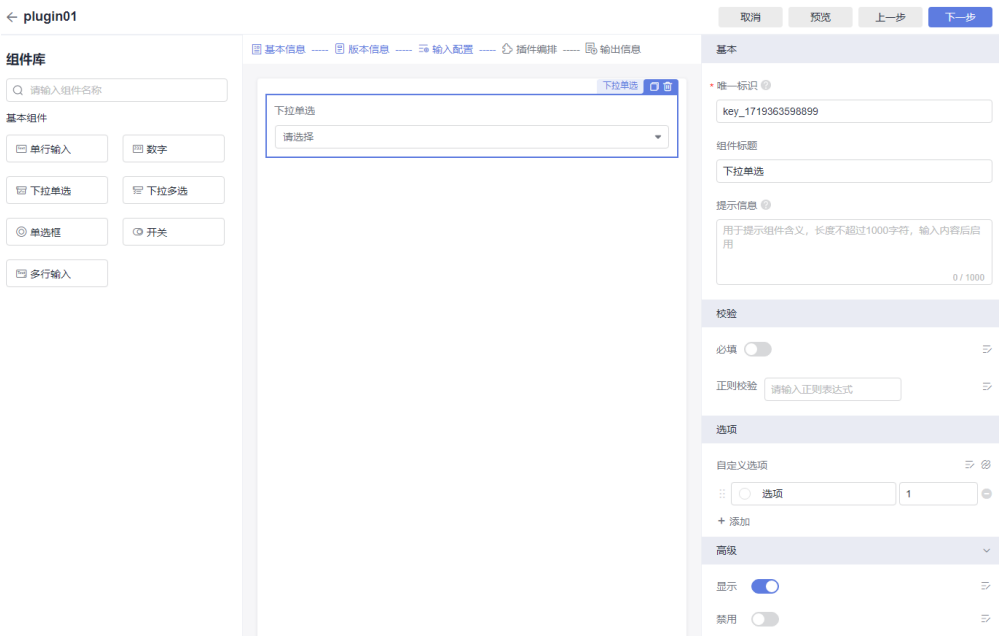
图 11-1 编排组件
