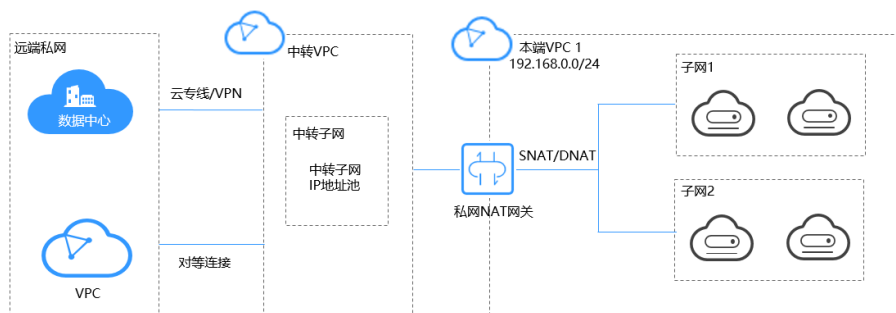
图 3-1 私网 NAT 网关
