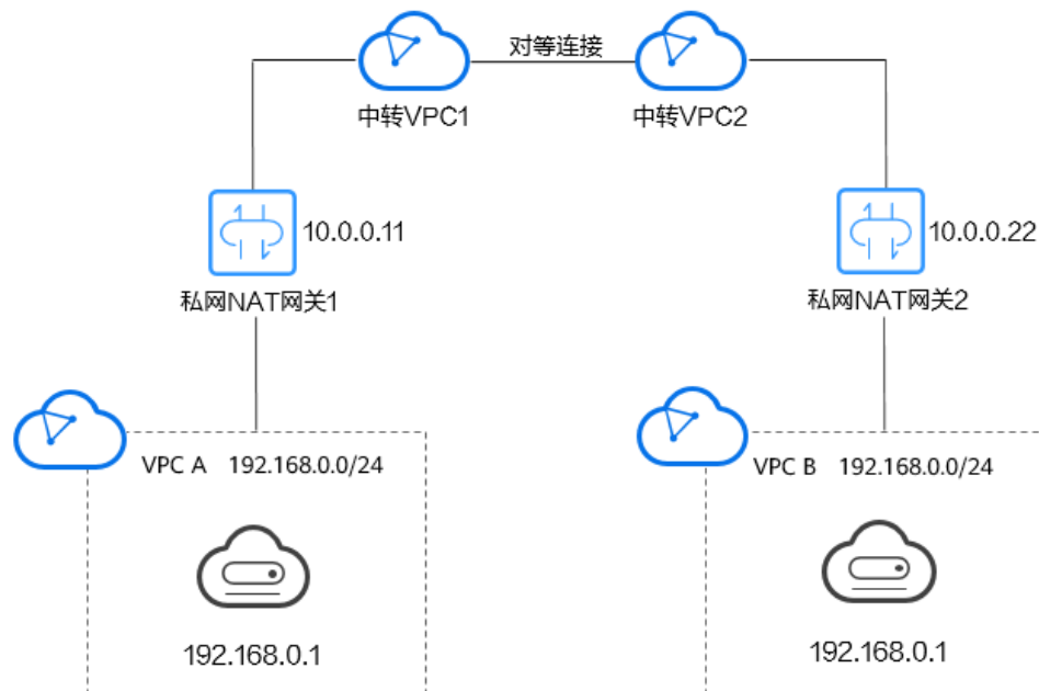
图 3-2 重叠网段 VPC 间互通
