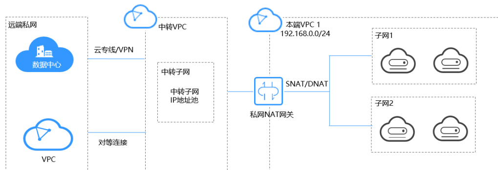
图 2-1 私网 NAT 网关
